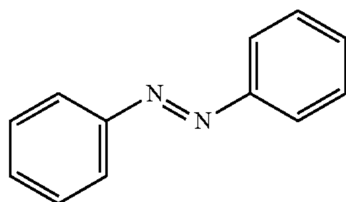
(E)-diphenyldiazene, (E)-Azobenzene
