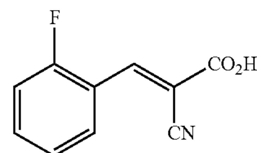
(E)-2-Cyano-3-(2-fluorophenyl)acrylic Acid (JXL030)
