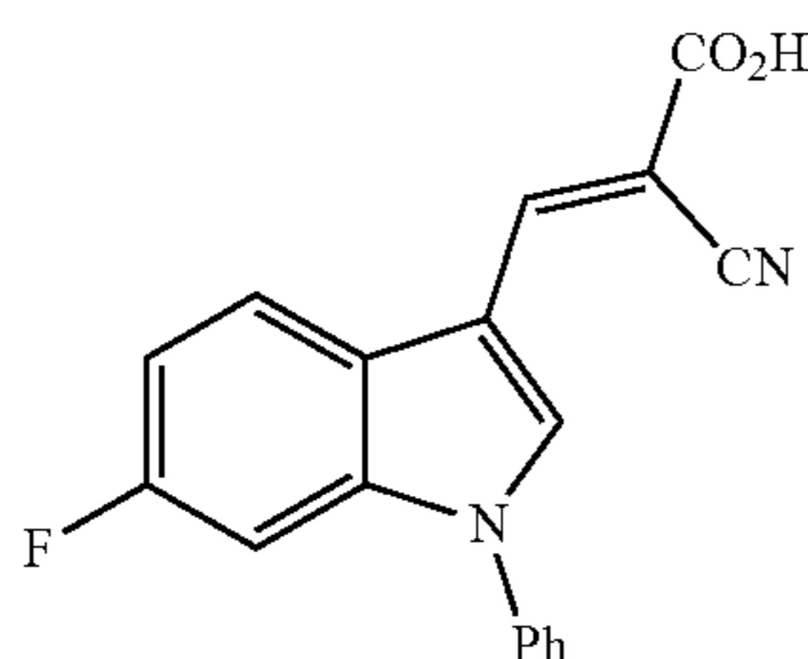
(E)-2-Cyano-3-(6-fluoro-1-phenyl-1H-indol-3-yl) acrylic Acid (JXL027)
