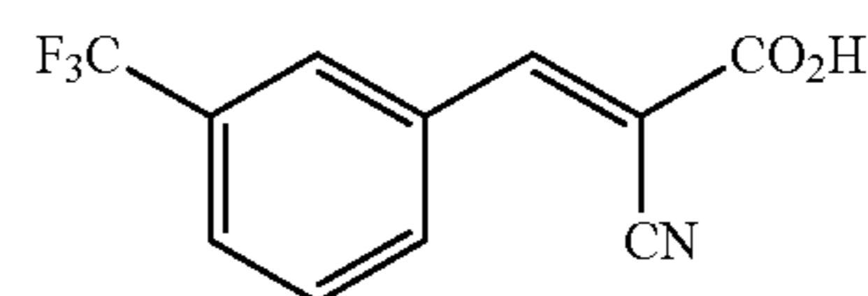
(E)-2-cyano-3-(3-(trifluoromethyl)phenyl)acrylic Acid (JXL033)
