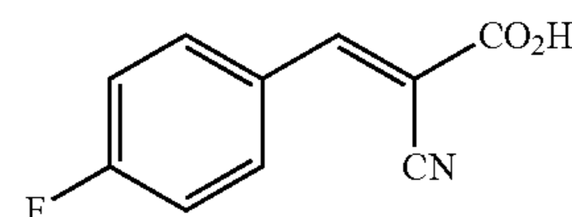
(E)-2-Cyano-3-(4-fluorophenyl)acrylic Acid (JXL032)
