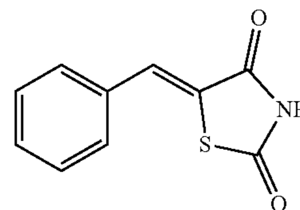
(Z)-5-Benzylidenethiazolidine-2,4-dione (JXL074)
