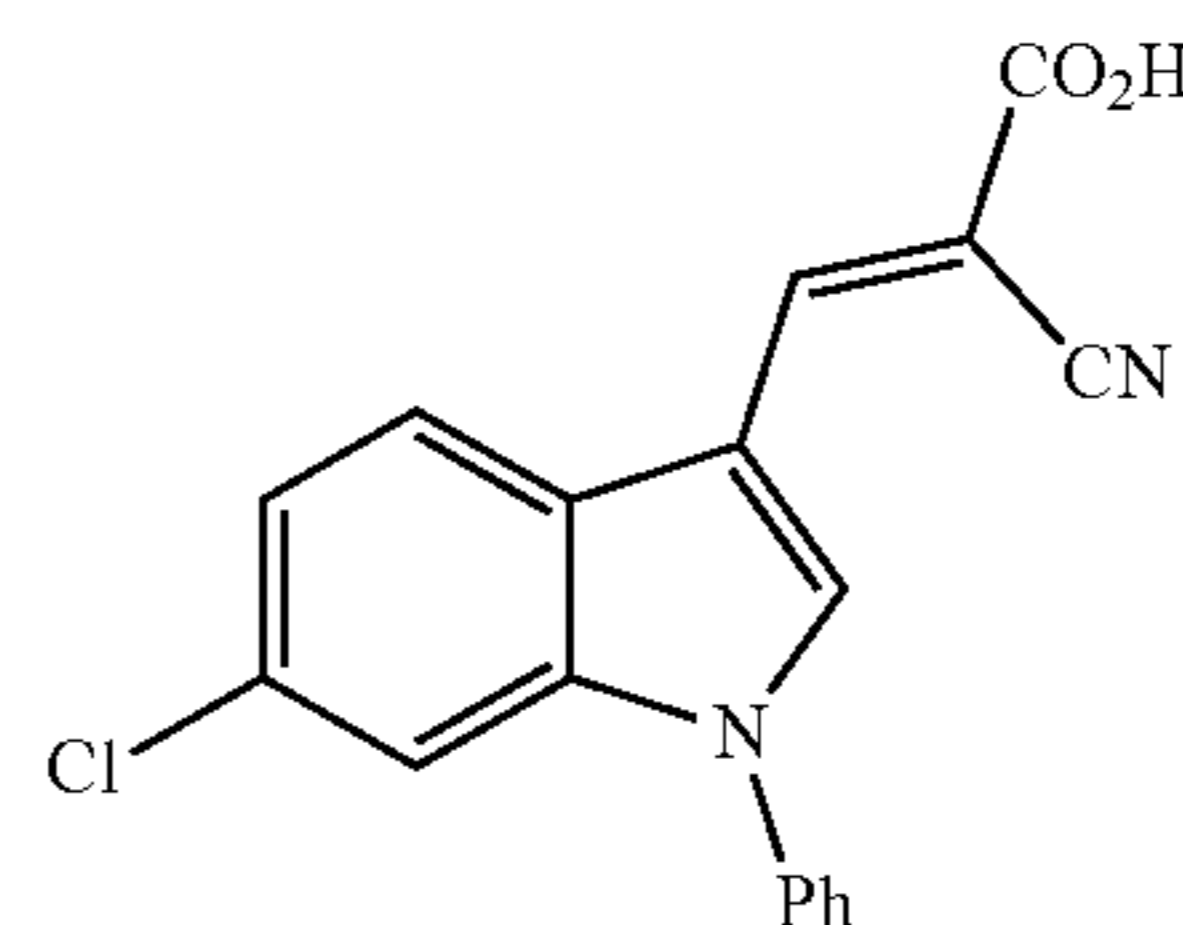
(E)-3-(6-Chloro-1-phenyl-1H-indol-3-yl)-2-cyanoacrylic Acid (JXL013)
