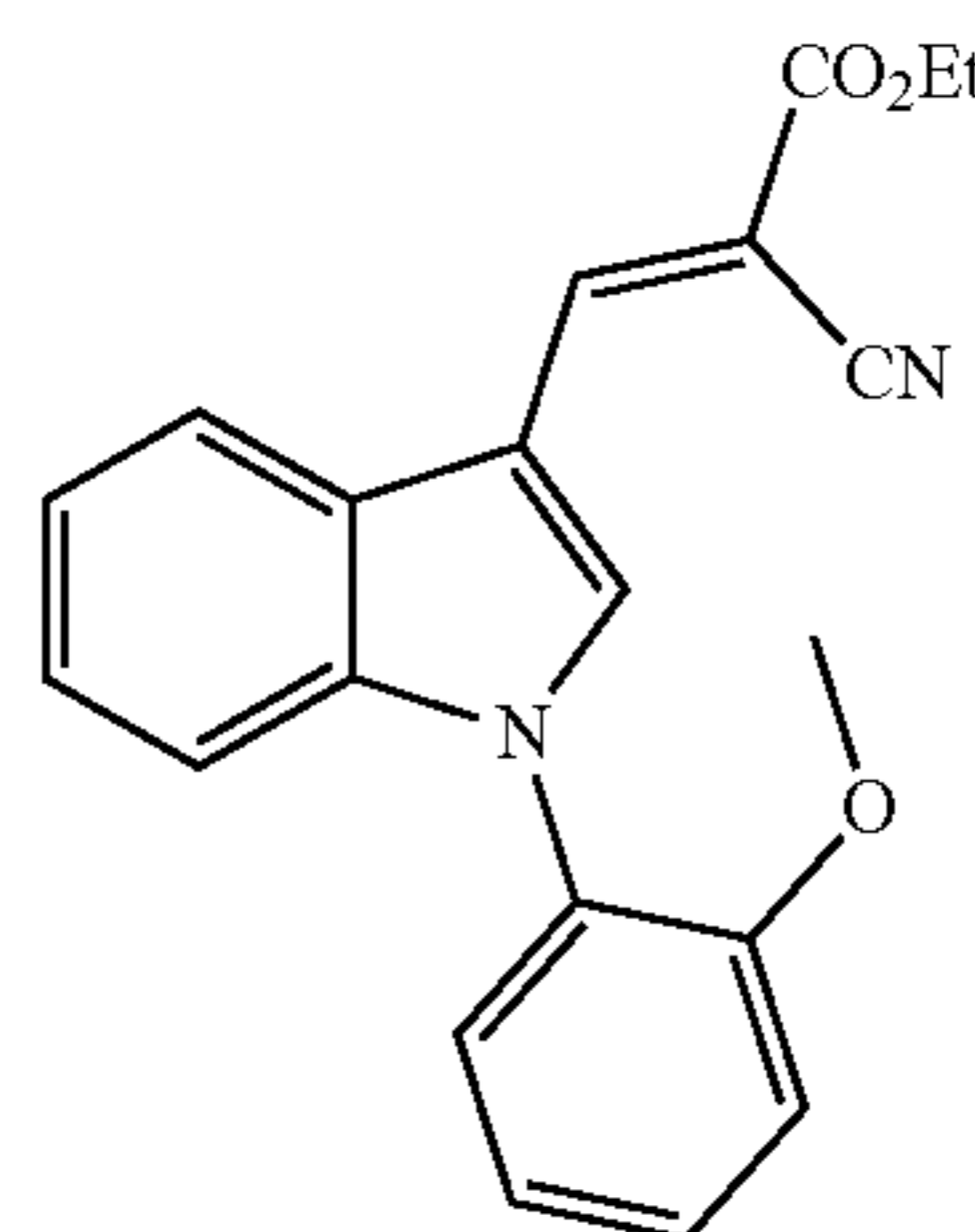
Ethyl (E)-2-cyano-3-(1-(2-methoxyphenyl)-1H-indol-3-yl)acrylate (JXL006)
