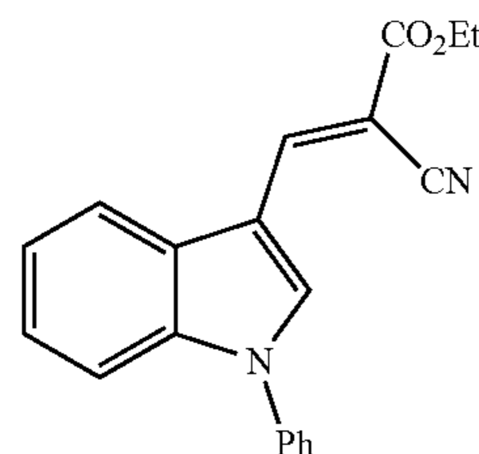
Ethyl (E)-2-cyano-3-(1-phenyl-1H-indol-3-yl)acrylate (JXL004)
