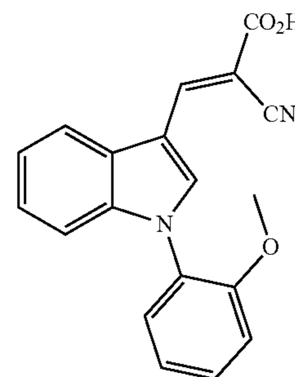
(E)-2-Cyano-3-(1-(2-methoxyphenyl)-1H-indol-3-yl)acrylic Acid (JXL014)
