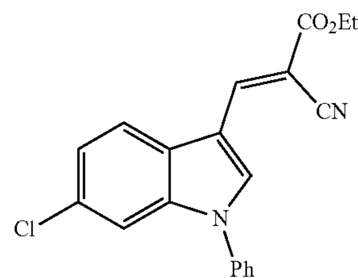
Ethyl (E)-3-(6-chloro-1-phenyl-1H-indol-3-yl)-2-cyanoacrylate (JXL005)
