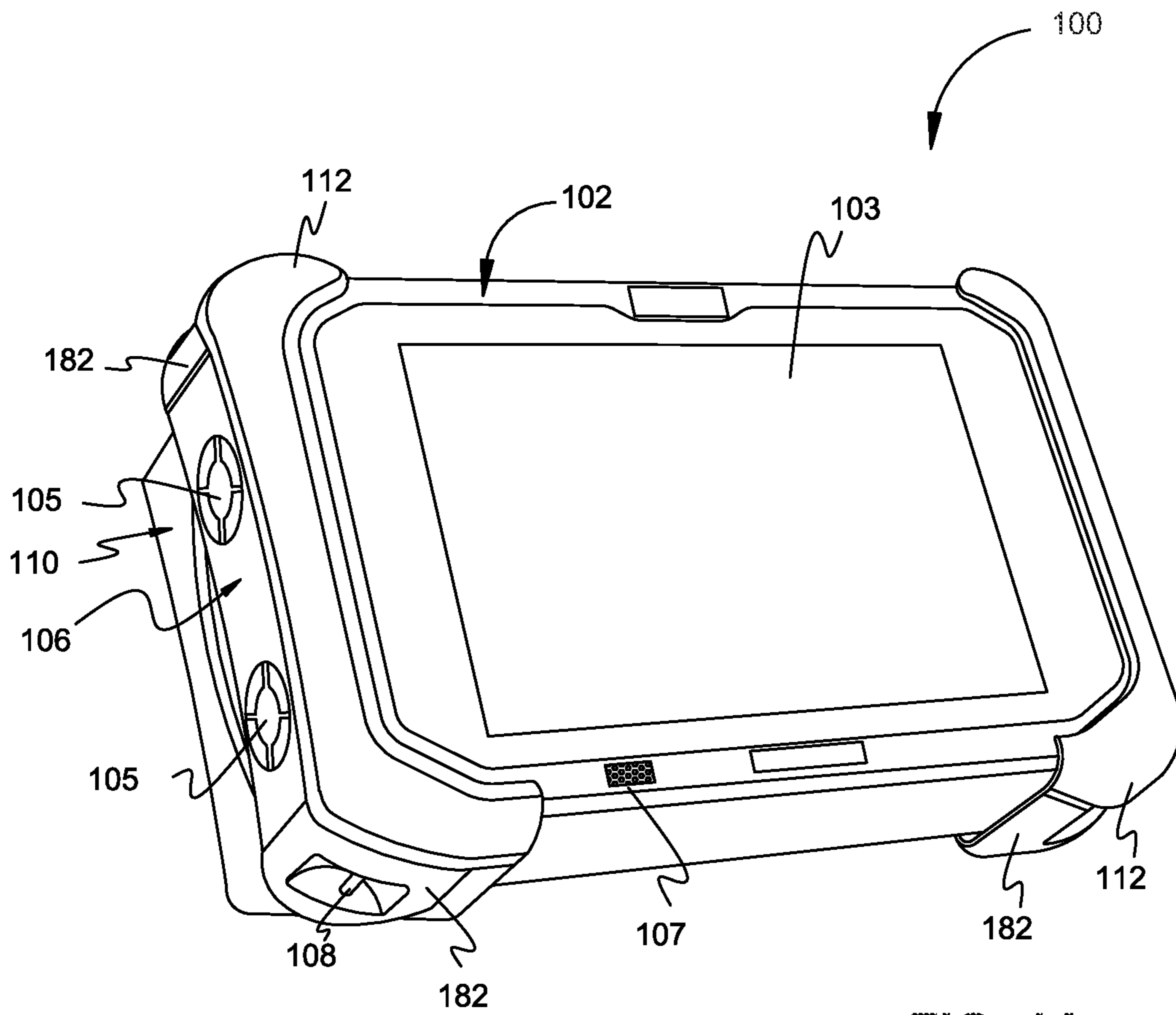
FIG. 1A
