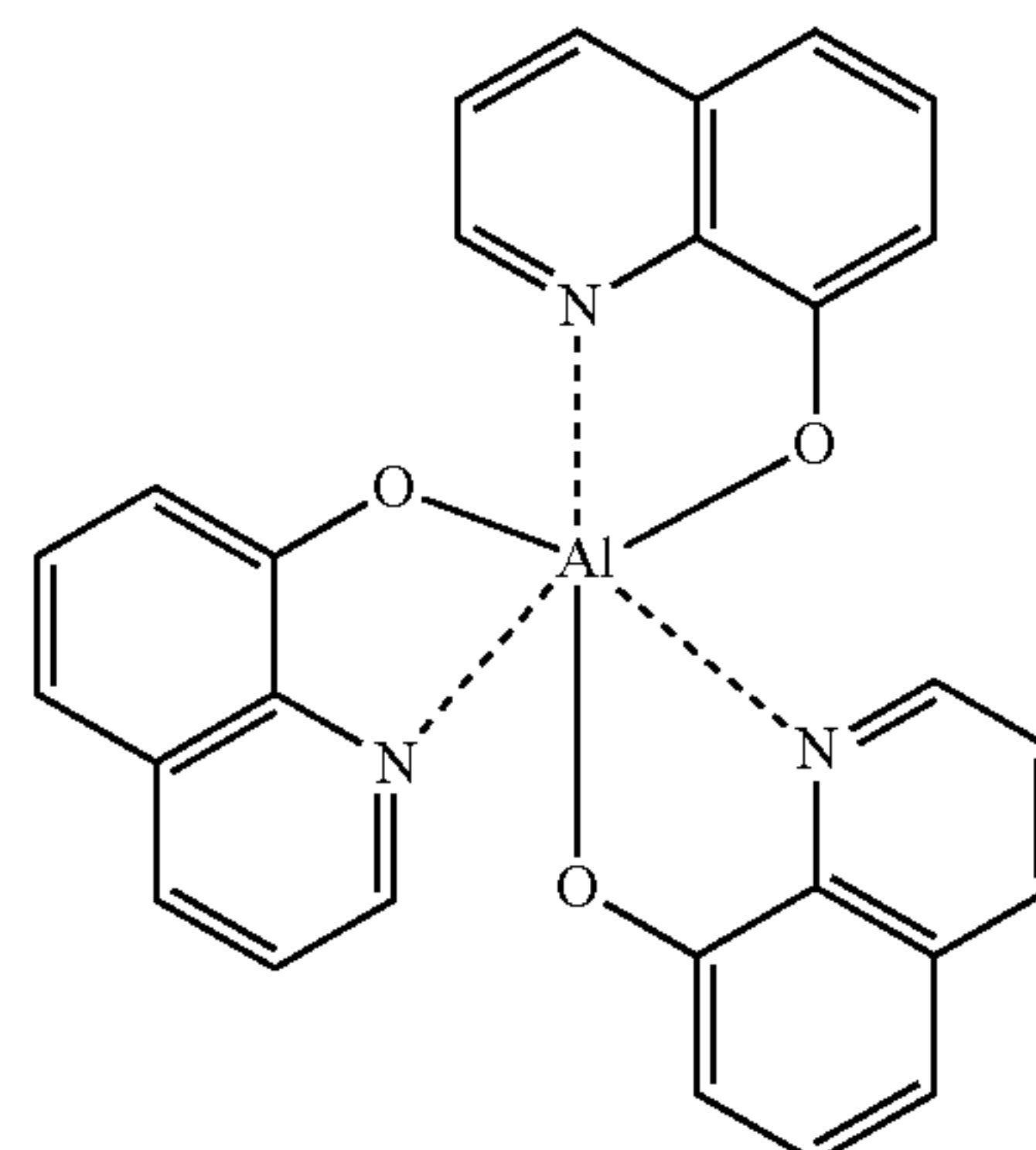
Alq 3
