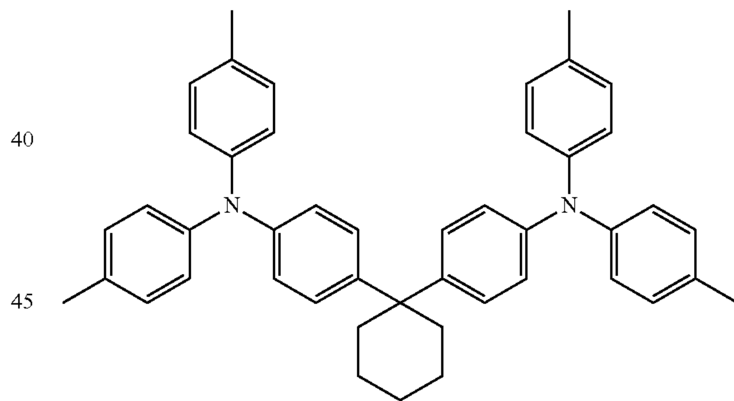
TAPC
