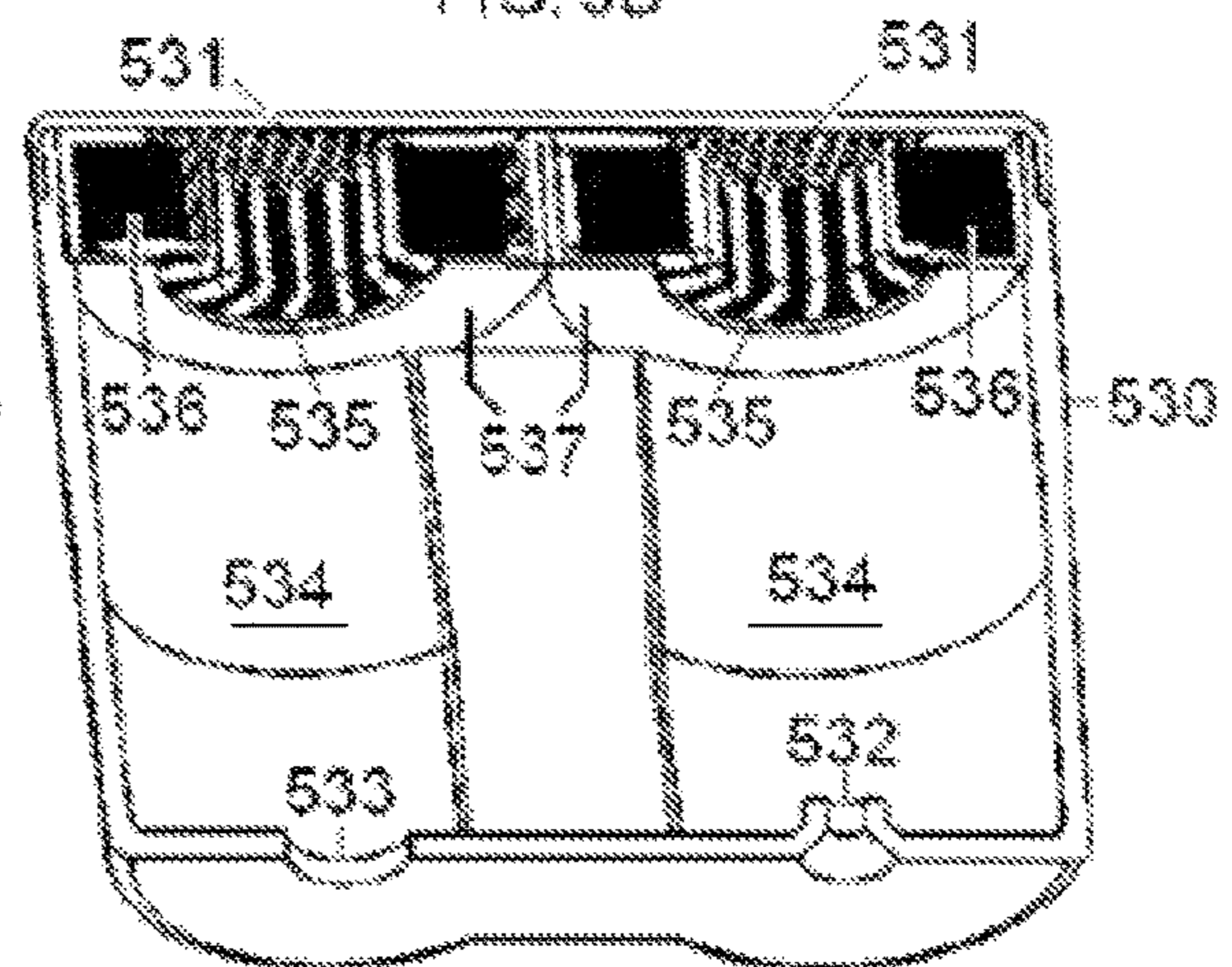
FIG. 5D
