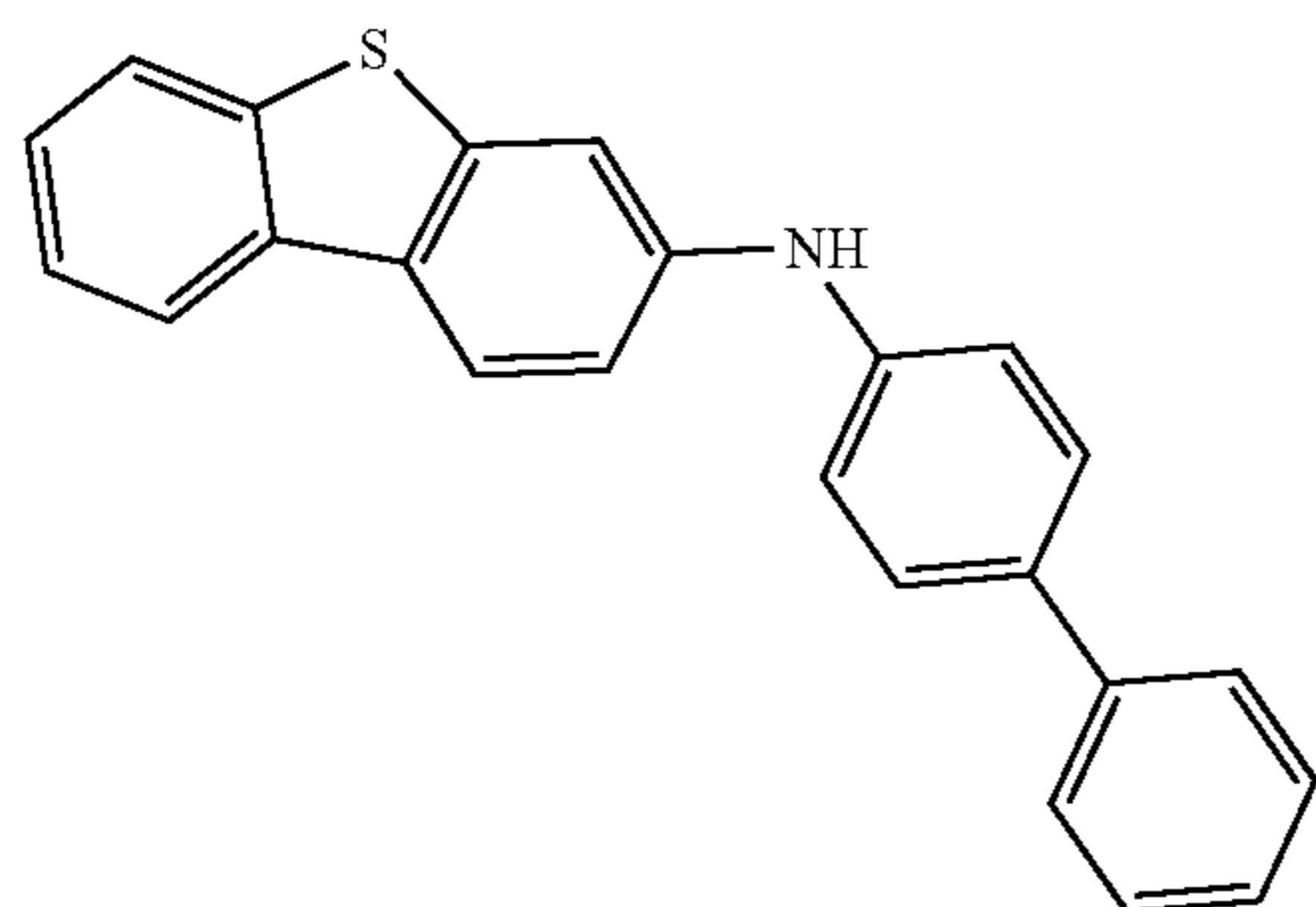
Intermediate31-2
