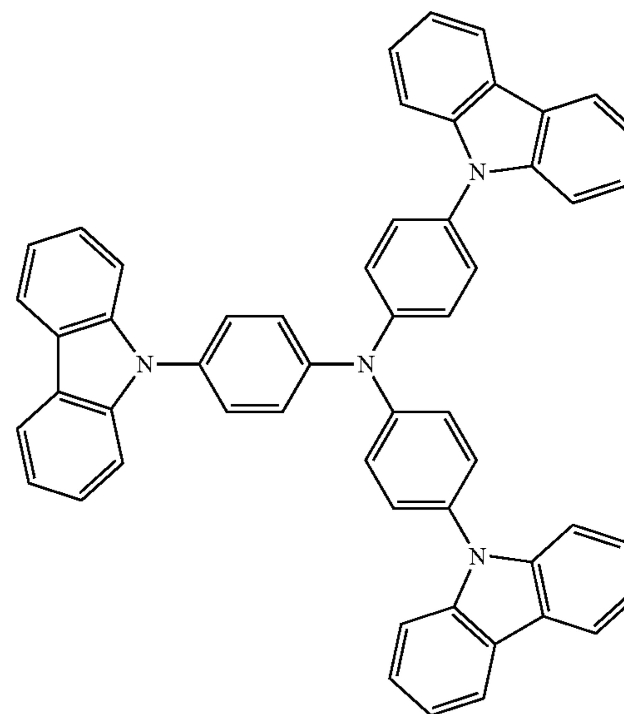
TCTA
