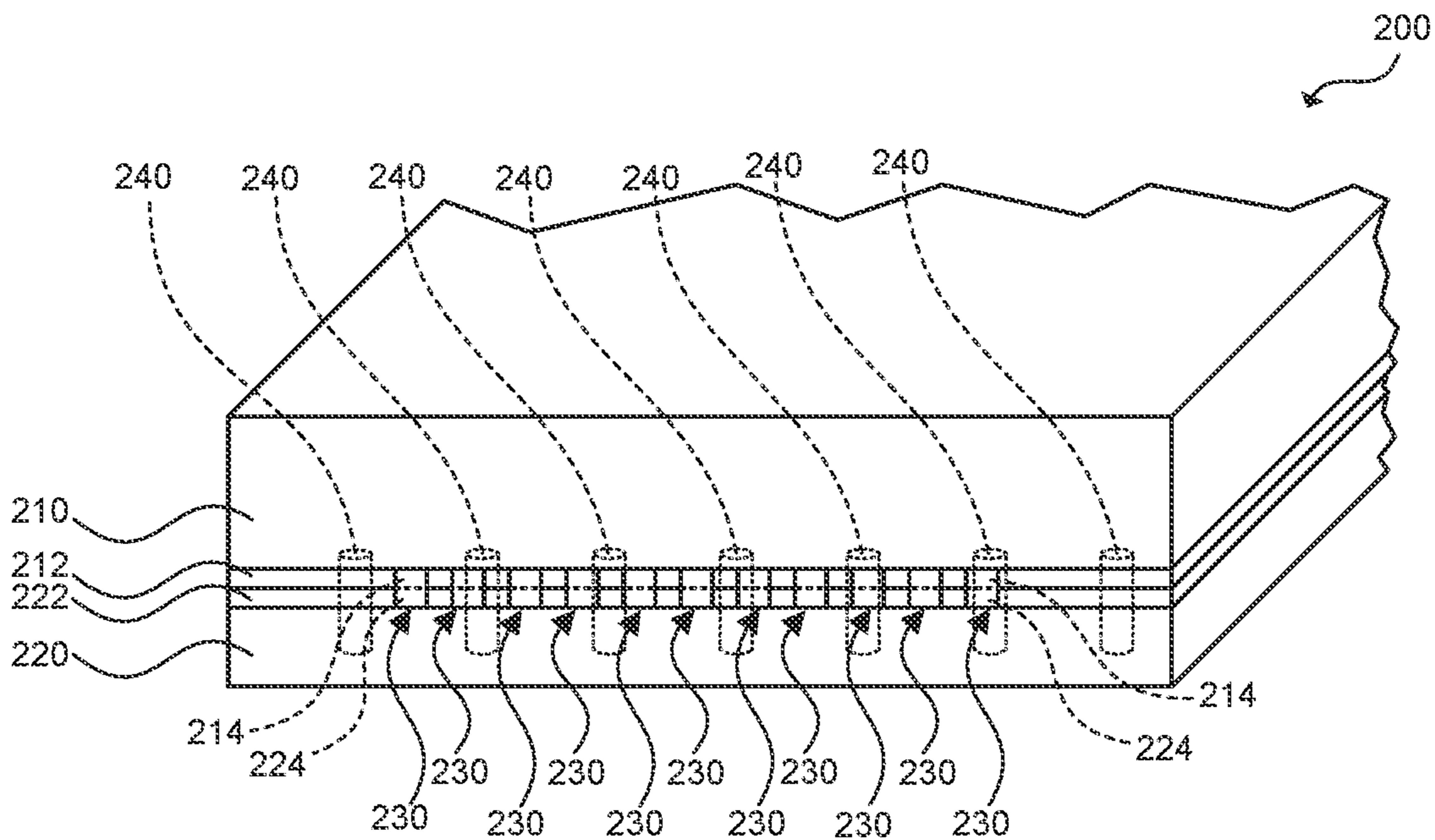
FIG. 1A
