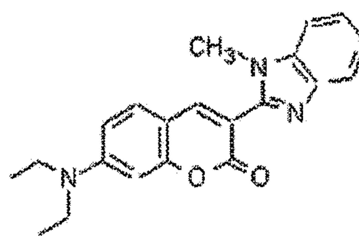
Coumarin 30
