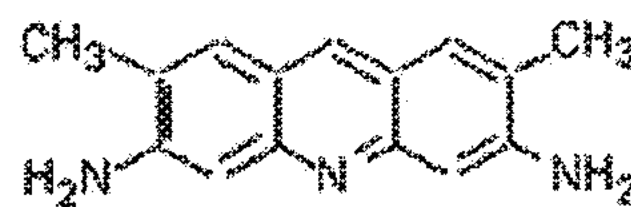
Acridyne Acridyne
