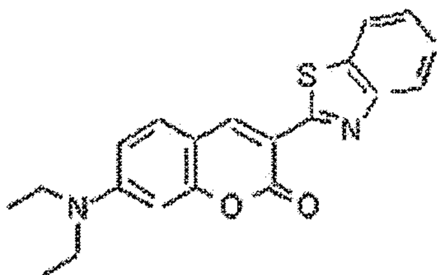
Coumarin 6
