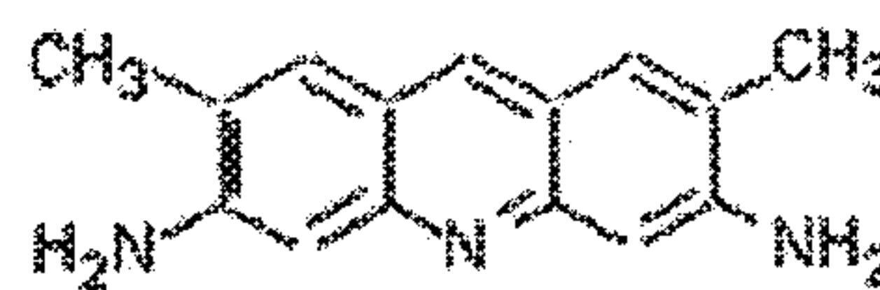
Acridyne Acridyne
