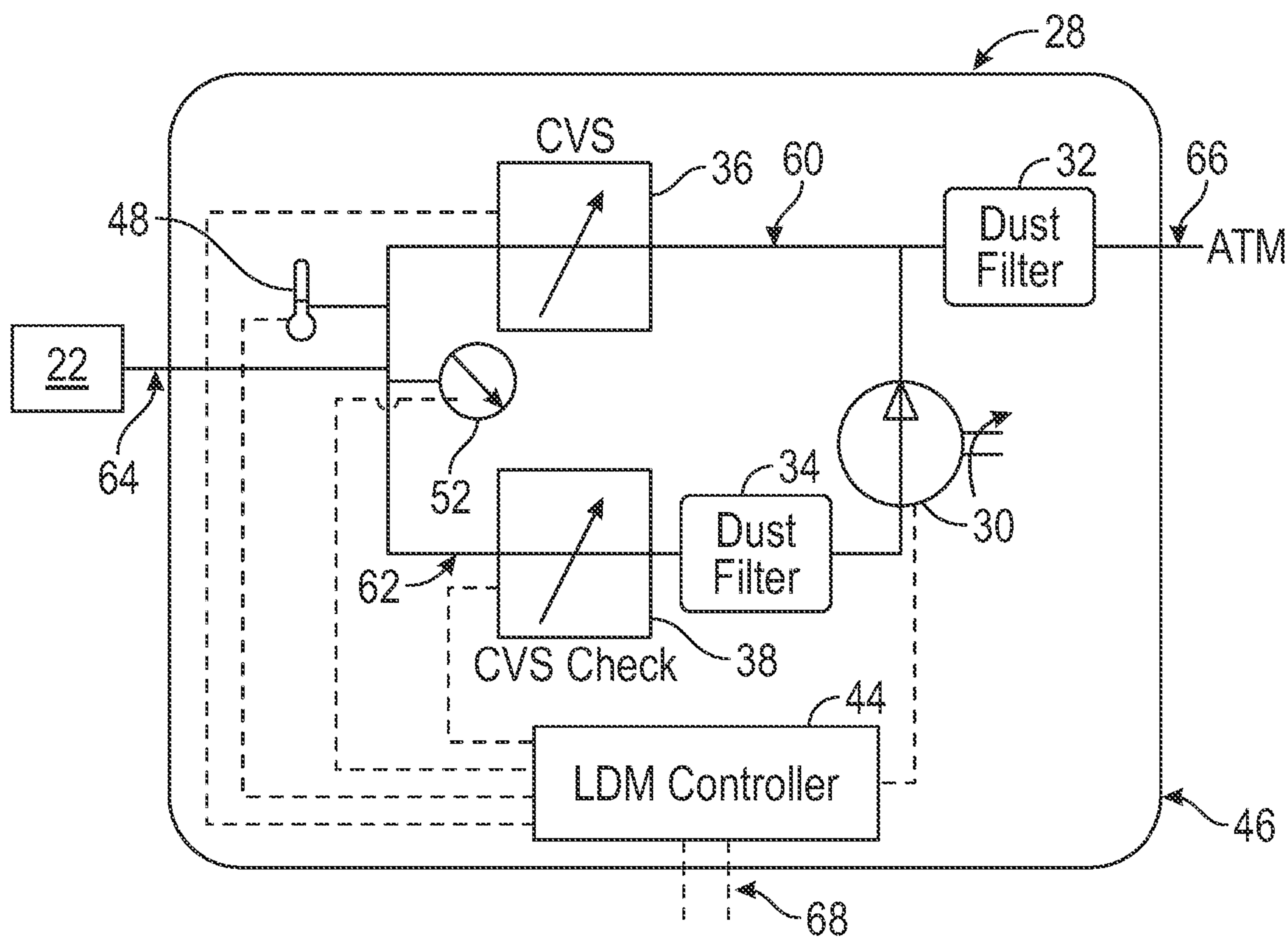
FIG. 2A
