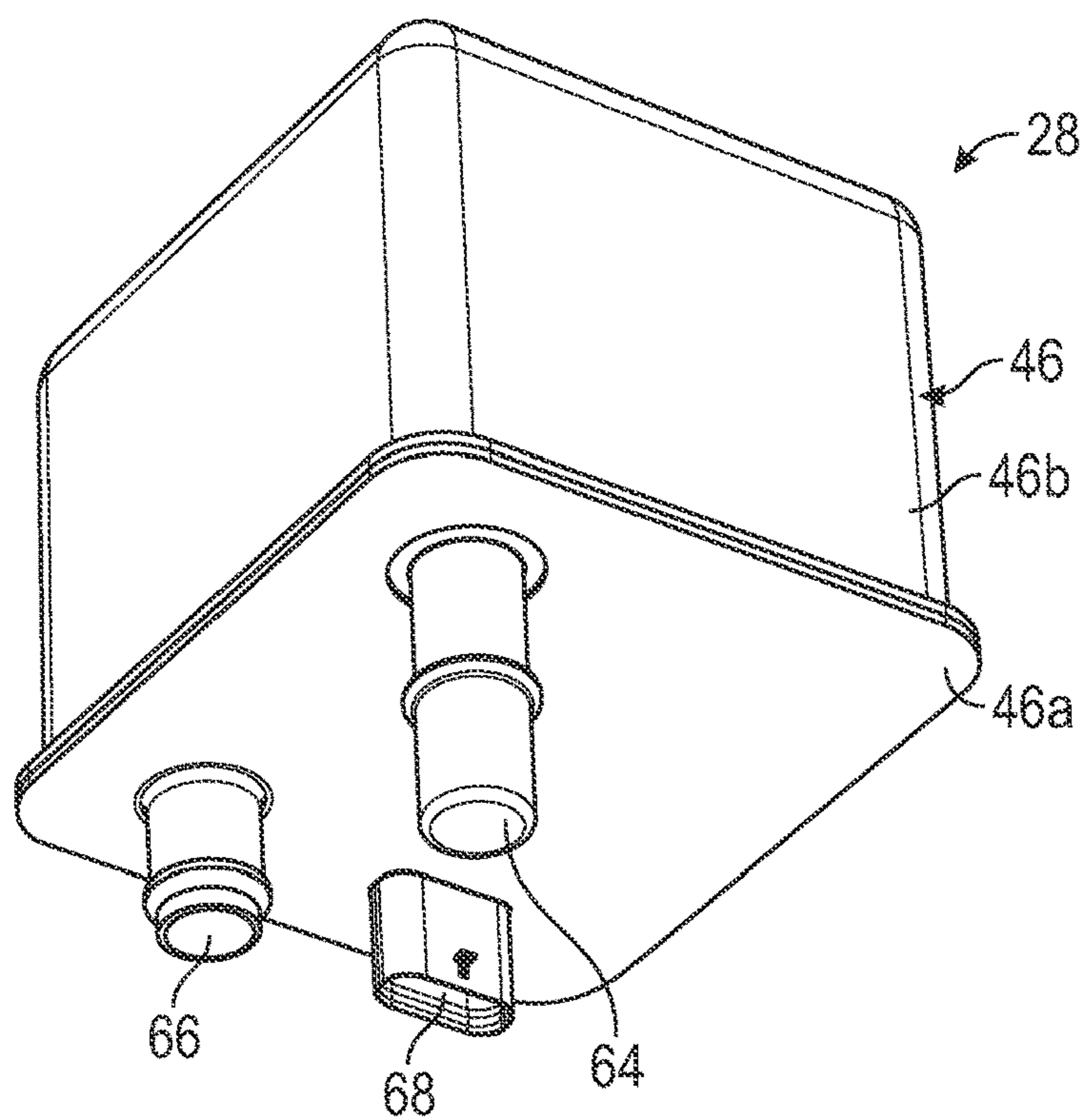
FIG. 3A
