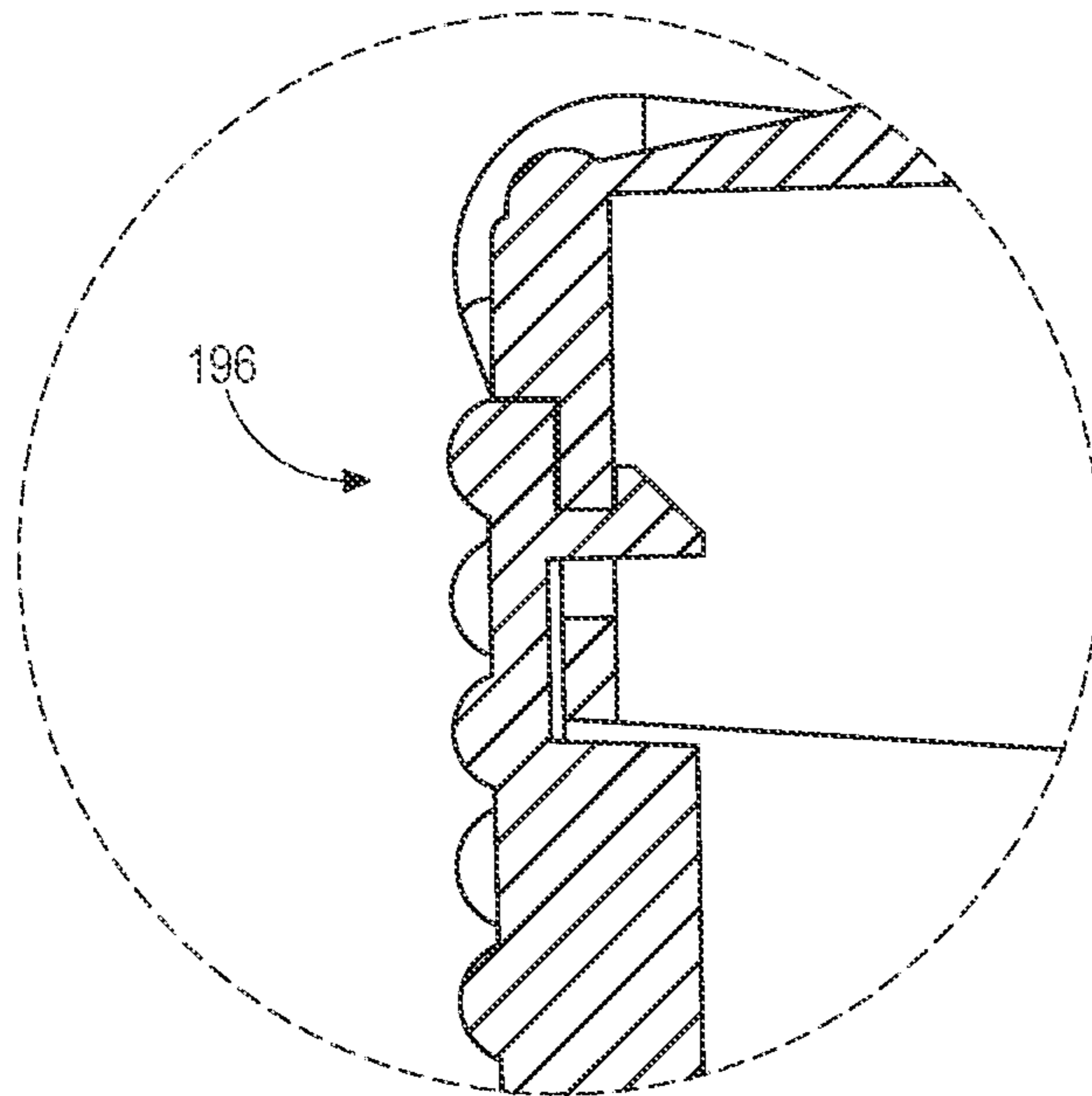
FIG. 19D
