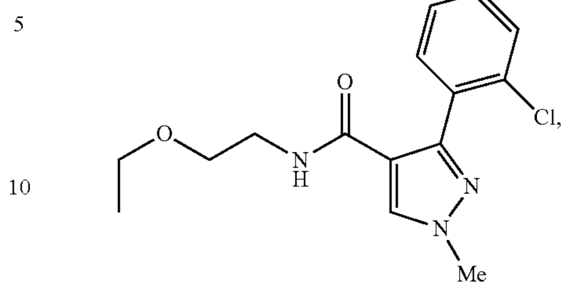
3-(2-chlorophenyl)-N-(2-ethoxyethyl)-1-methyl-1H-pyrazole-4-carboxamide
