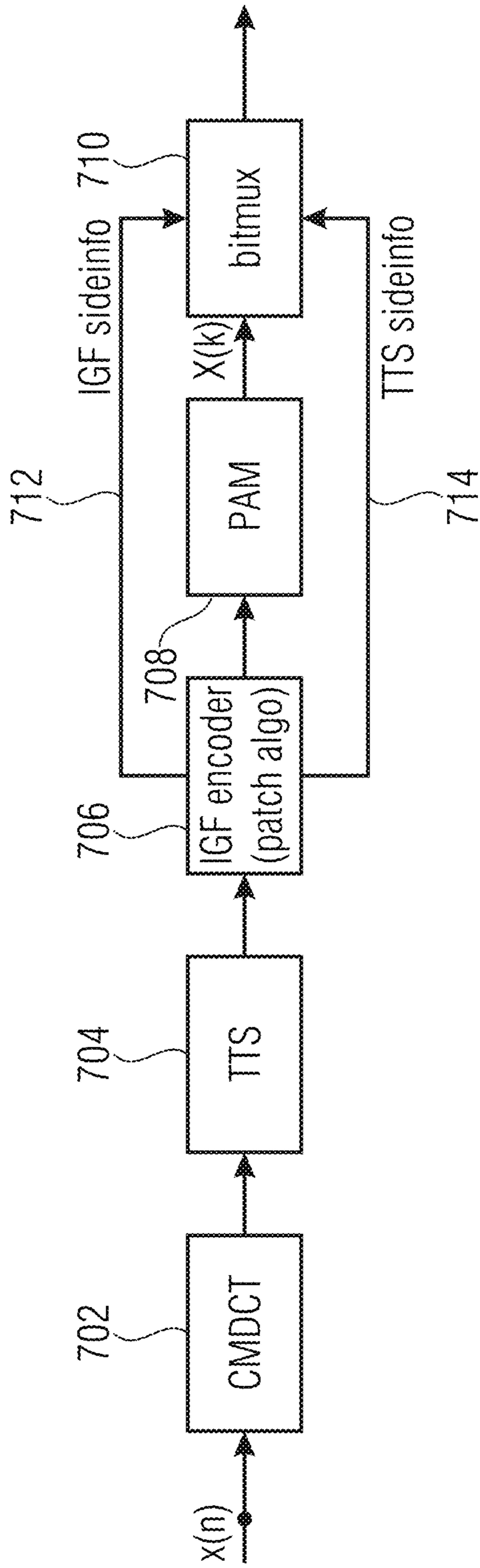
FIG 7A (ENCODER)
