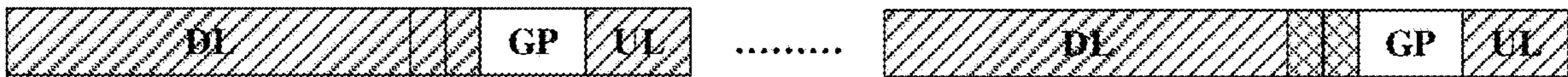
(d) RS transmission periodicity > UL-DL pattern periodicity
