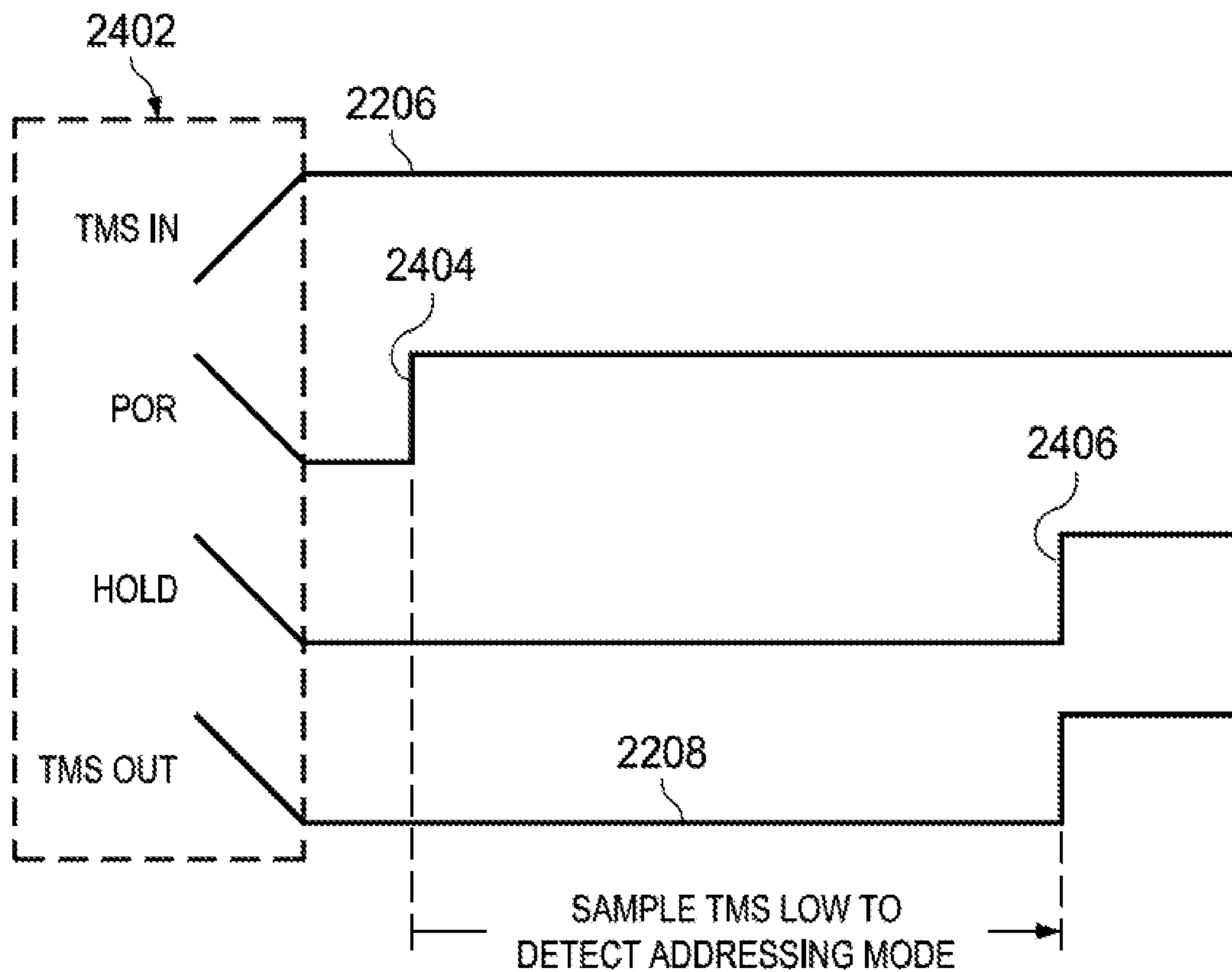
FIG. 24
