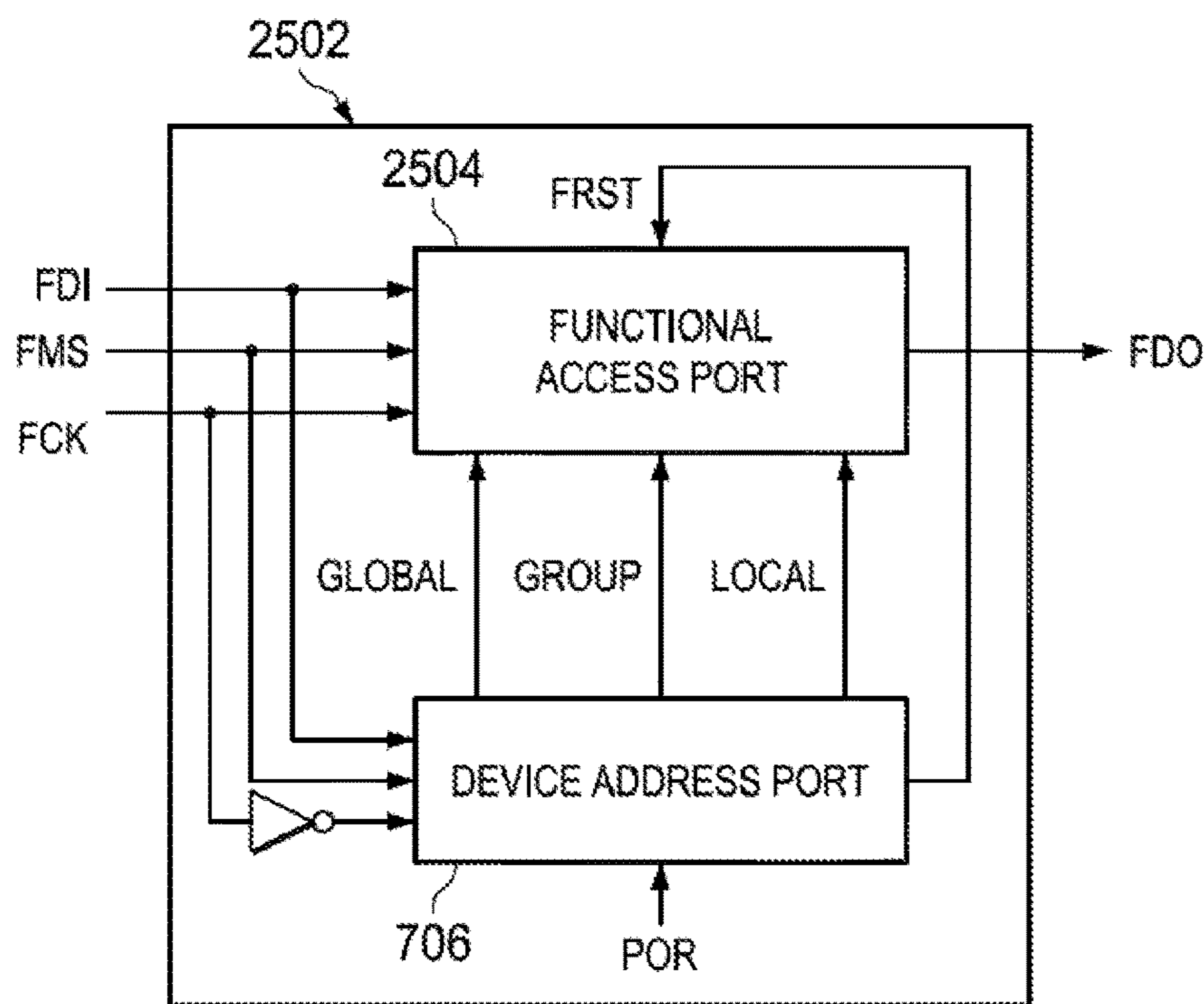
FIG. 25A
