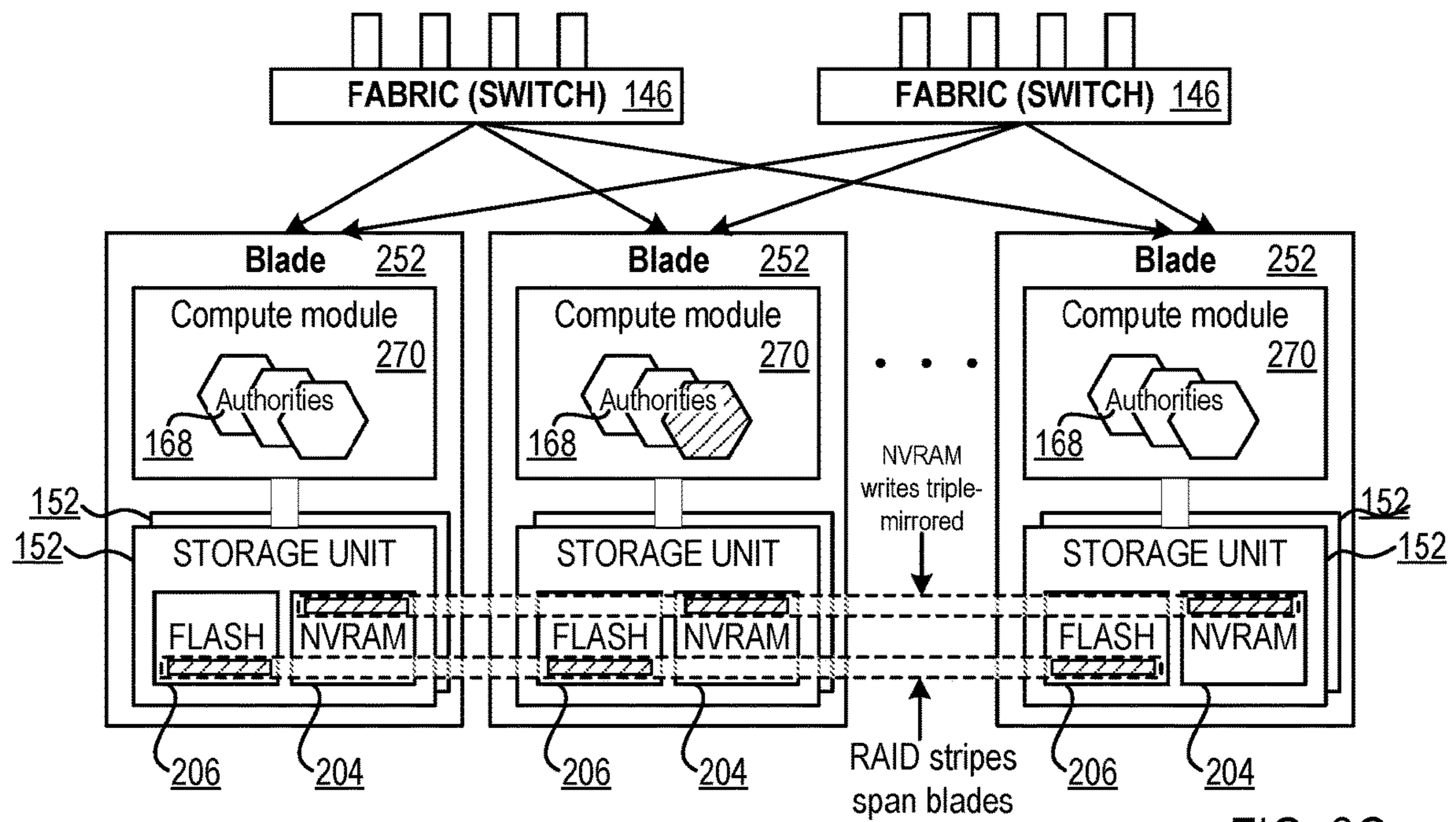
FIG. 2G
