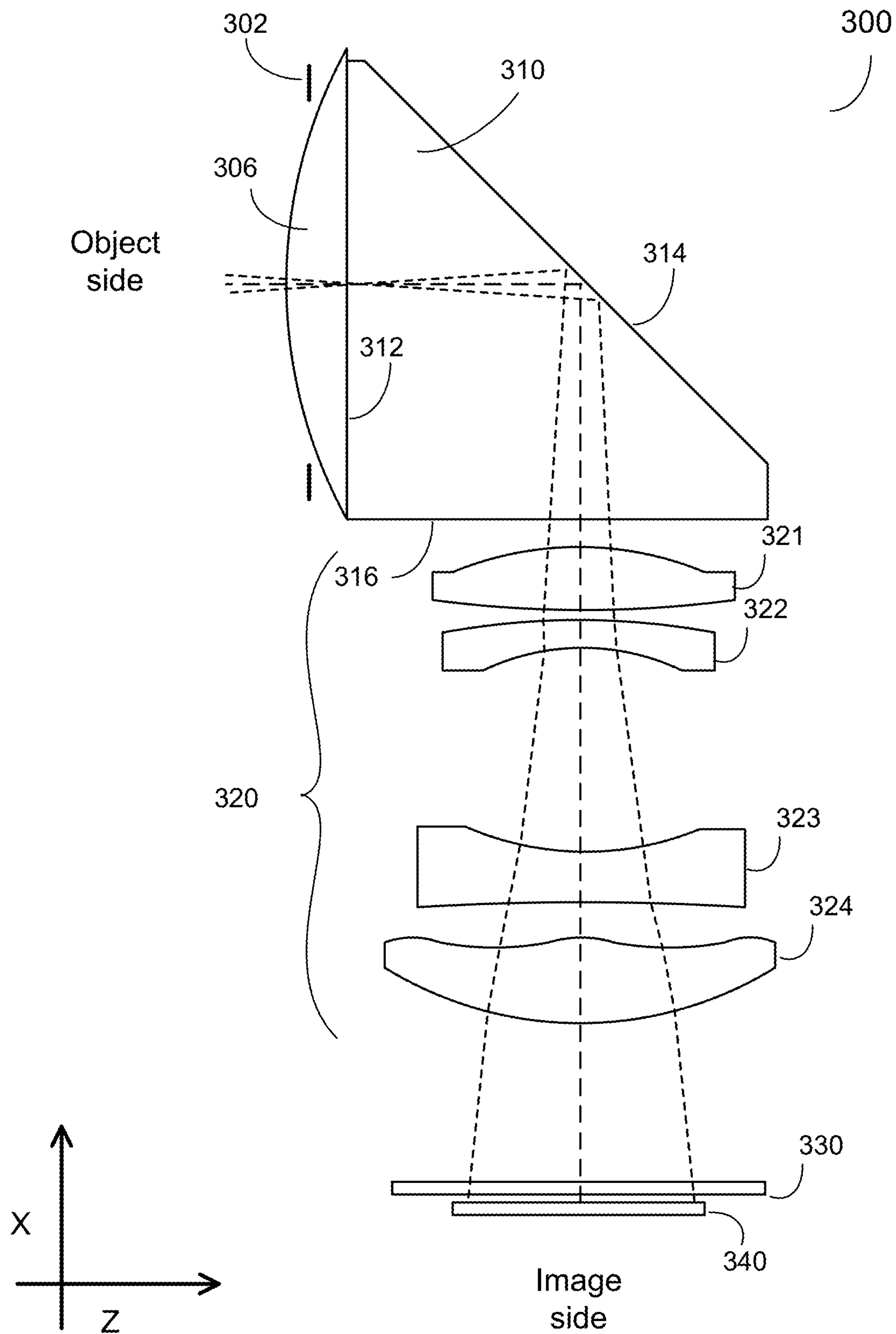
FIG. 3
