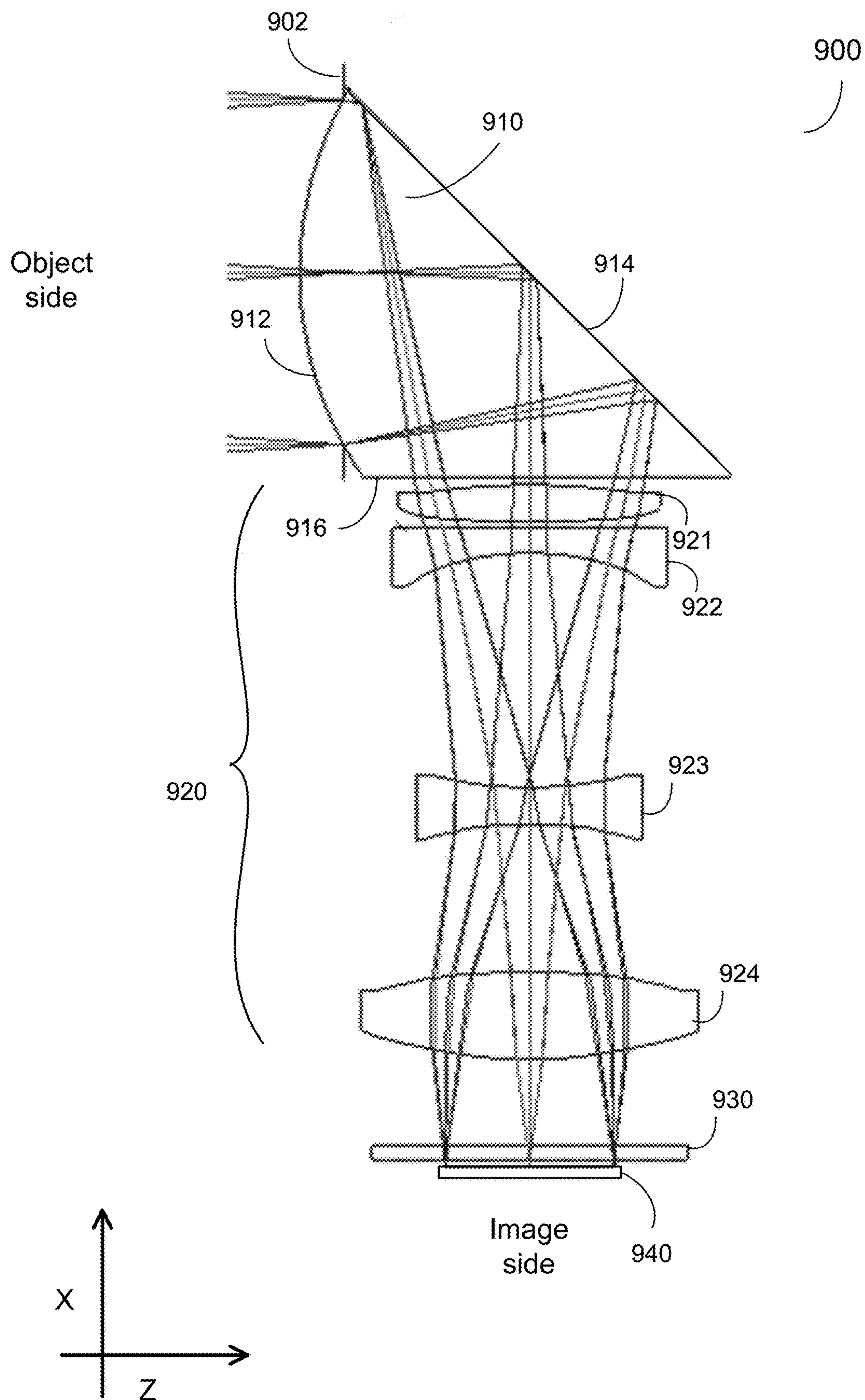
FIG. 9A
