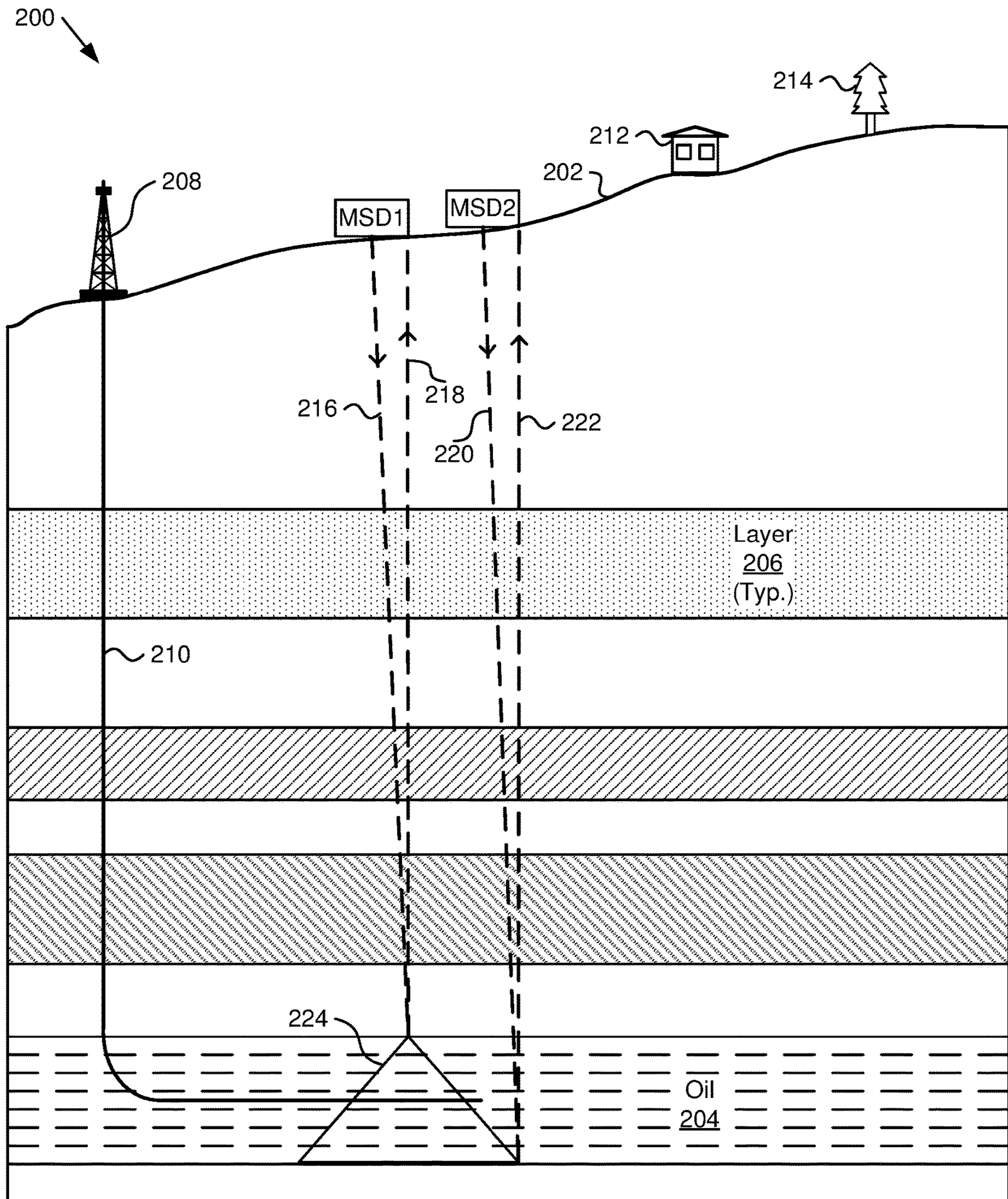
FIG. 2
