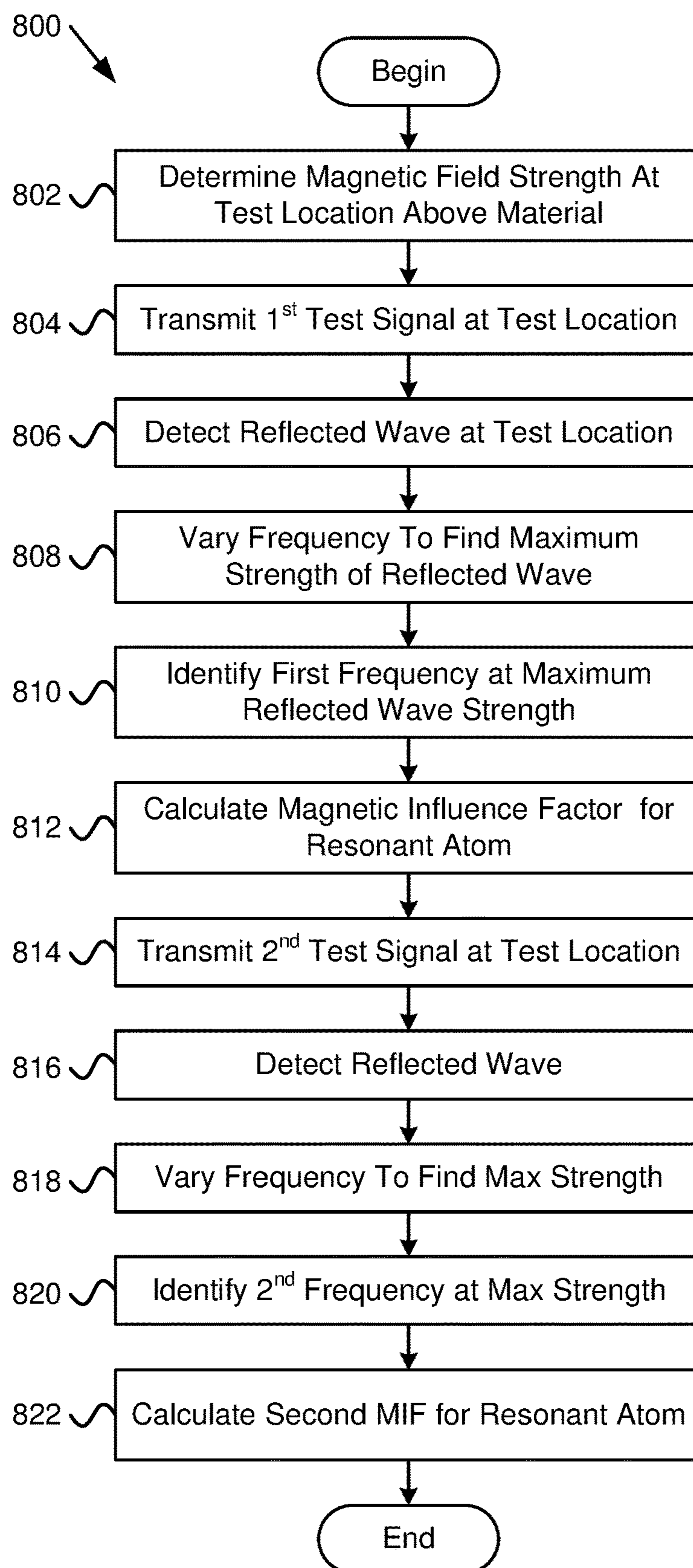
FIG. 8
