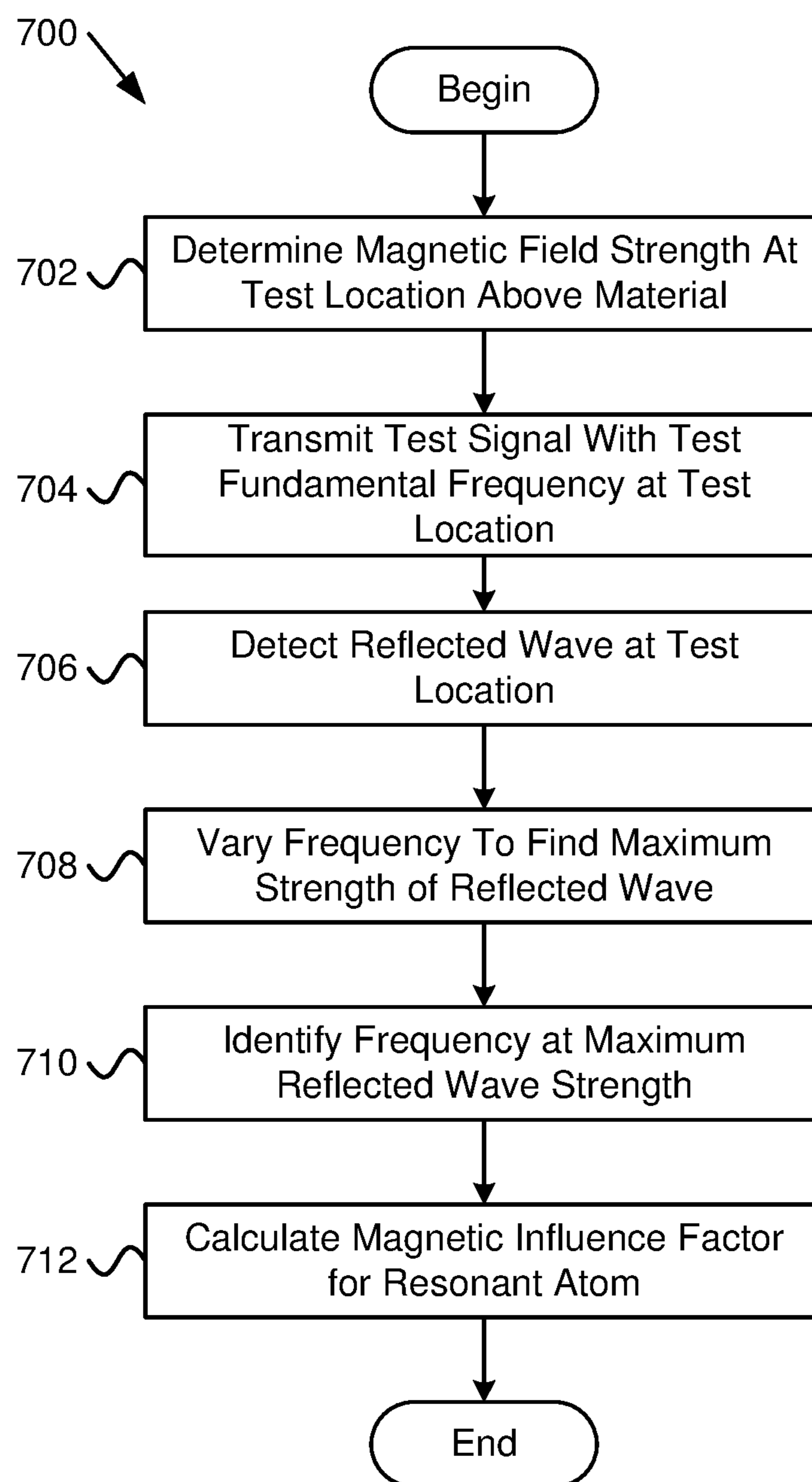
FIG. 7
