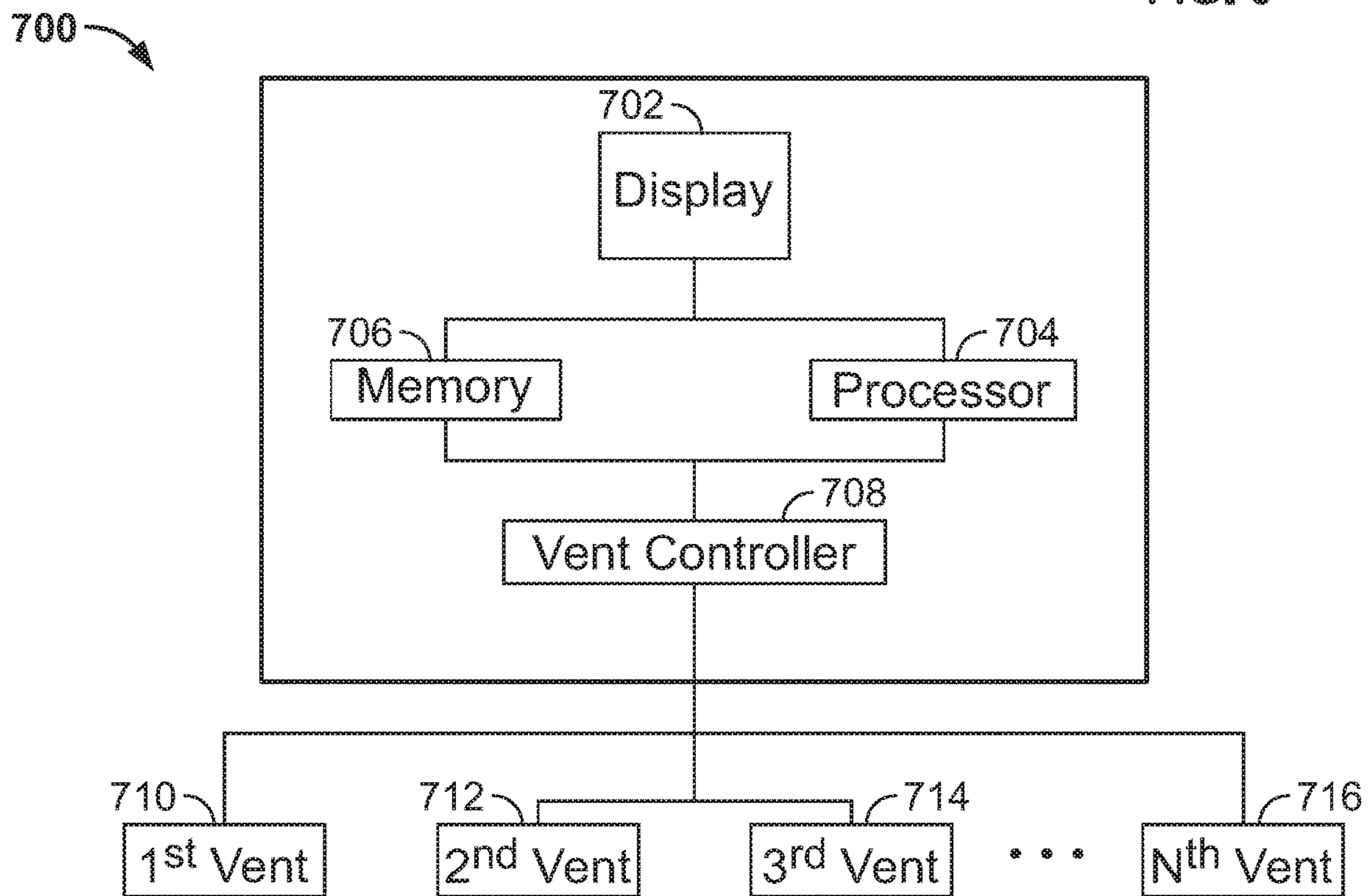
FIG. 7
