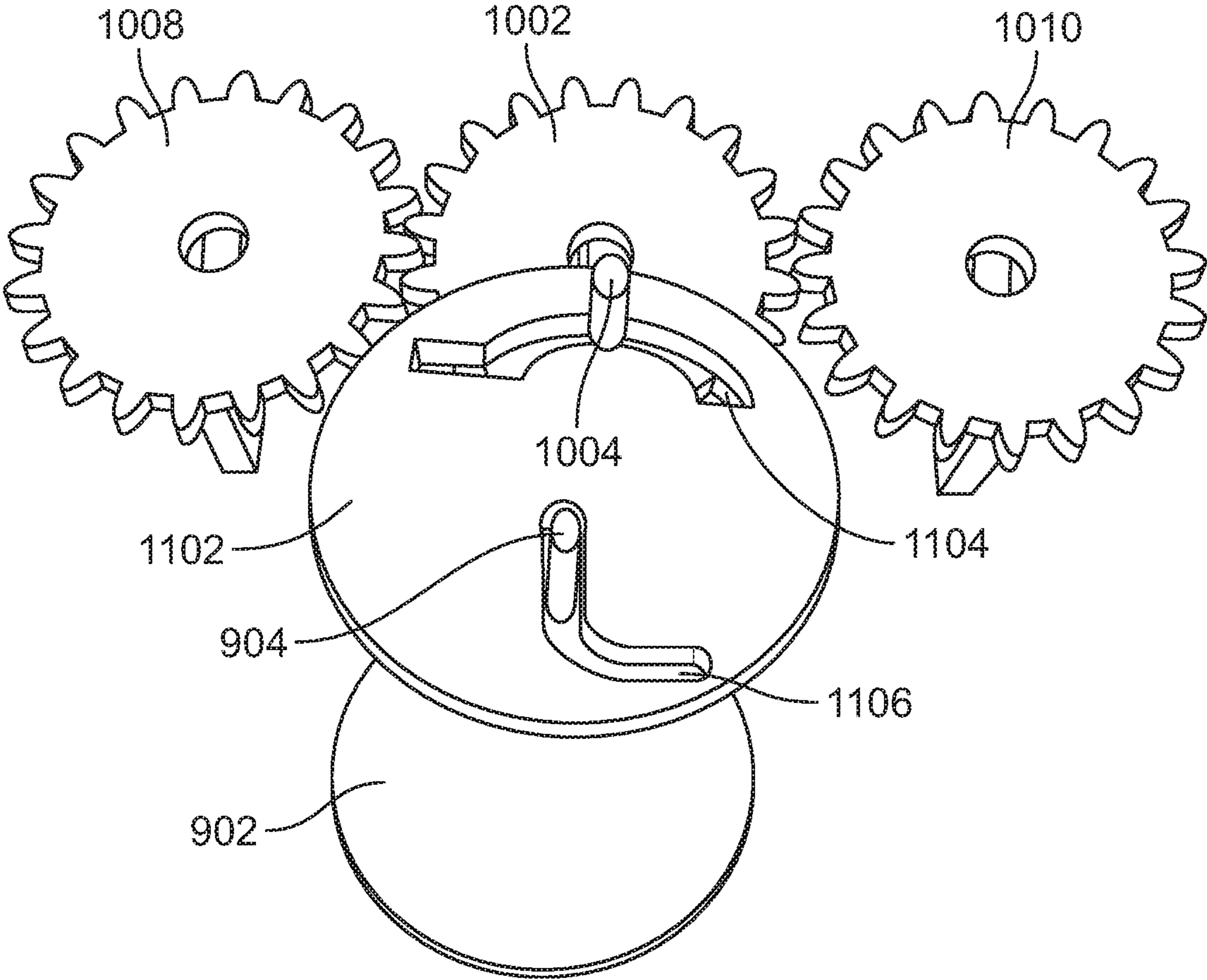
FIG. 12A
