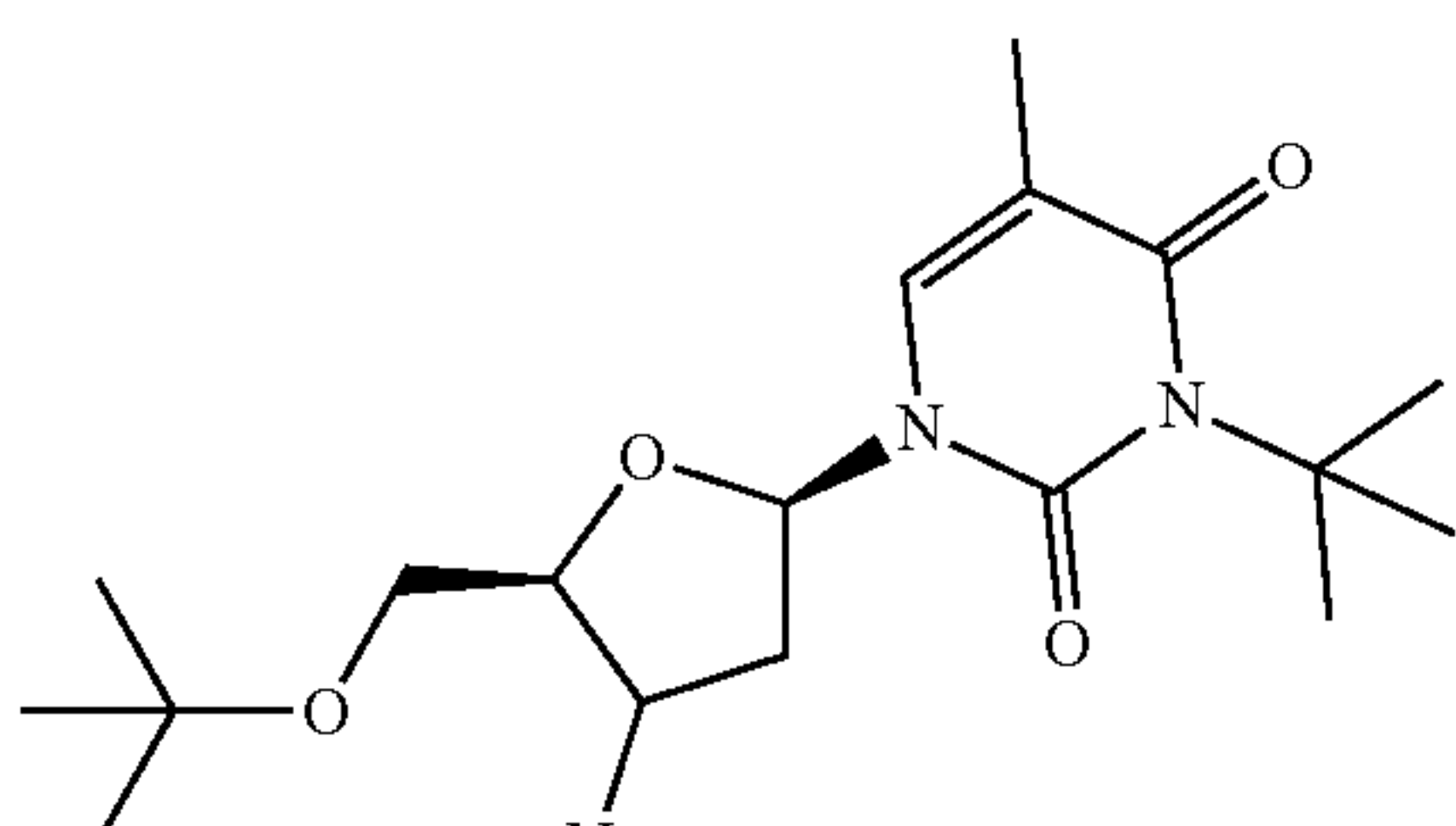
2-tert-butyl-AZT
