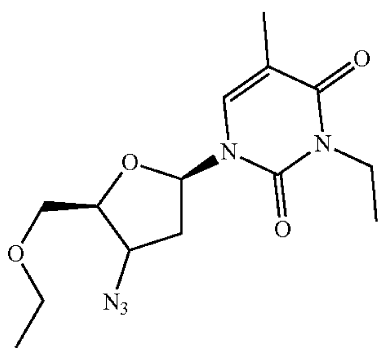
2-Et-AZT
