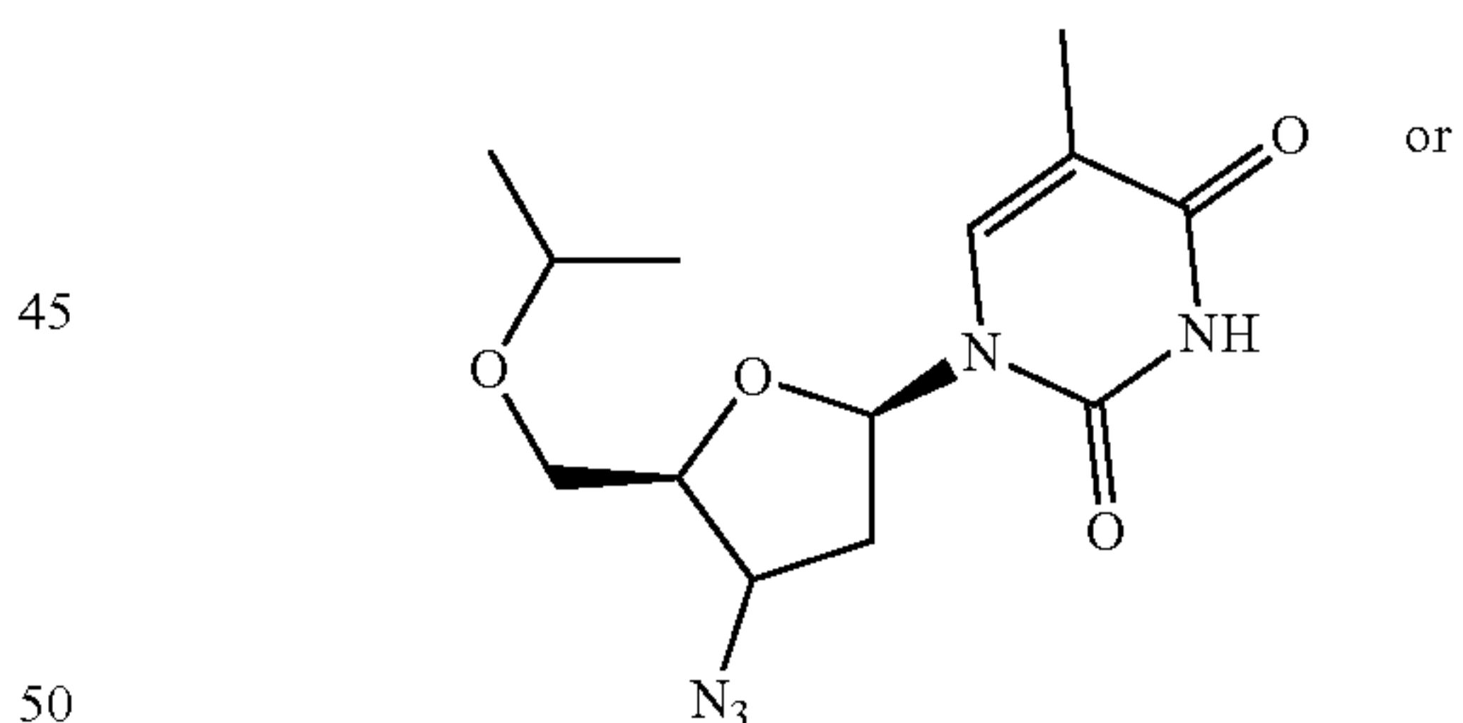
O-isopropyl-AZT
