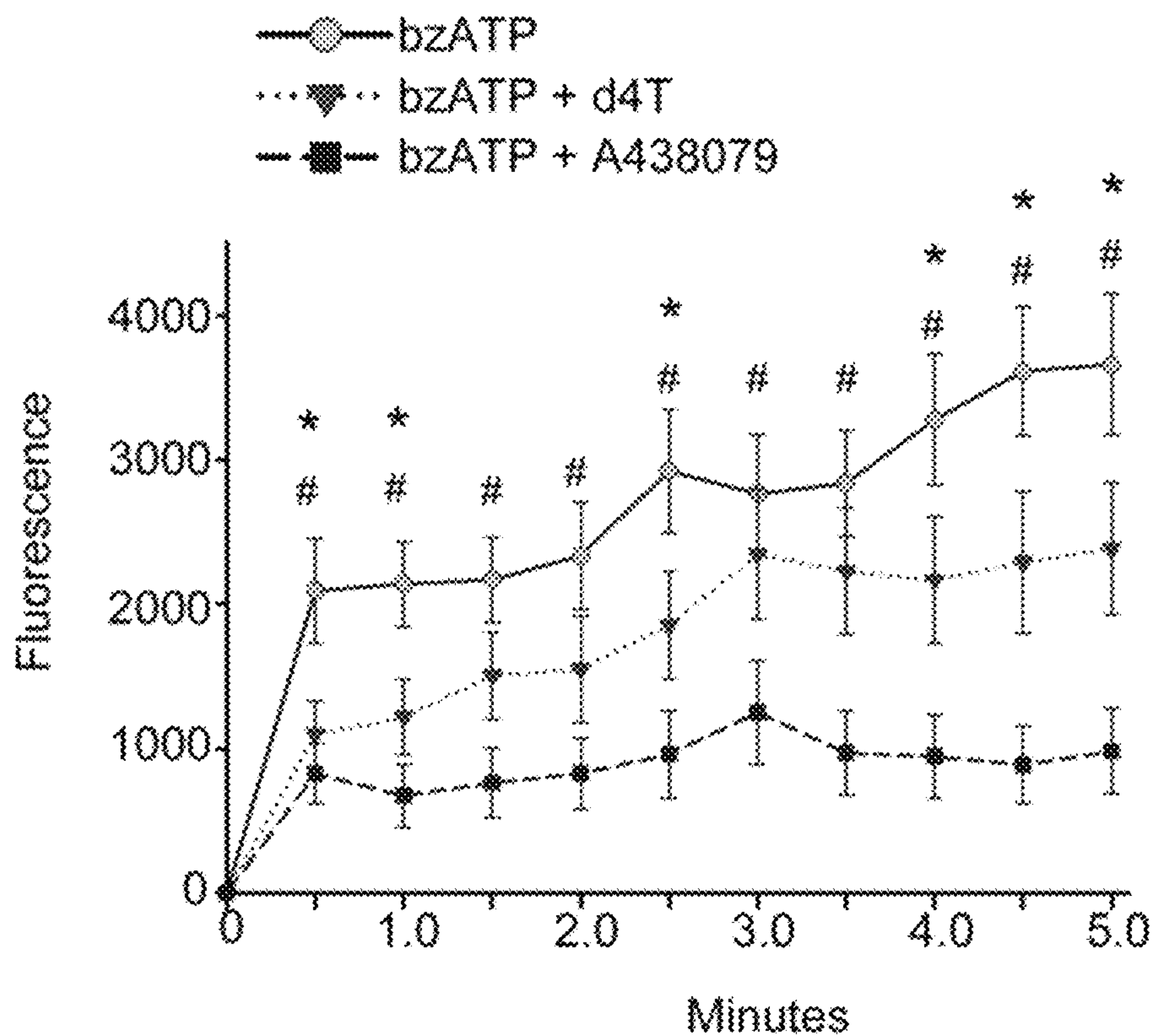
FIG. 43
