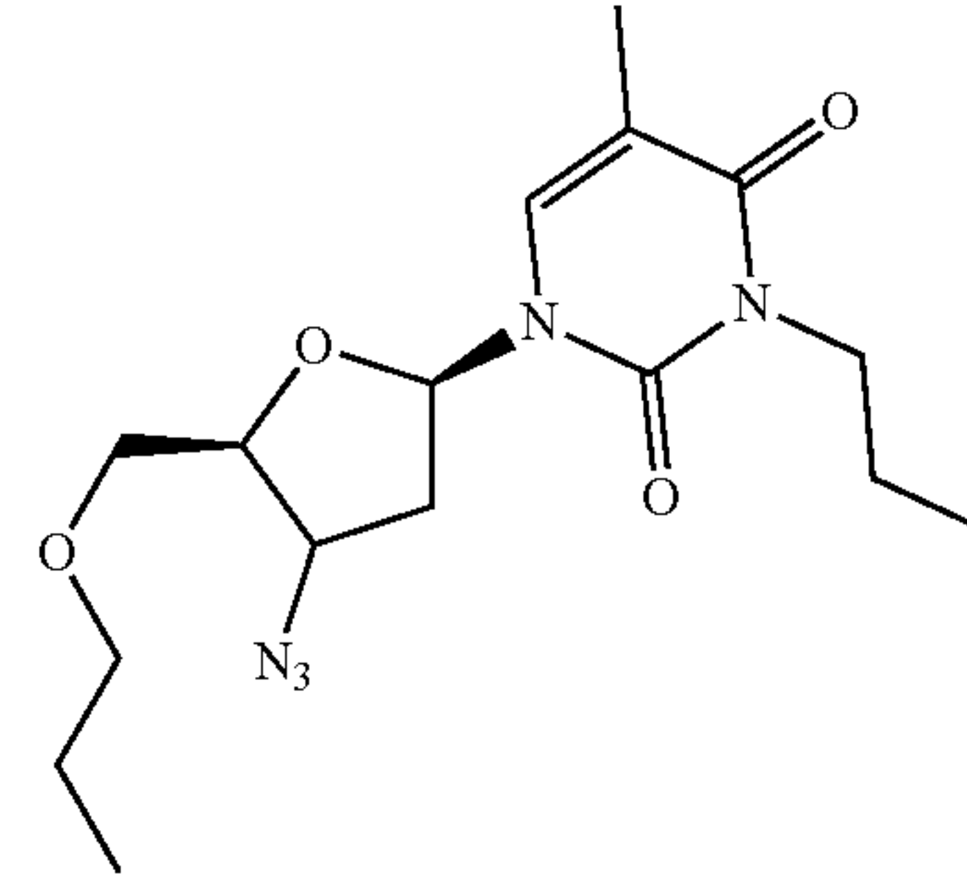
2-Propyl-AZT
