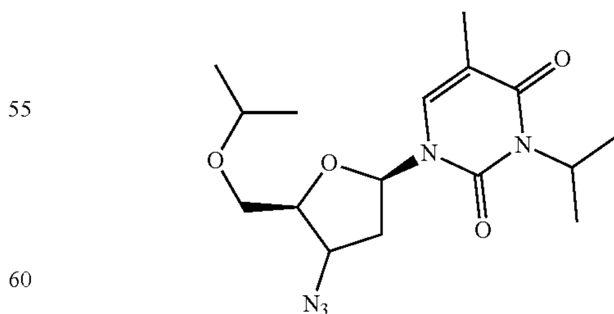
2-isopropyl-AZT
