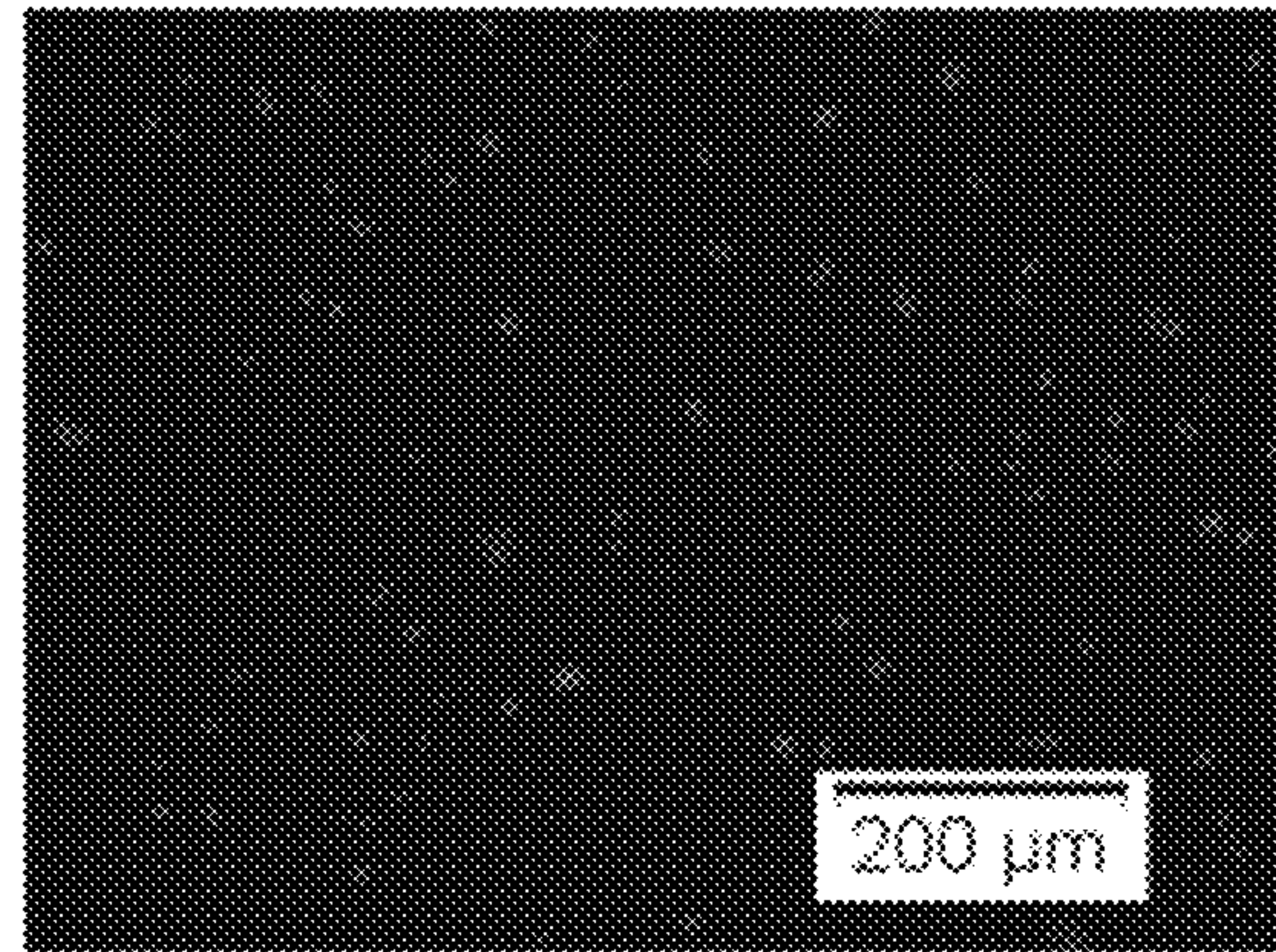
pAluA
