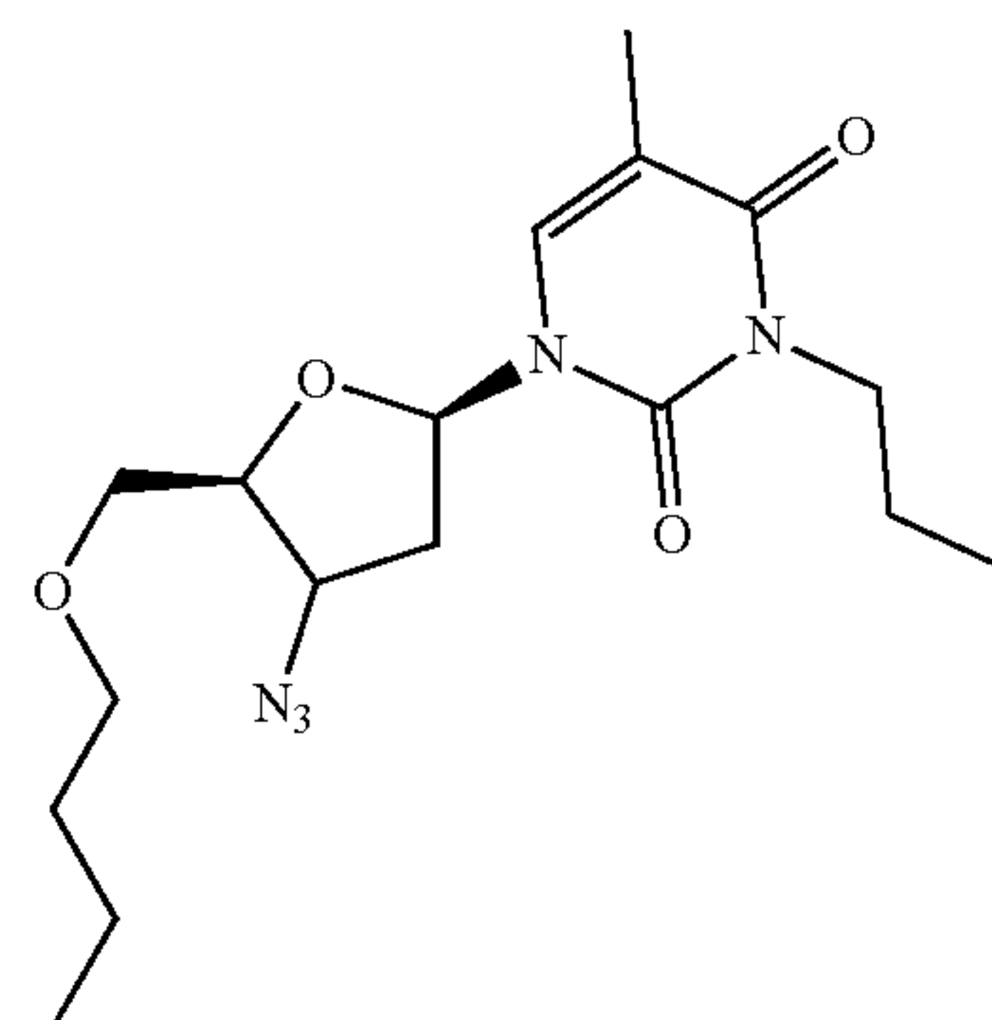
2-Butyl-AZT
