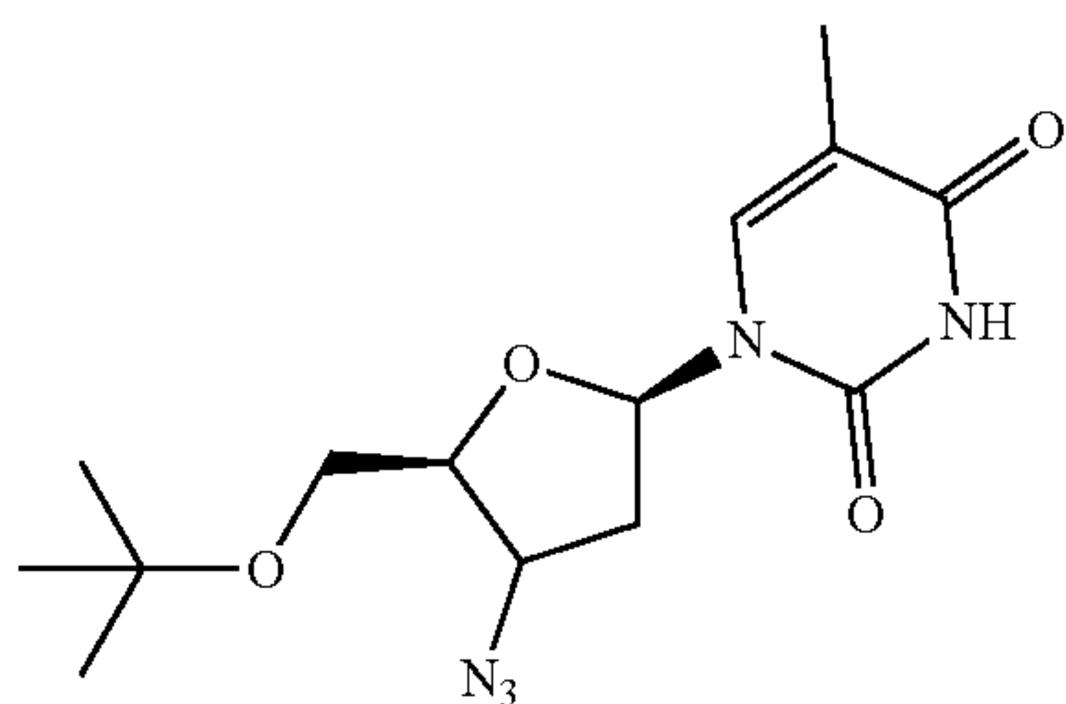
O-tert-butyl-AZT
