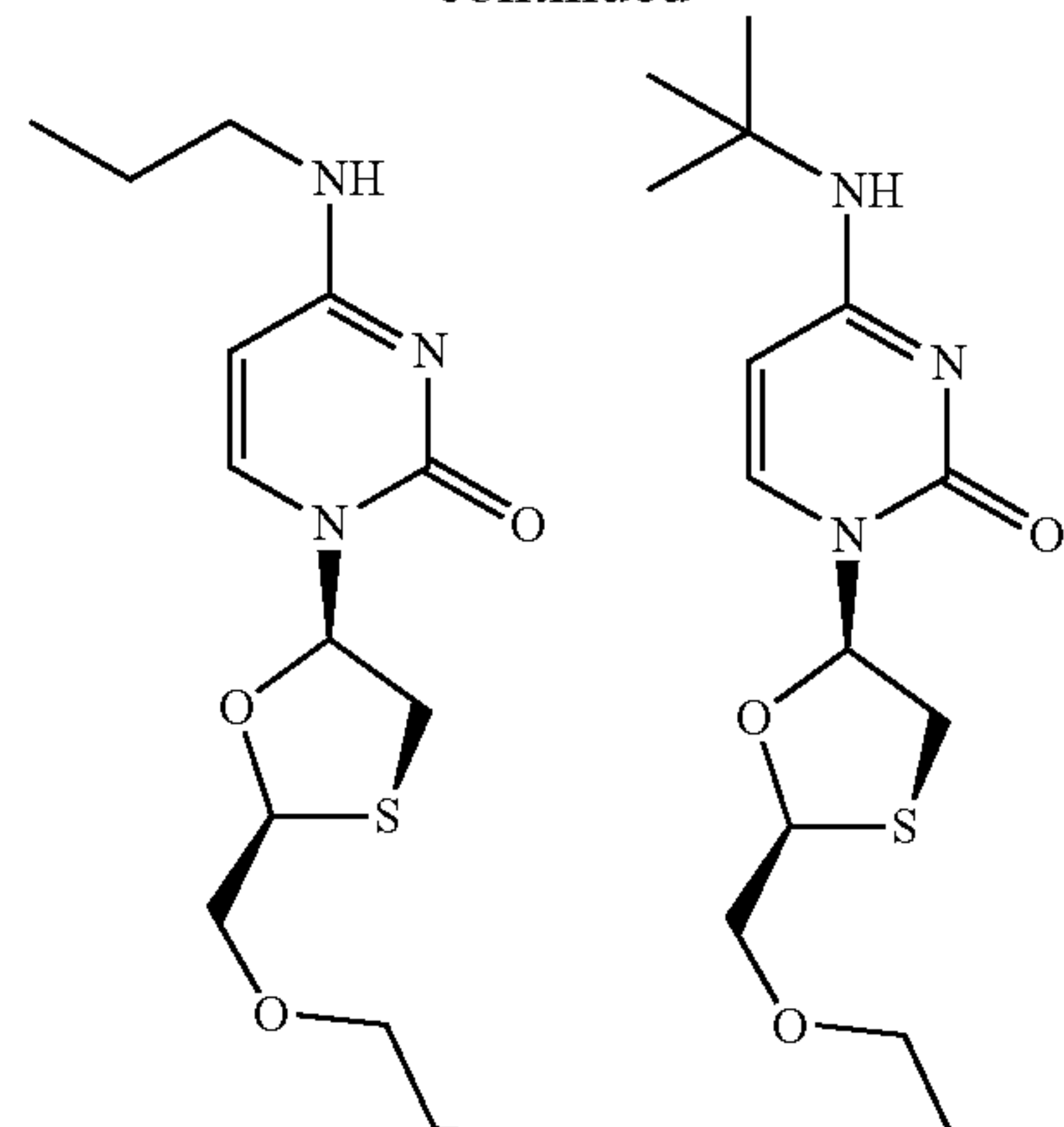
3tc-C6-3,3,0
