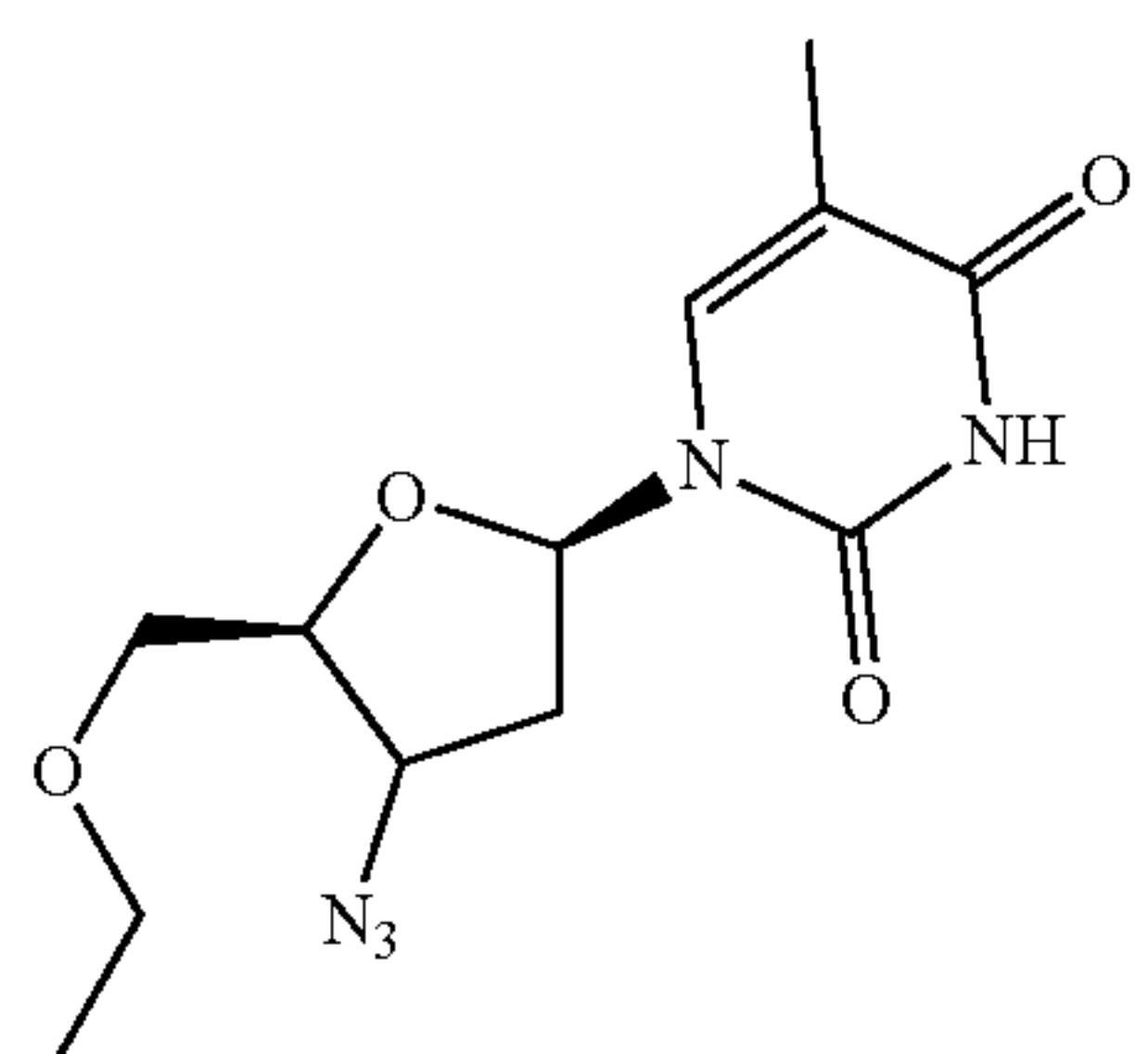
O-Et-AZT
