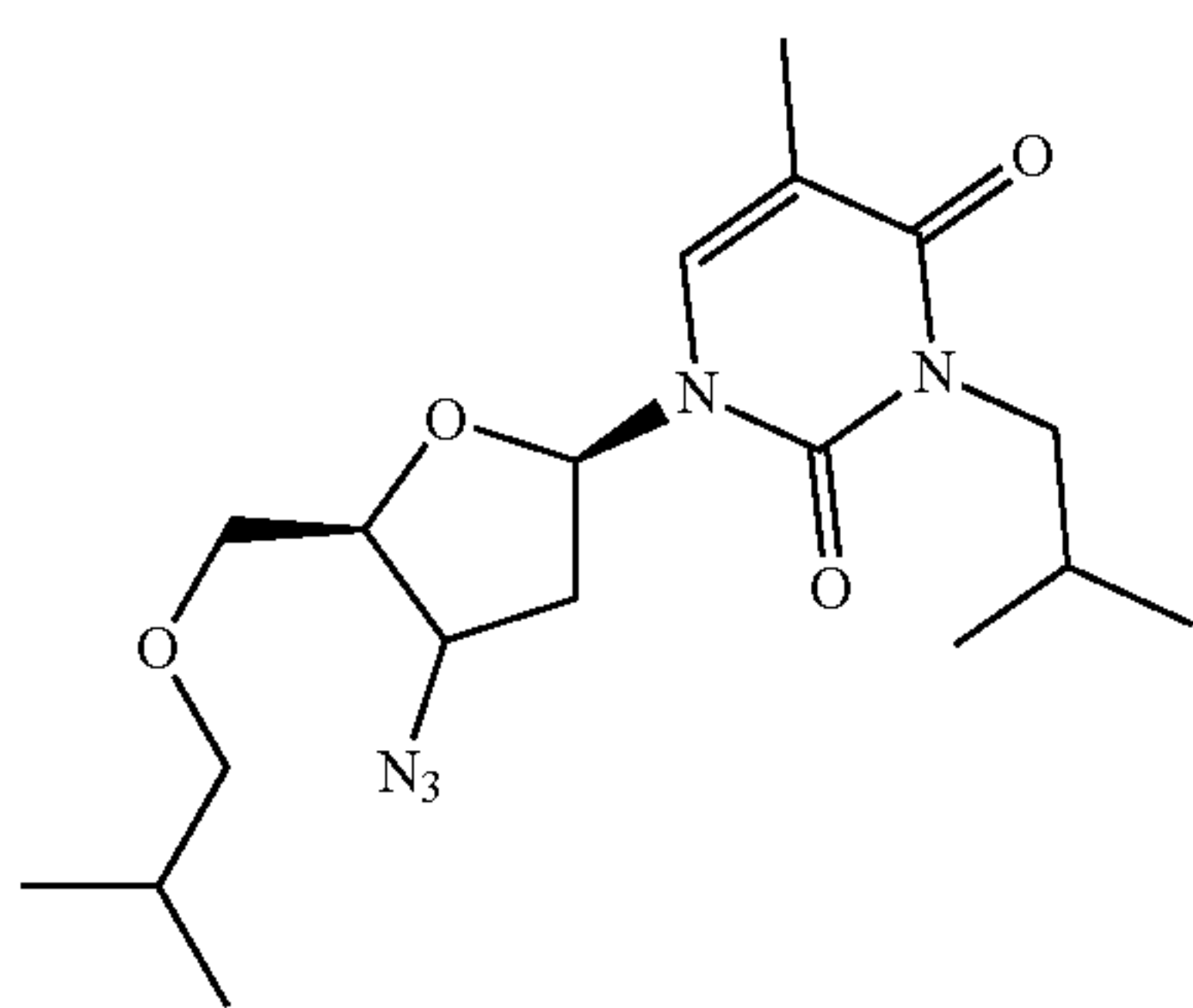
2-isobutyl-AZT
