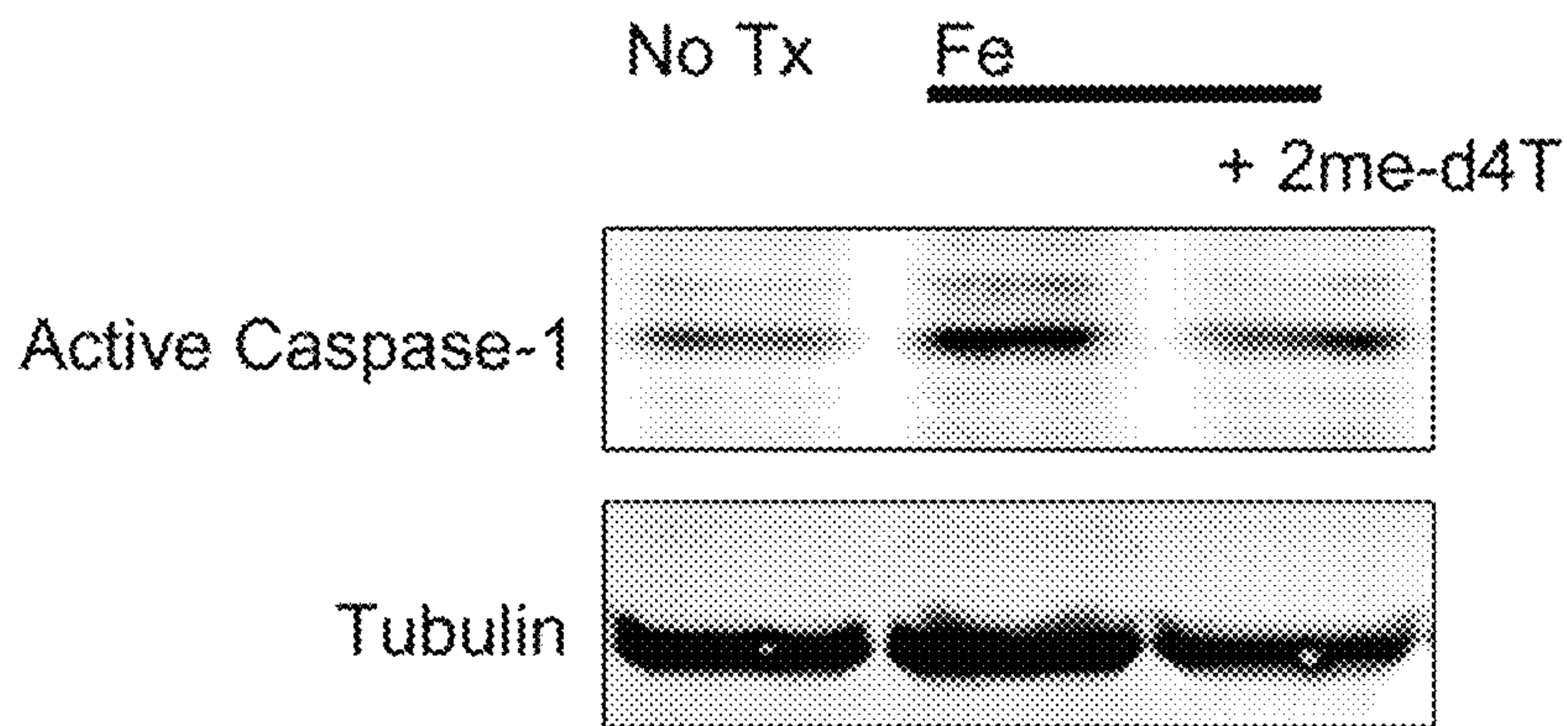
FIG. 57
