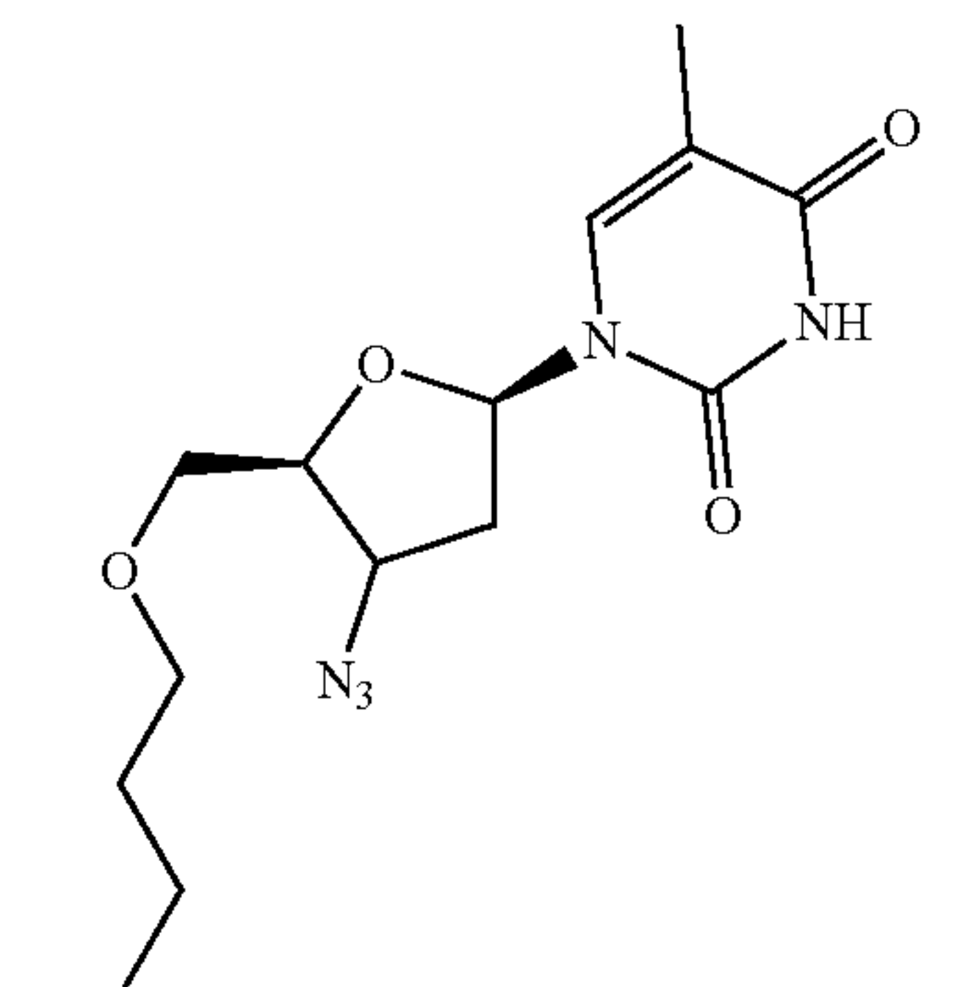
O-Butyl-AZT
