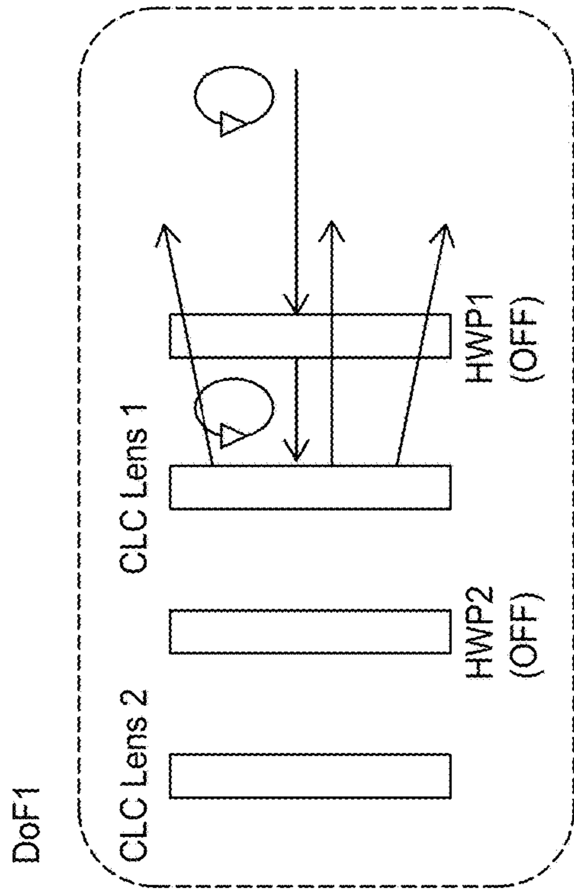
FIG. 33B
