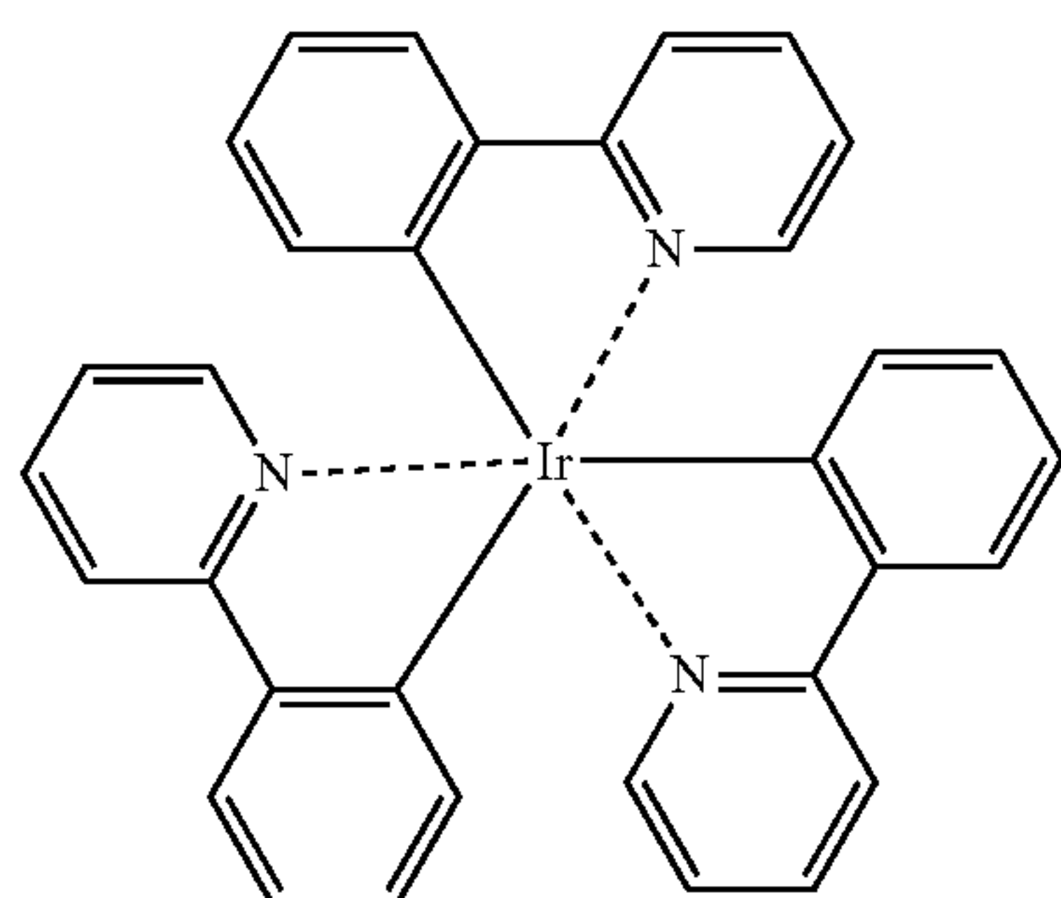
Ir(ppy) 3
