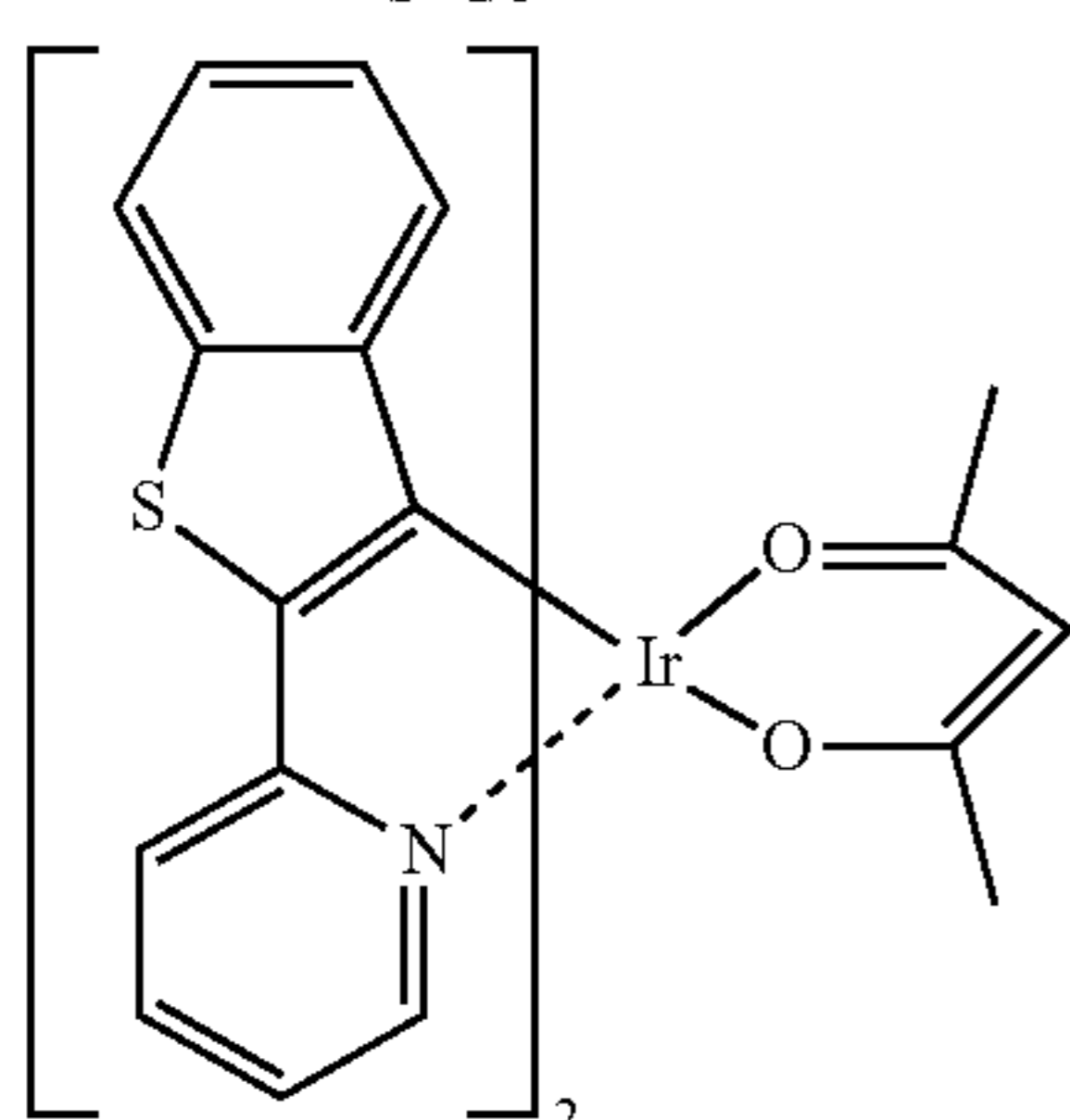
Btp 2 Ir(acac)
