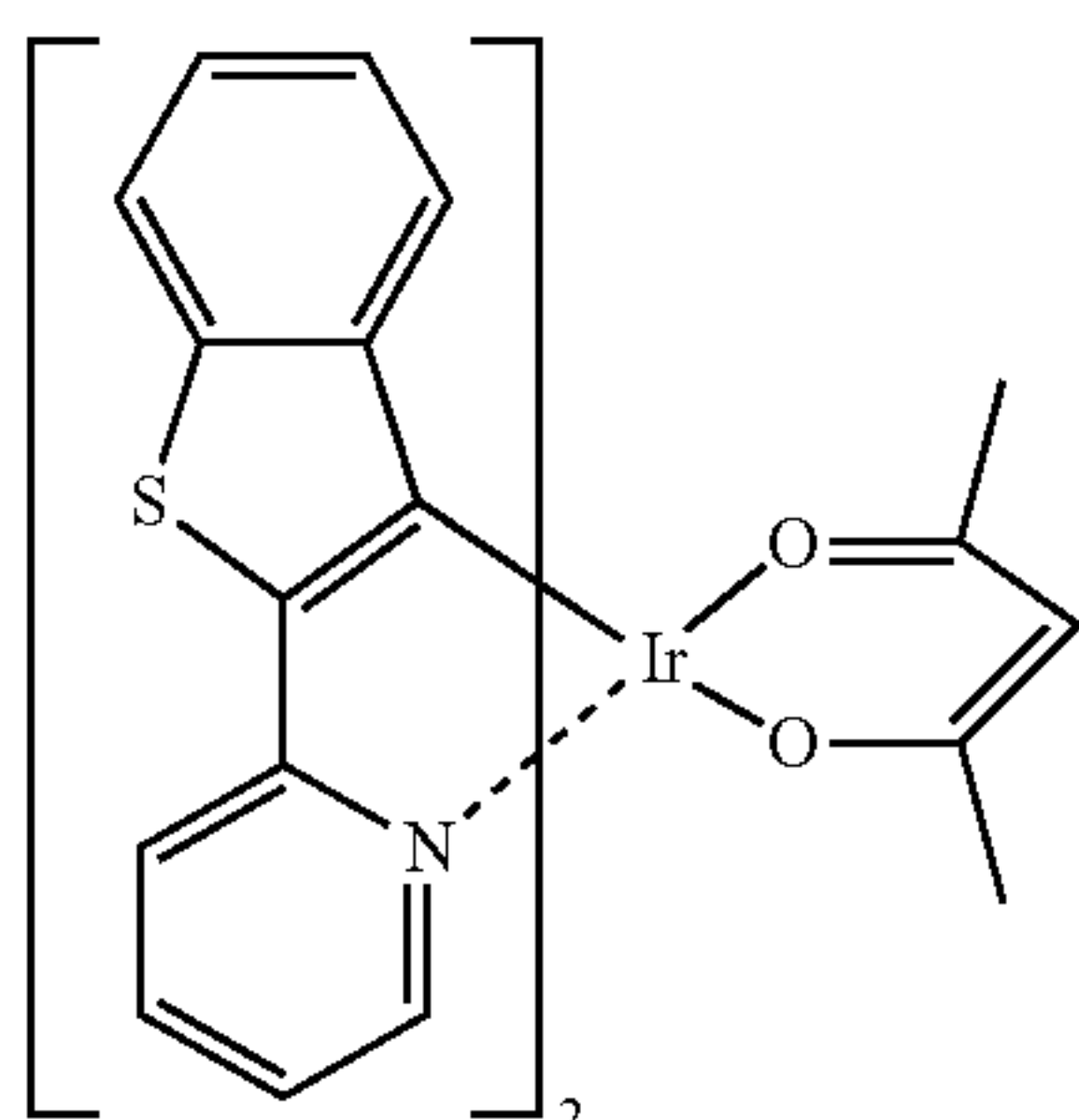
Btp 2 Ir(acac)
