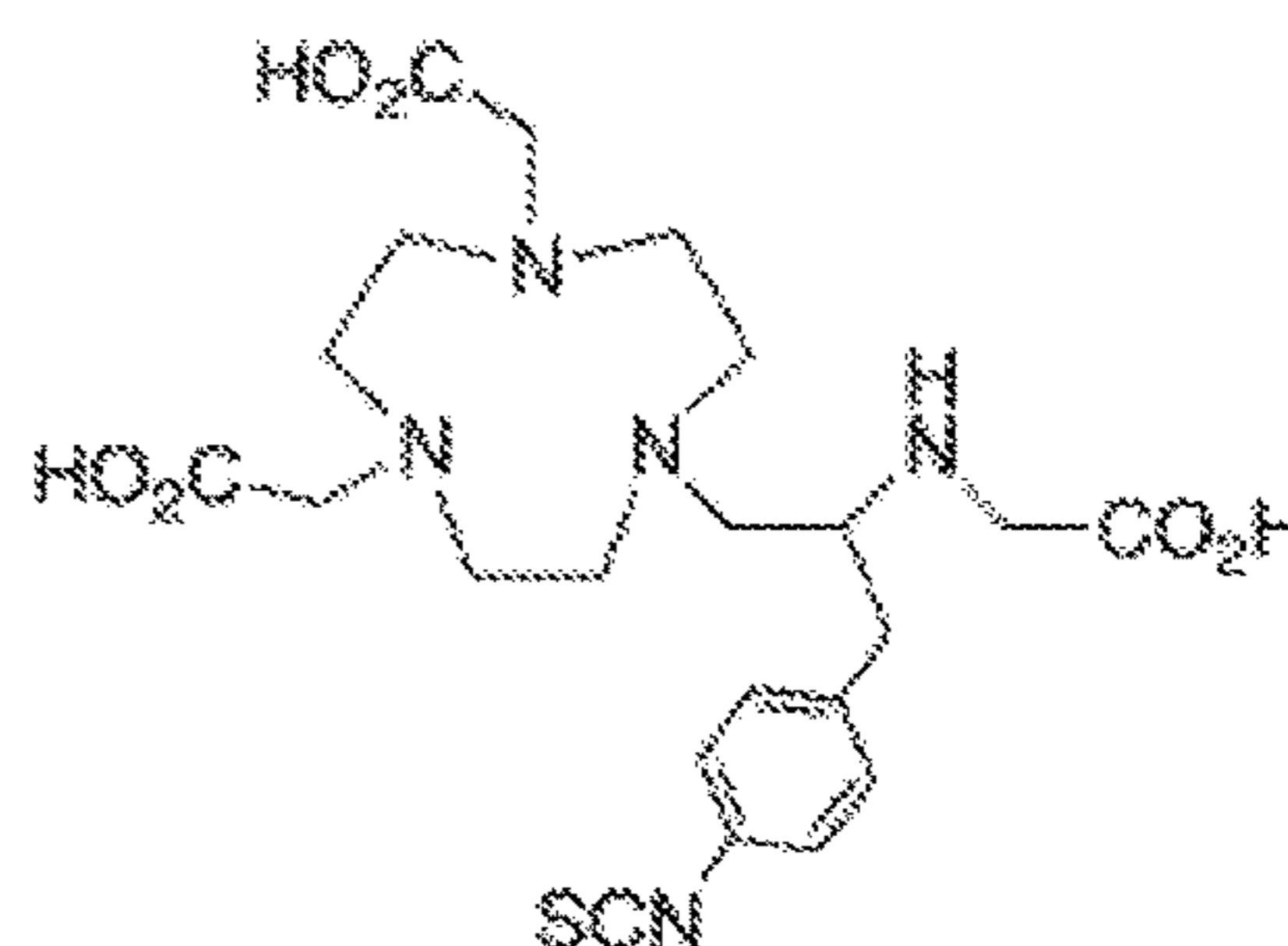
C-NE3TA-NCS
