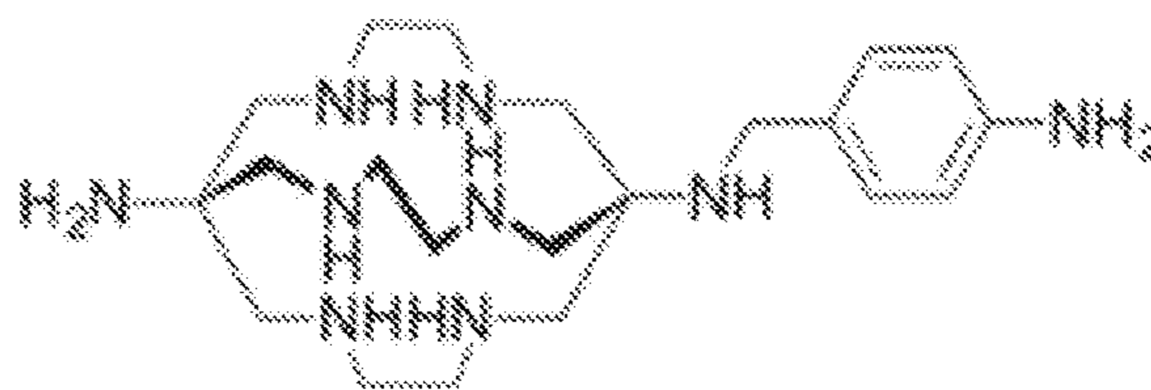
SarAr
