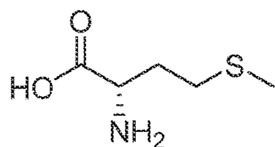
L-Methionine
