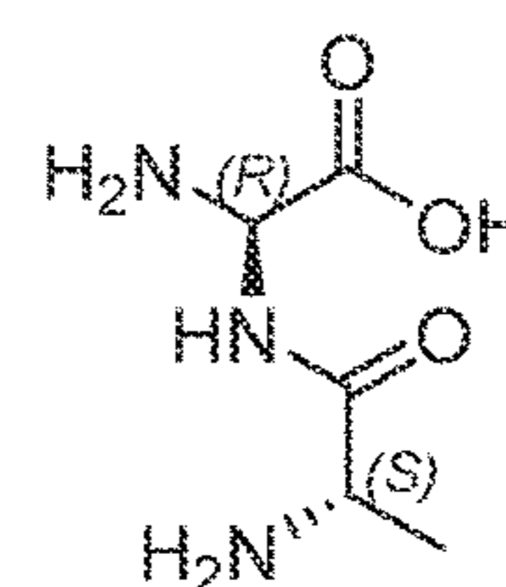
D-Agl(βAla)
