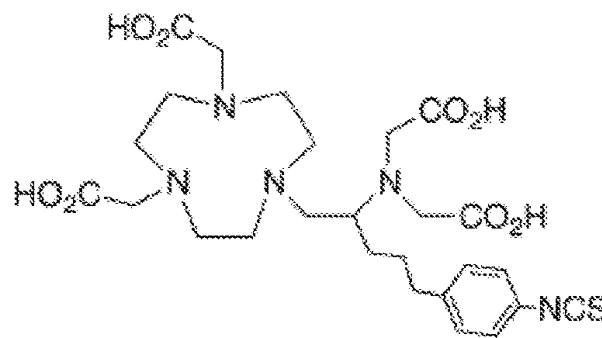
3 p -C-NETA
