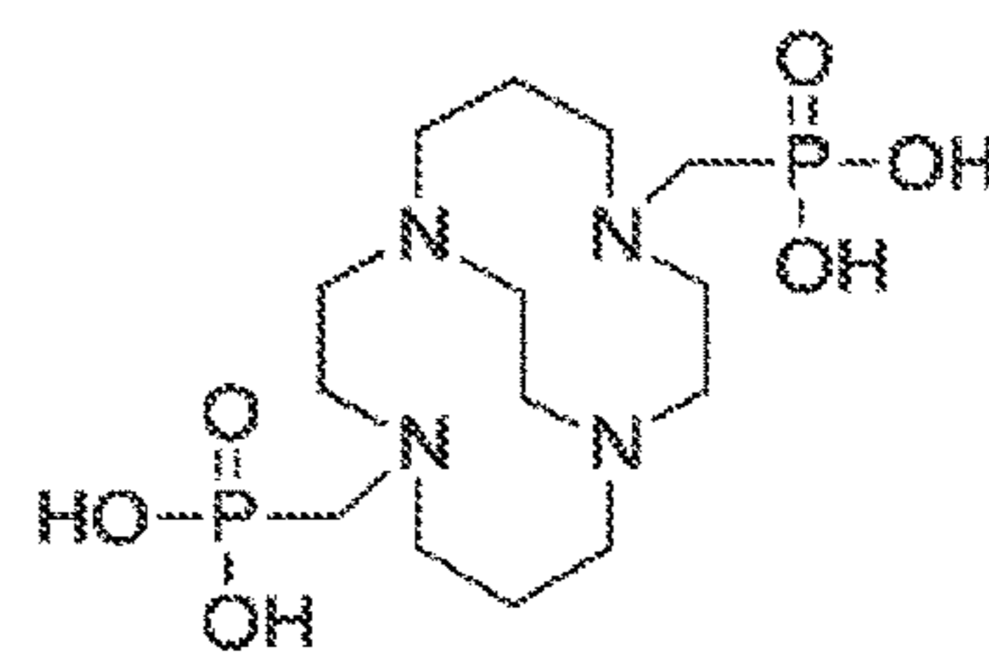
CB-TE2P
