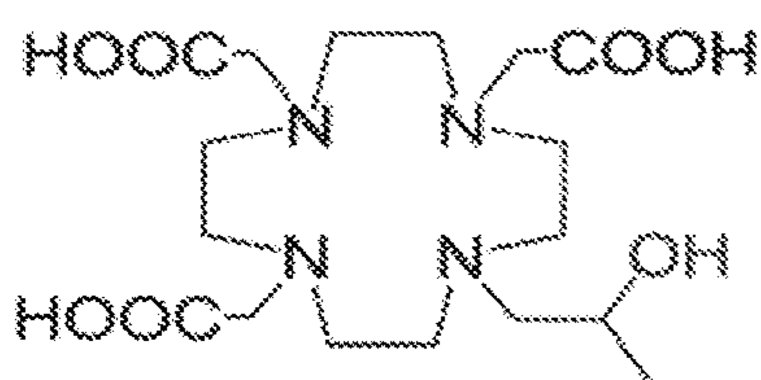
H 3 HP-DO3A
