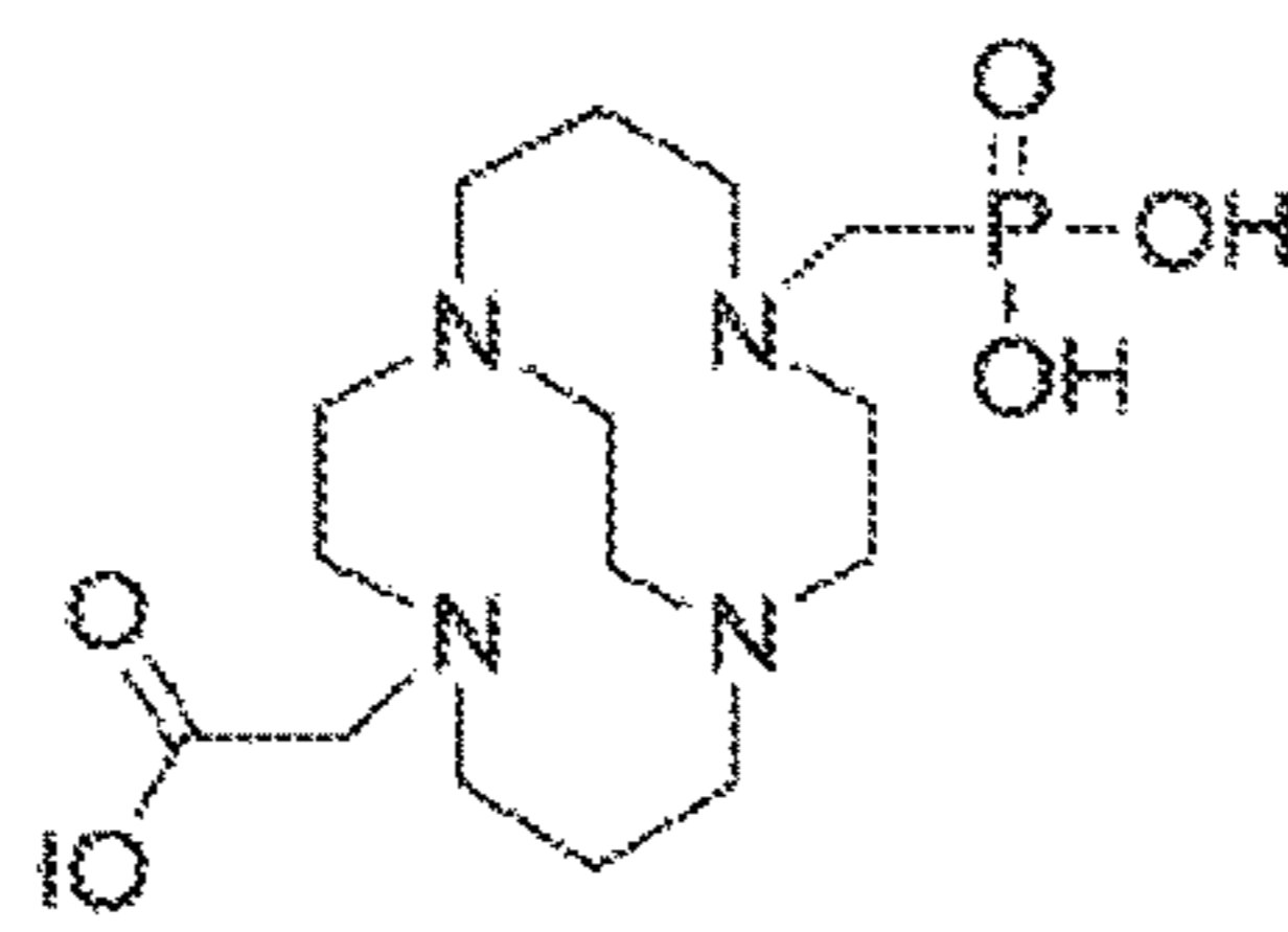
CB-TE1A1P
