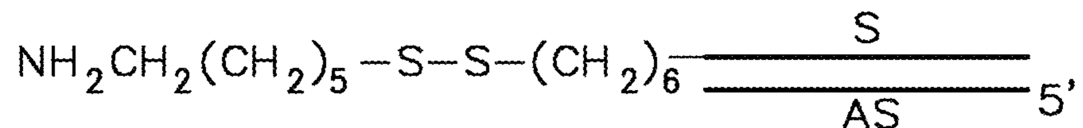
FIG. 17A
