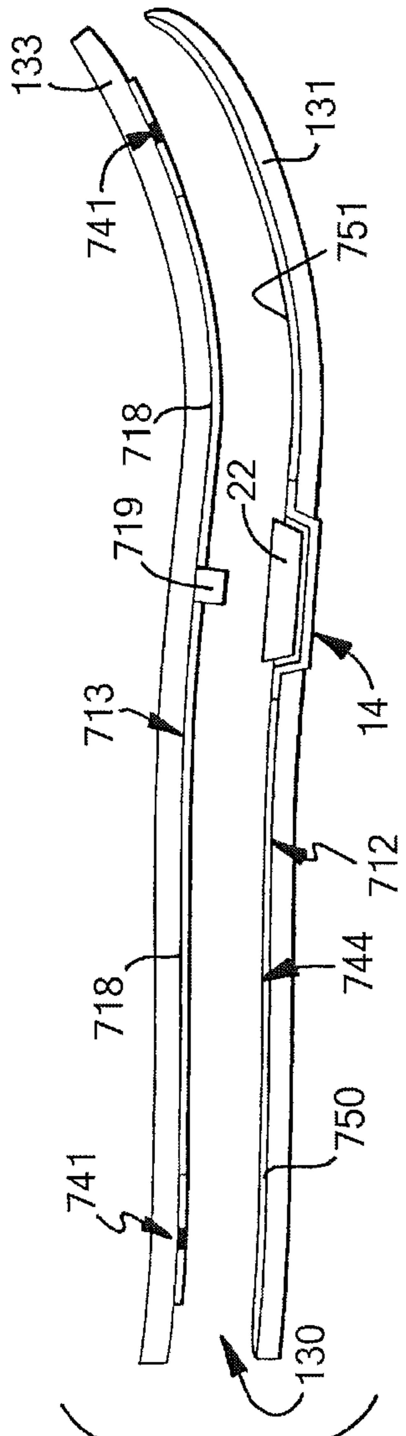
FIG. 16
