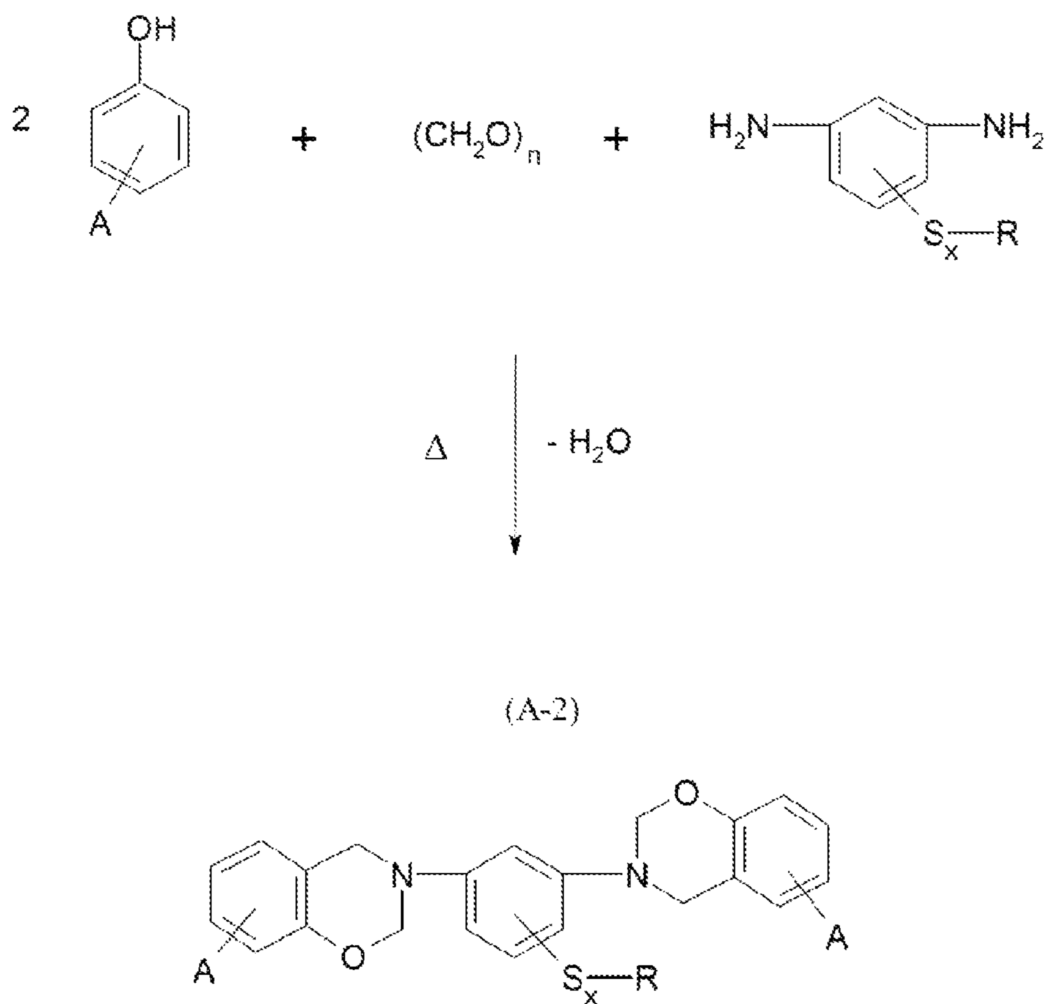
Monomer M-2
