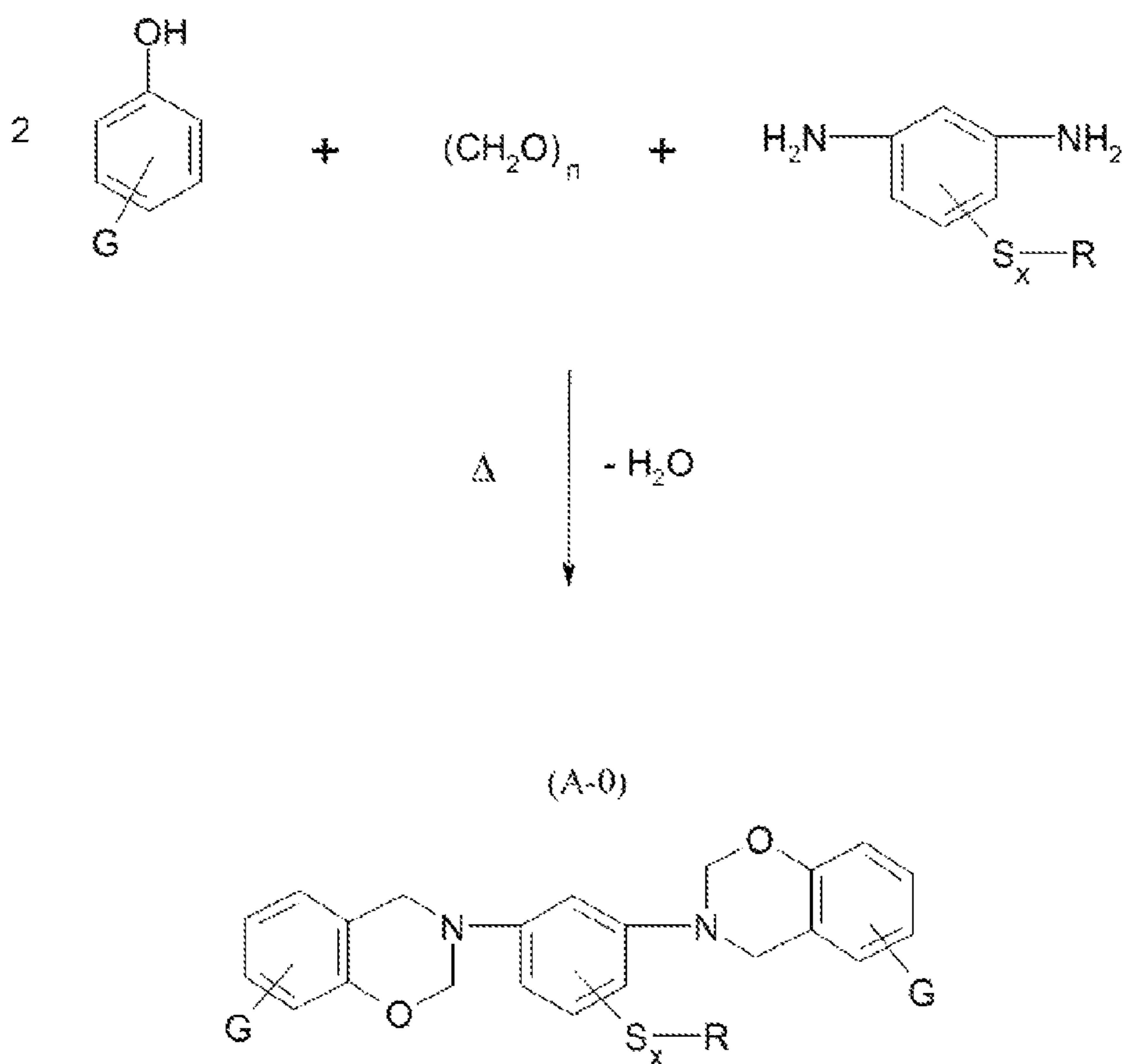
Monomer M-0
