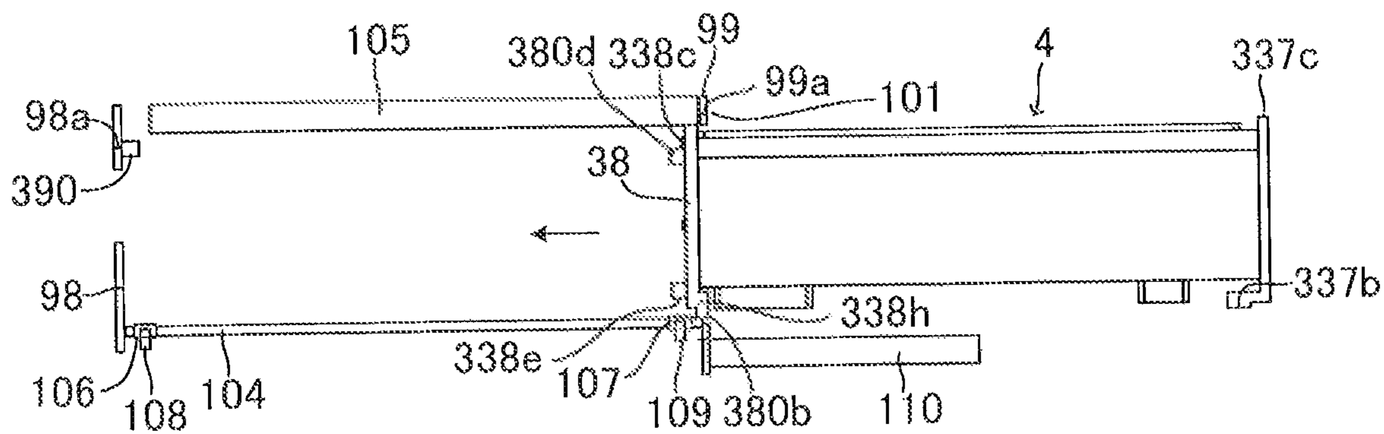
FIG.27A
