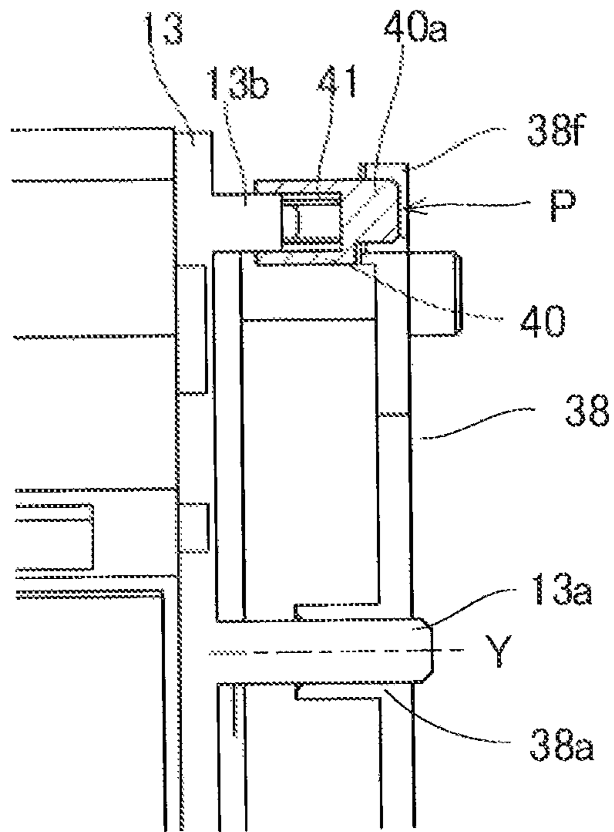
FIG. 9A
