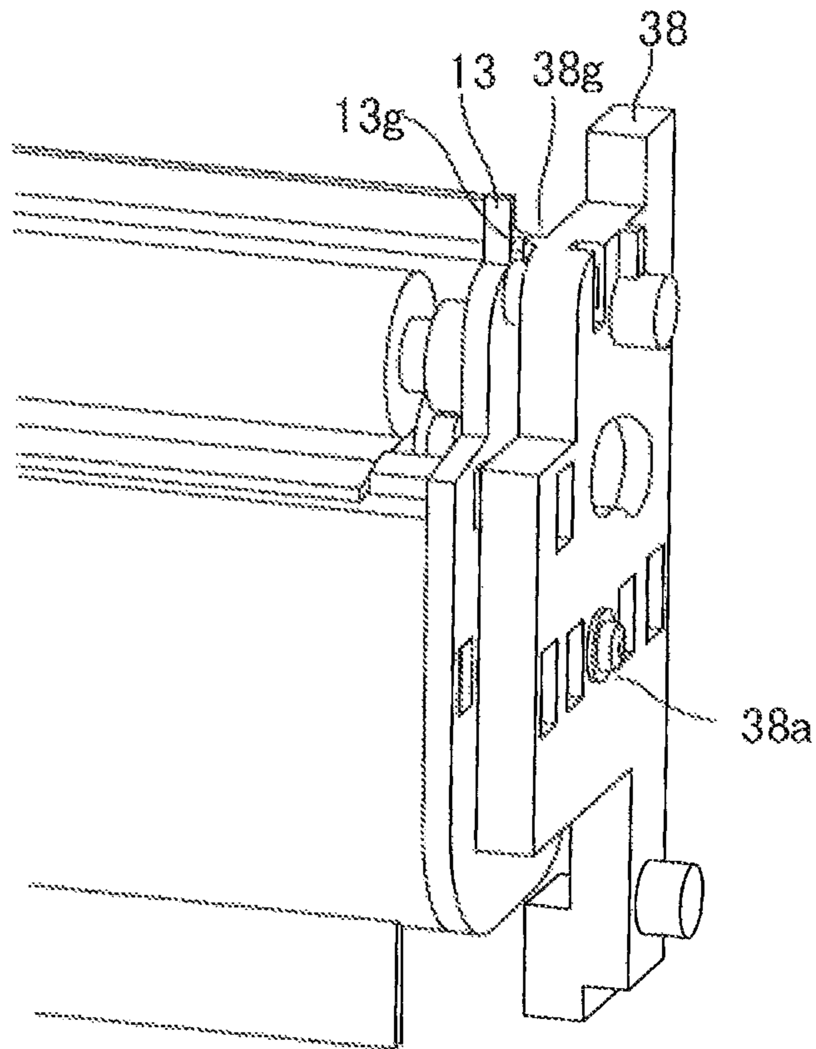
FIG. 18A
