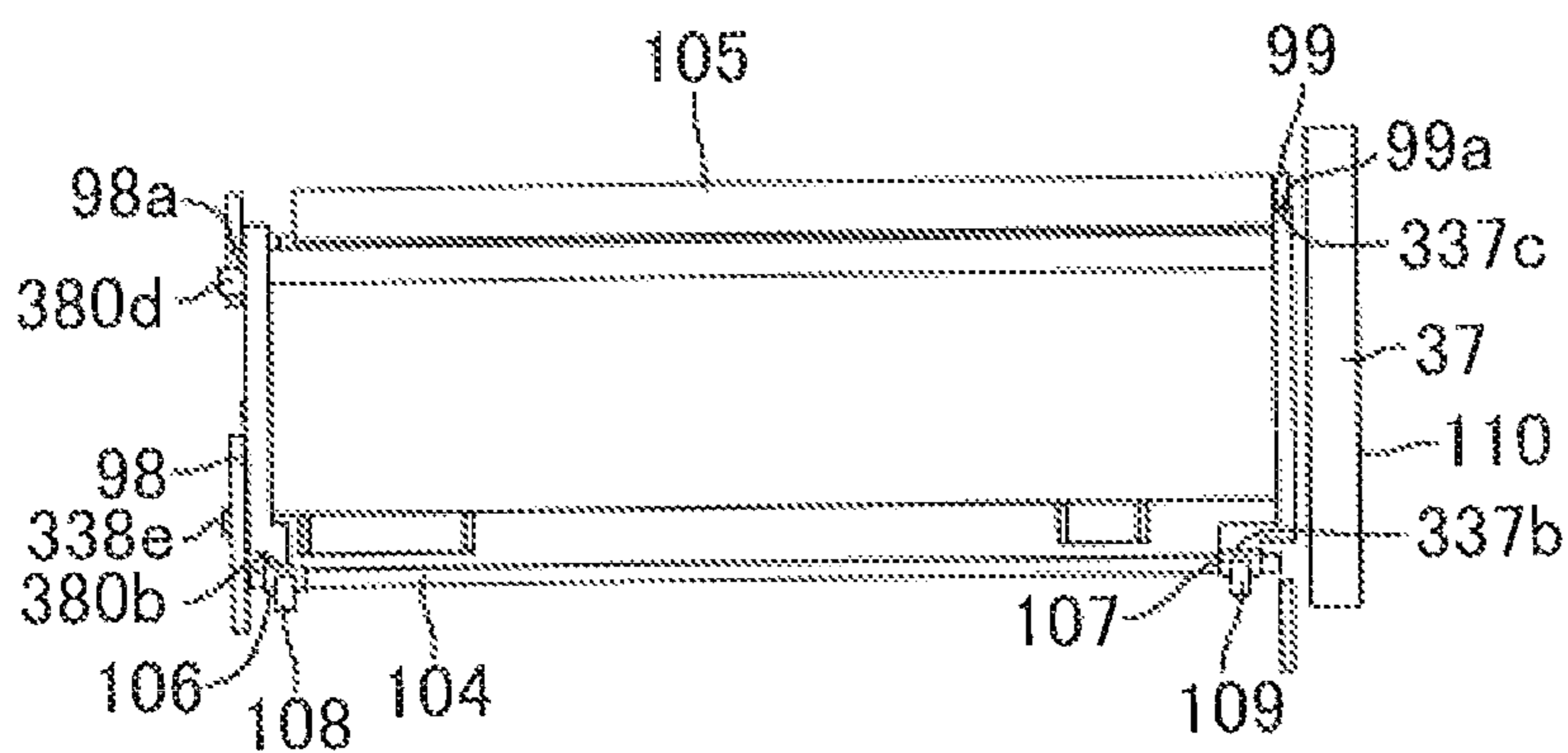
FIG.27C
