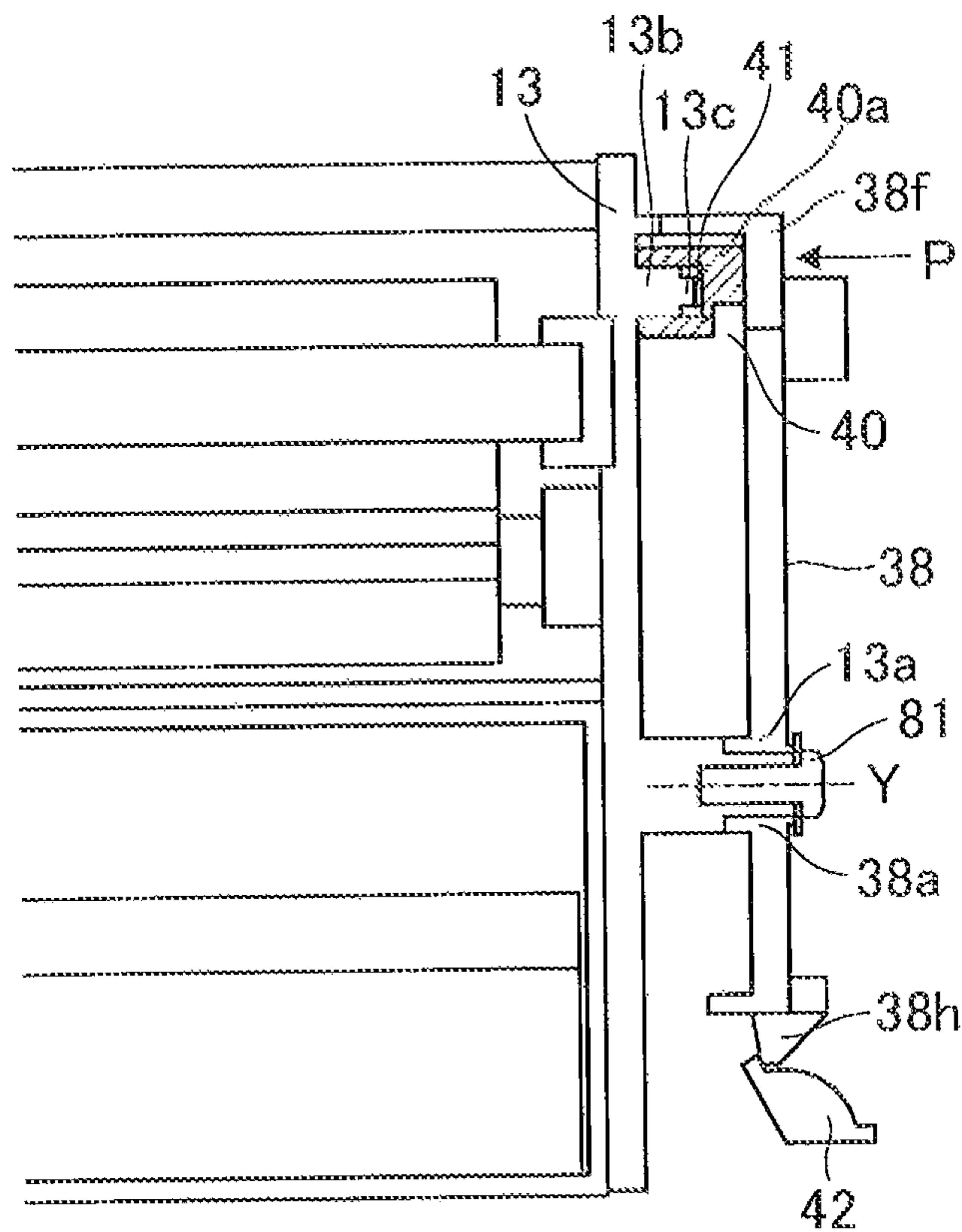
FIG. 21B
