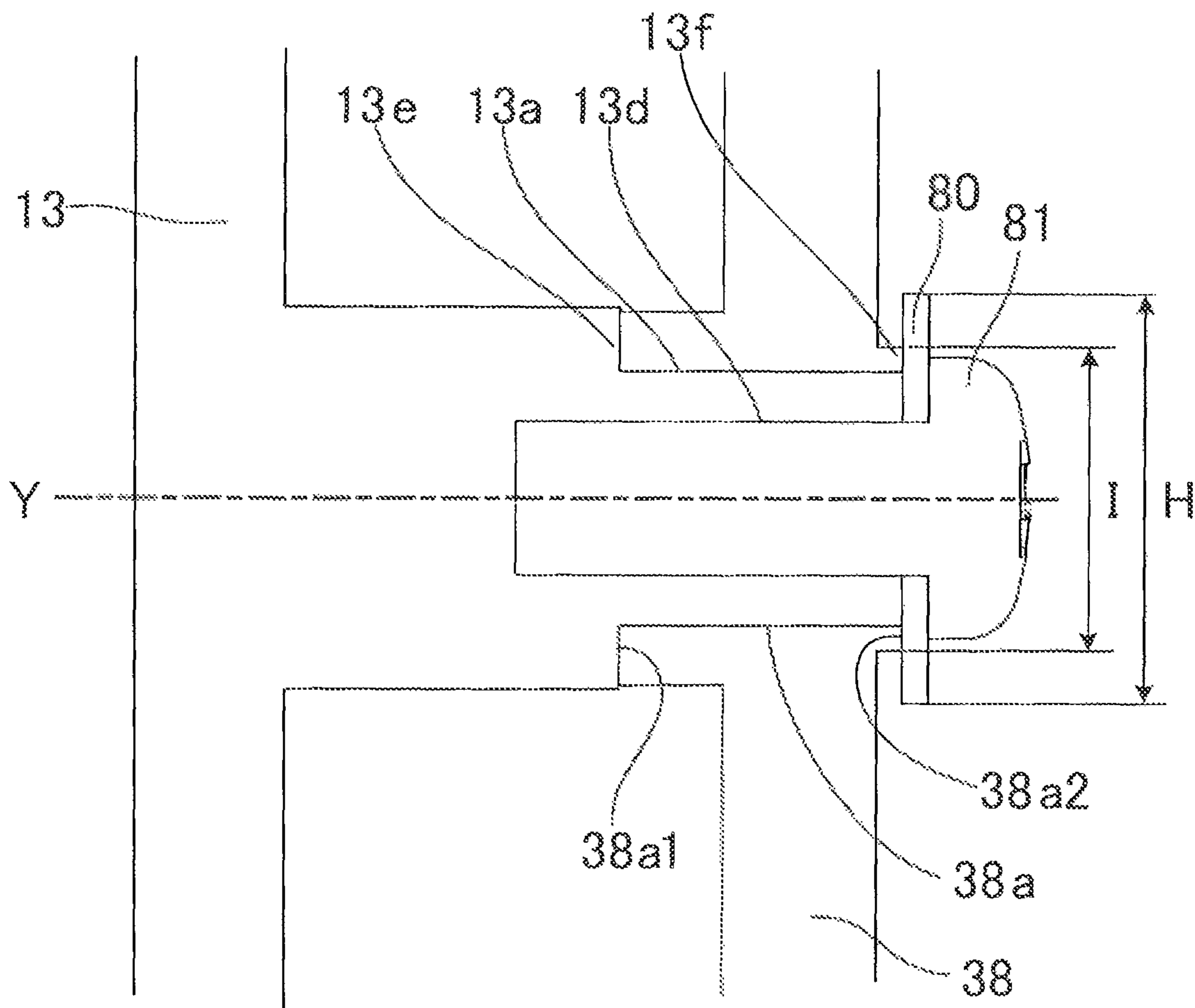
FIG. 19
