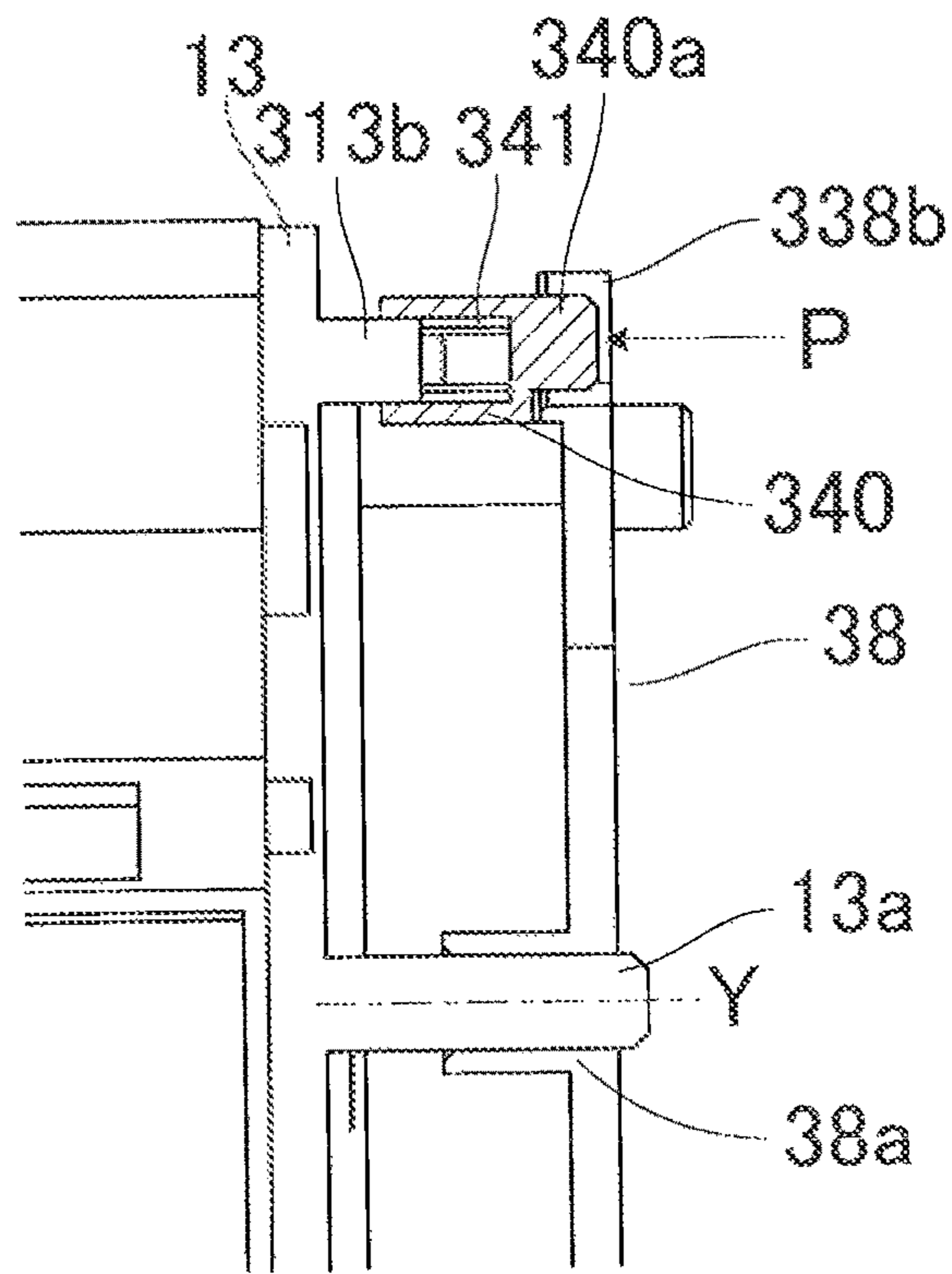
FIG. 25A
