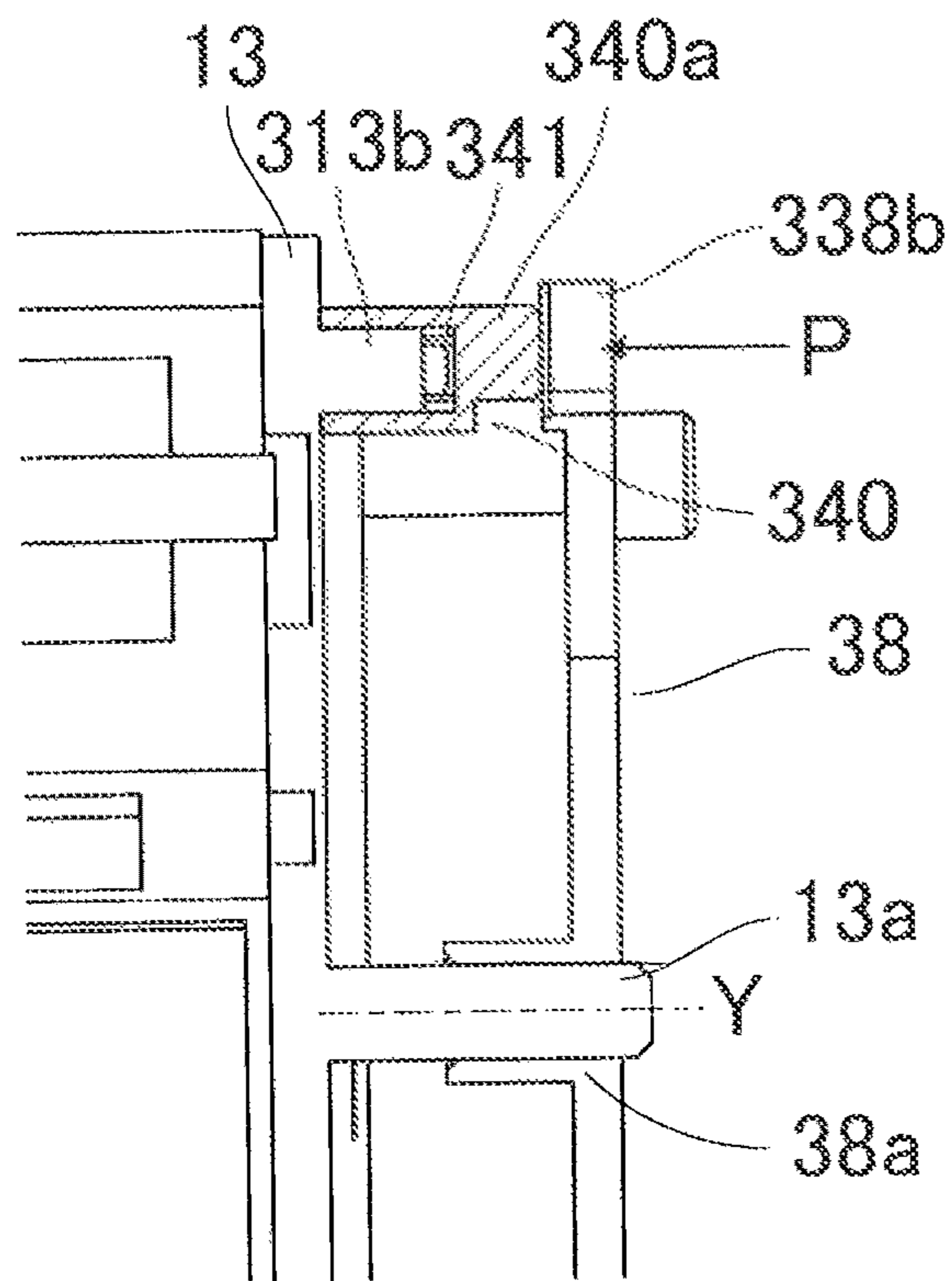
FIG. 25B
