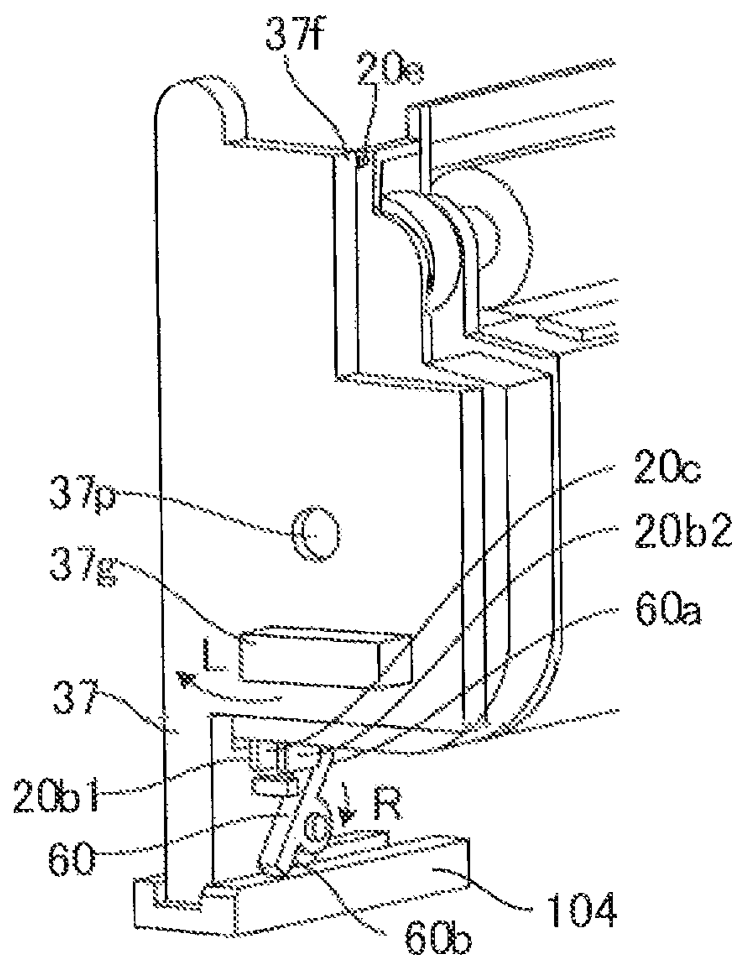
FIG. 17B
