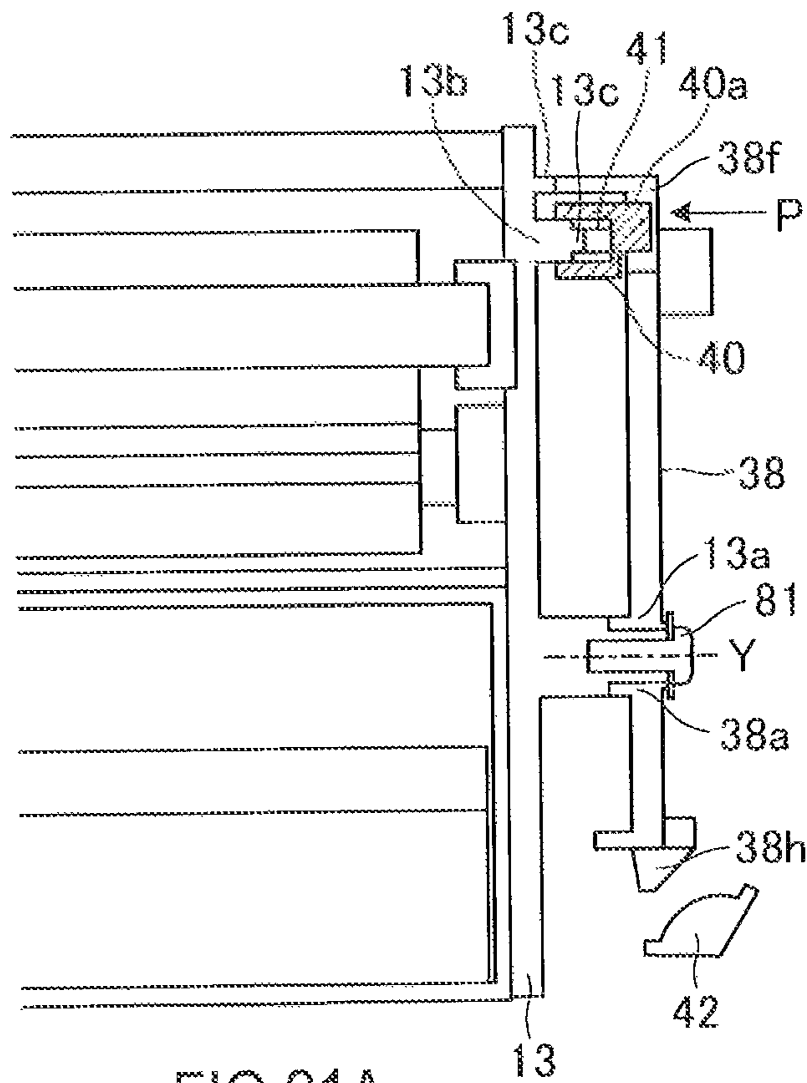
FIG. 21A
