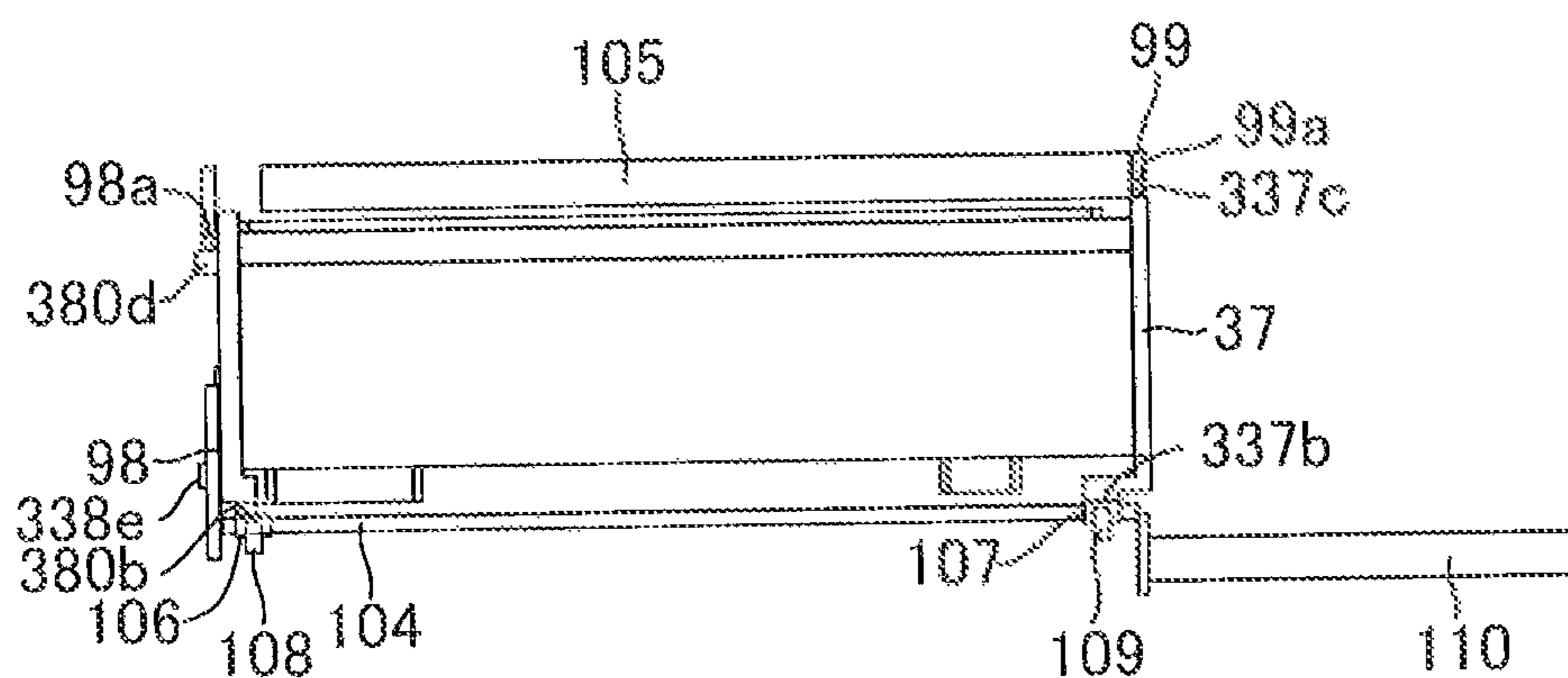
FIG.27B
