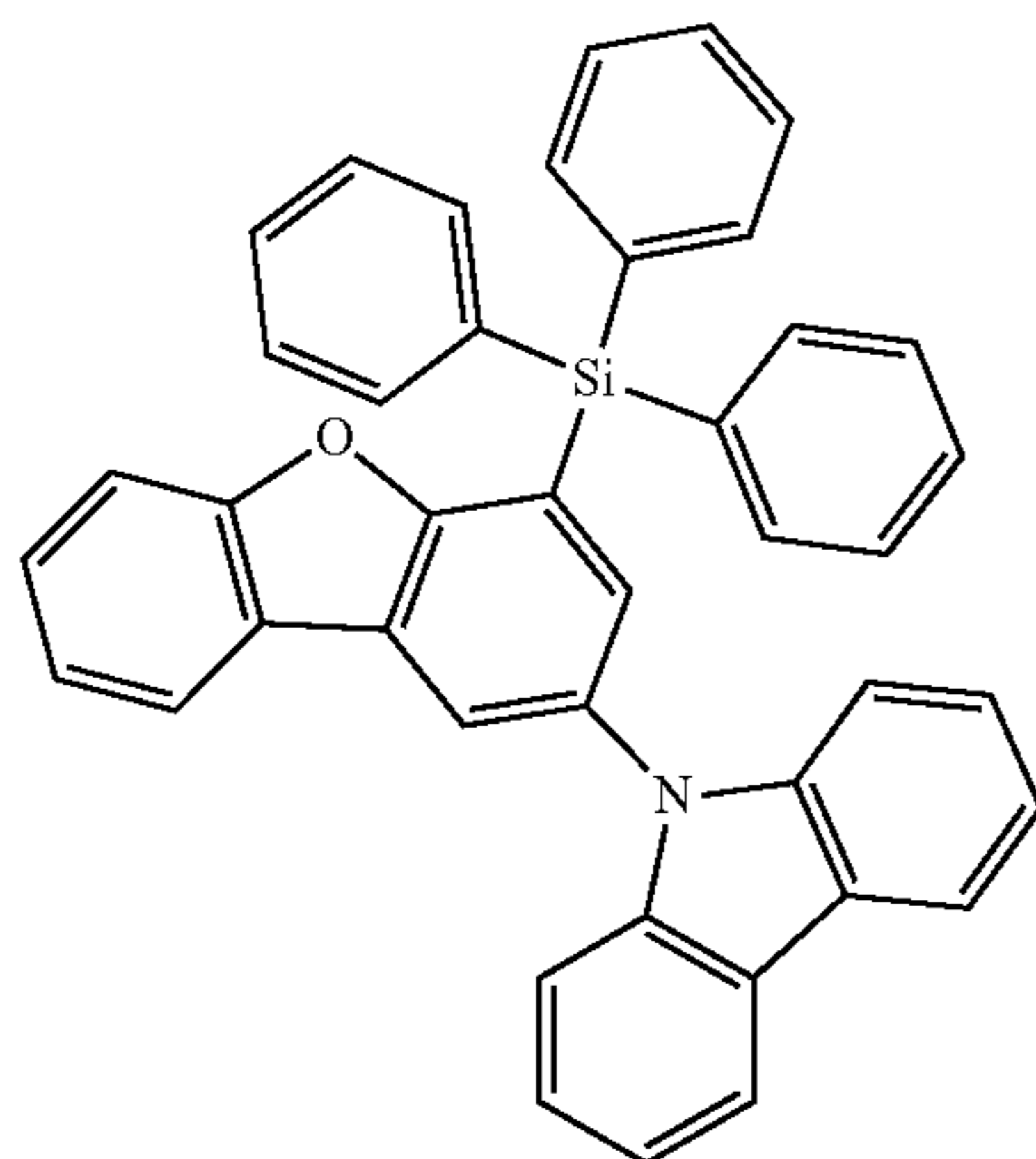
HTH4
