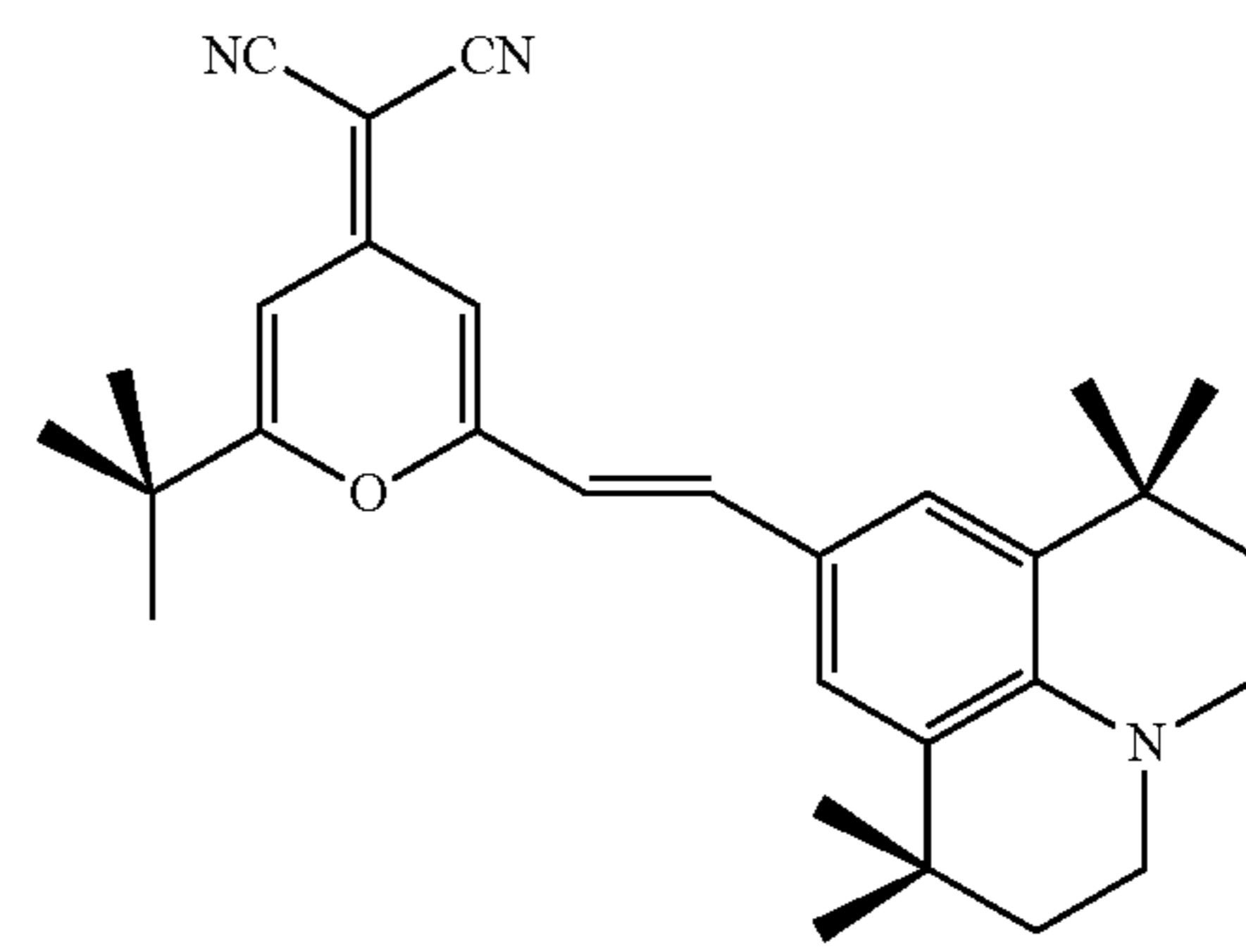
DCJTb
