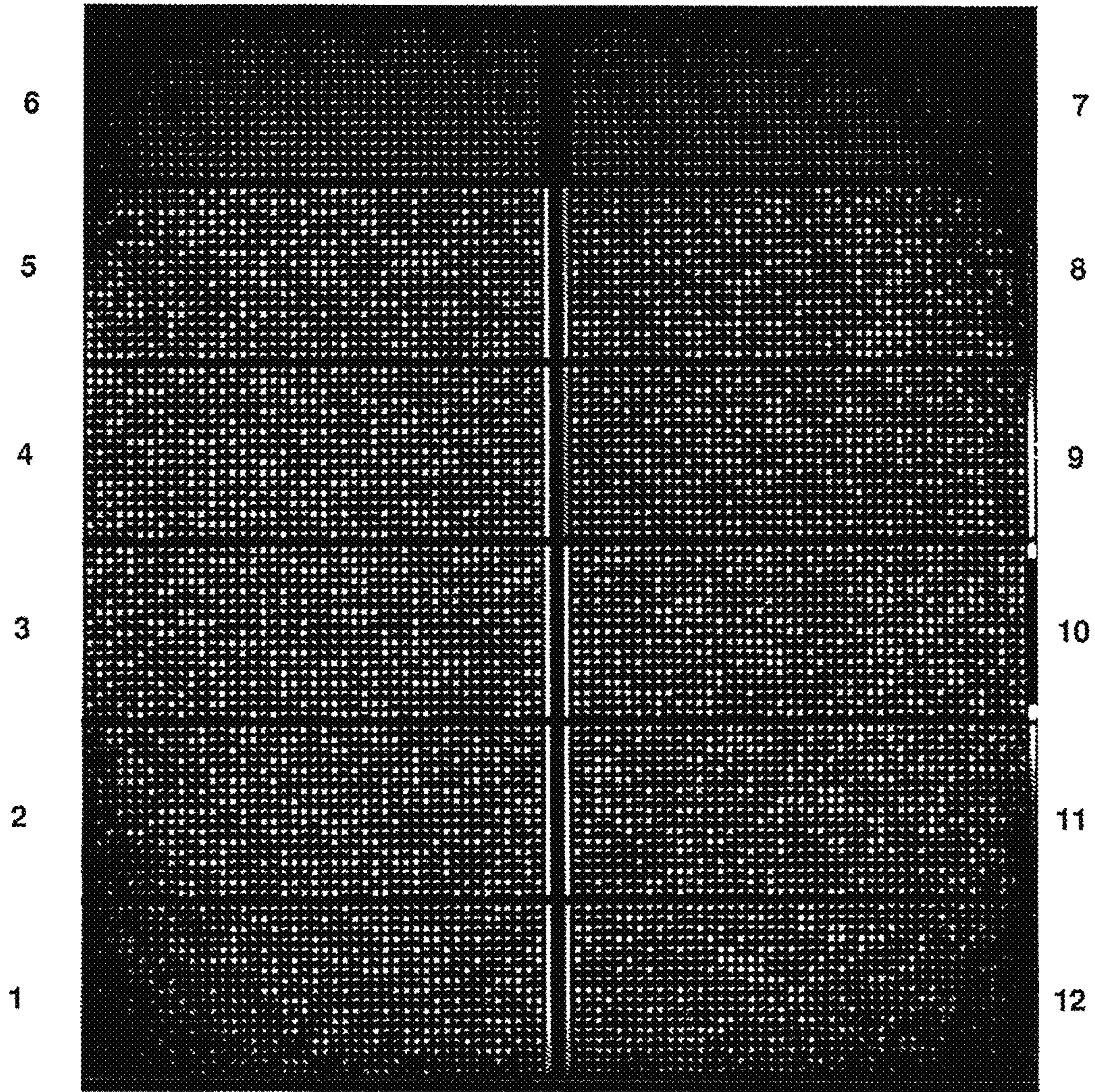
Chr 12 HEX
