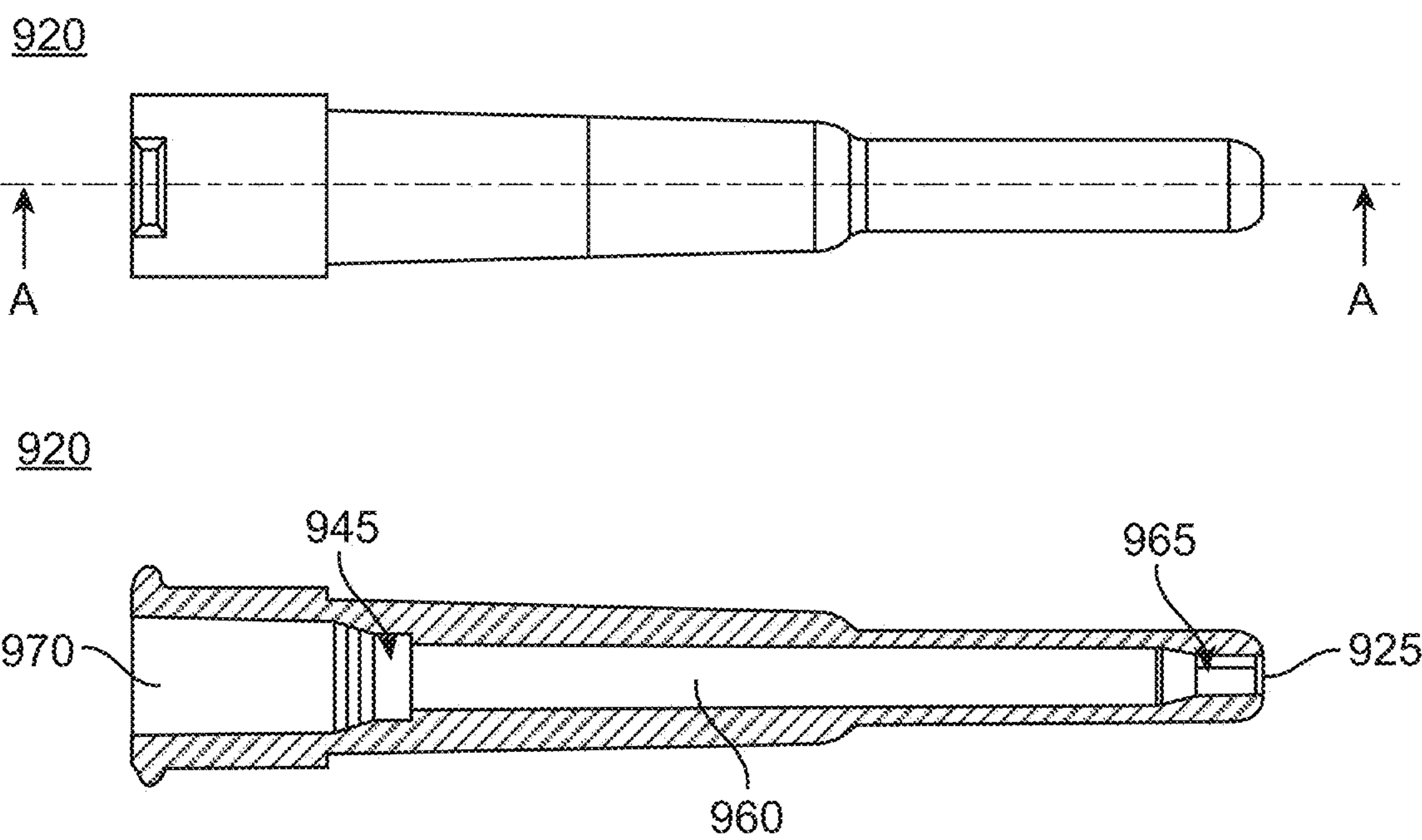
SECTION A-A
