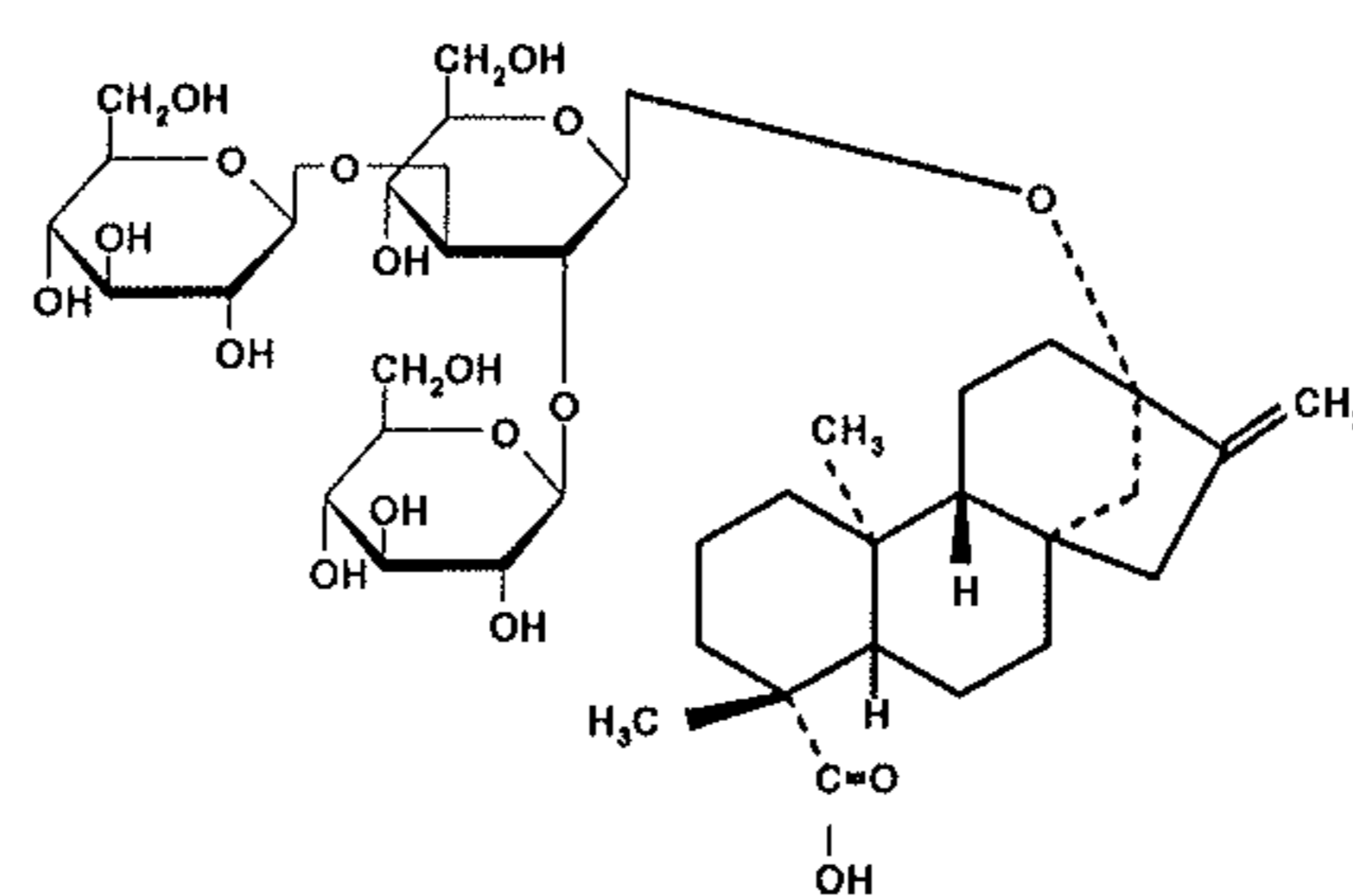
Rebaudioside B
