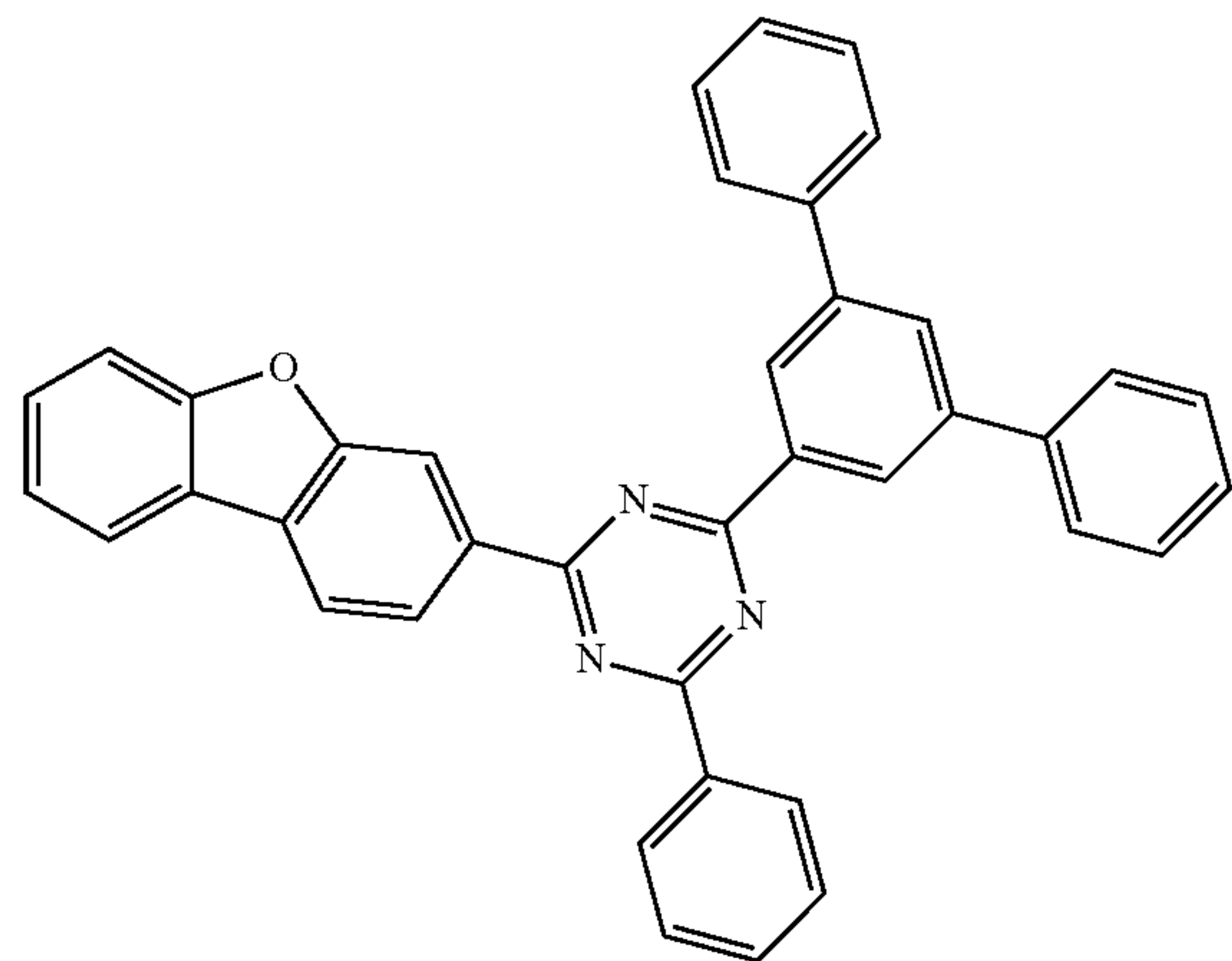
[B-2]
