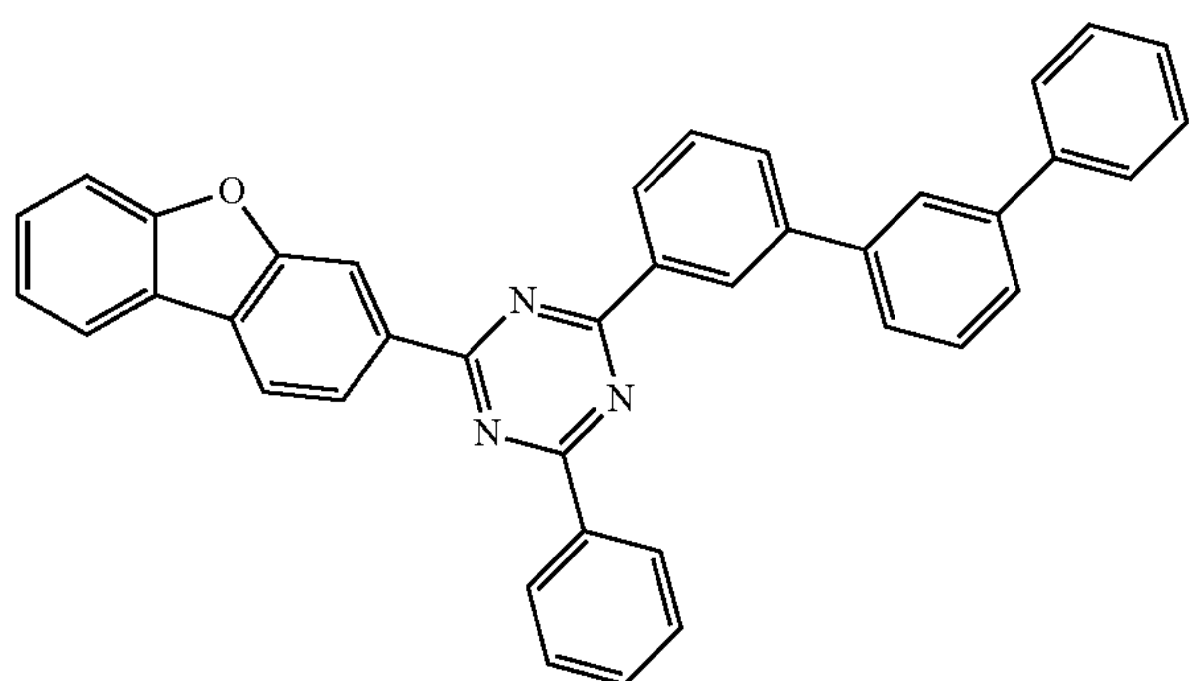
[B-2]
