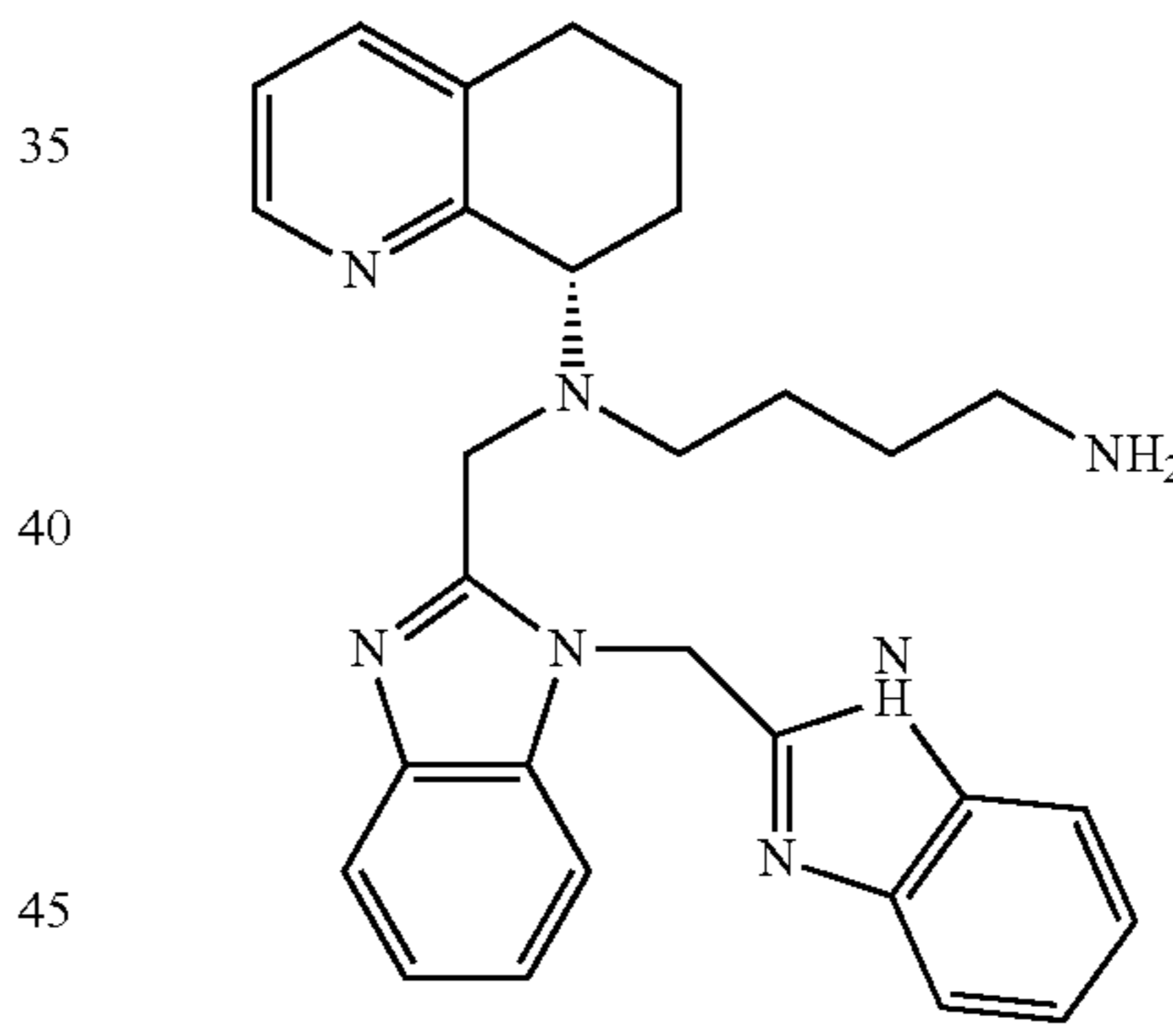
benzimidazole E
