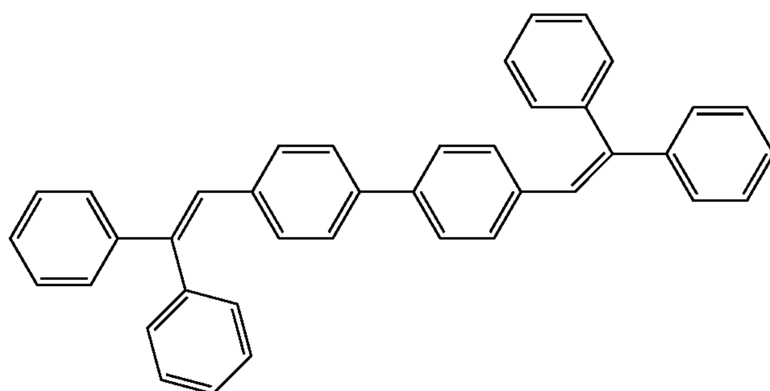
DPVBi
