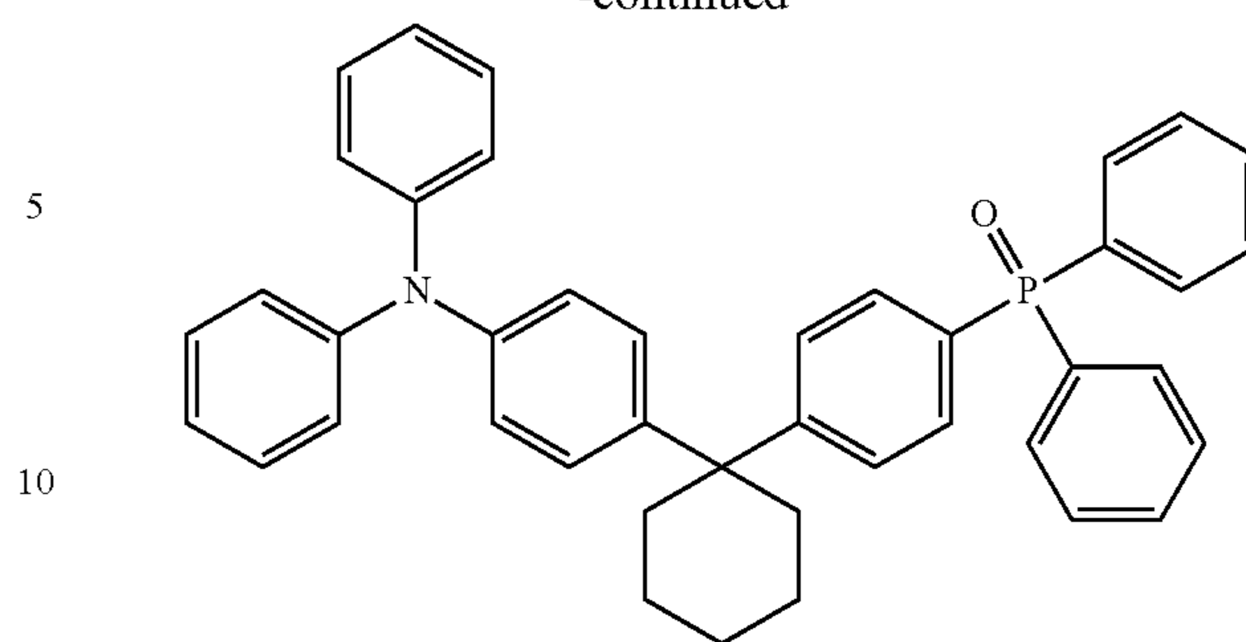
POPCPA
