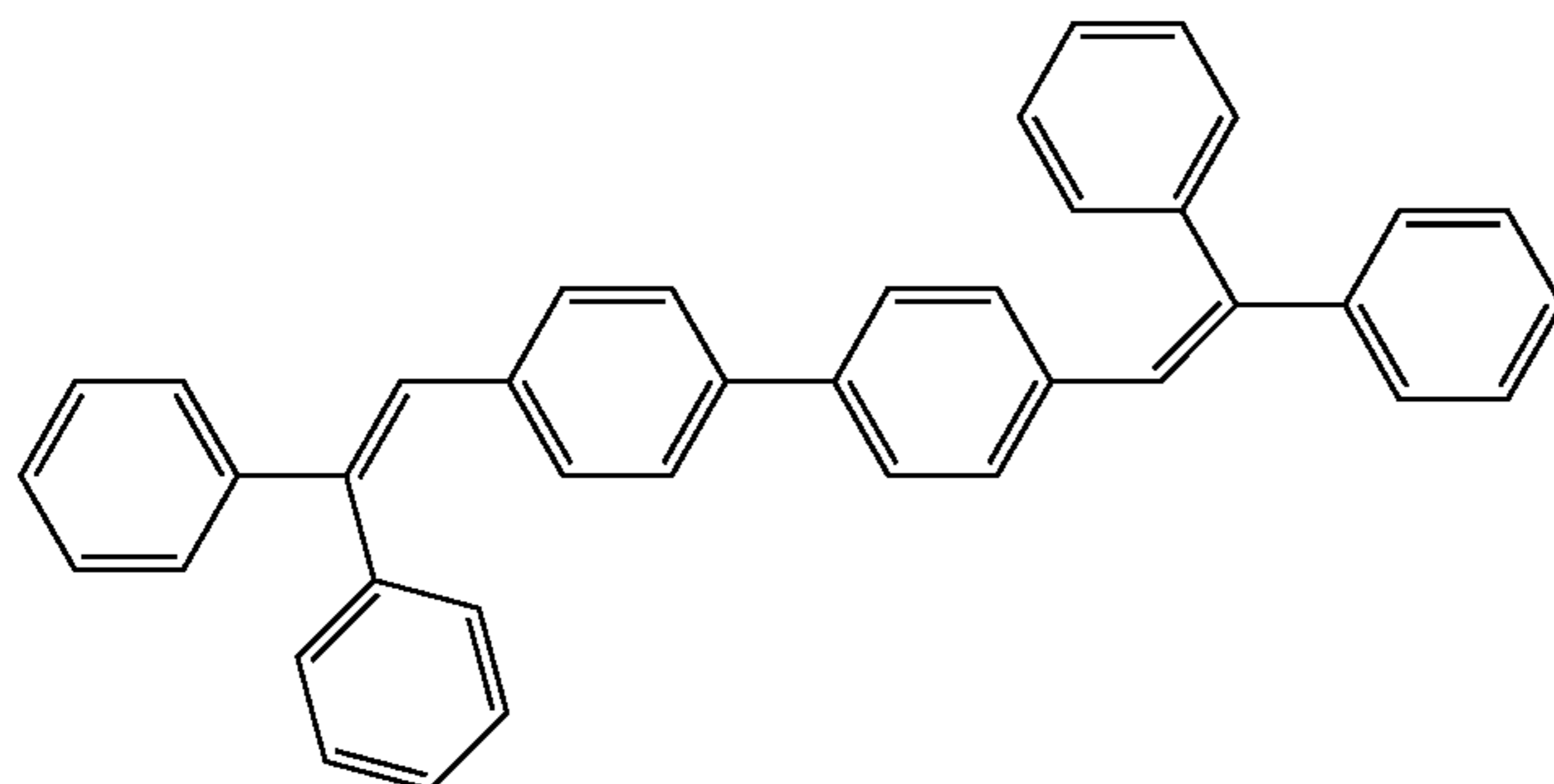
DPVBi
