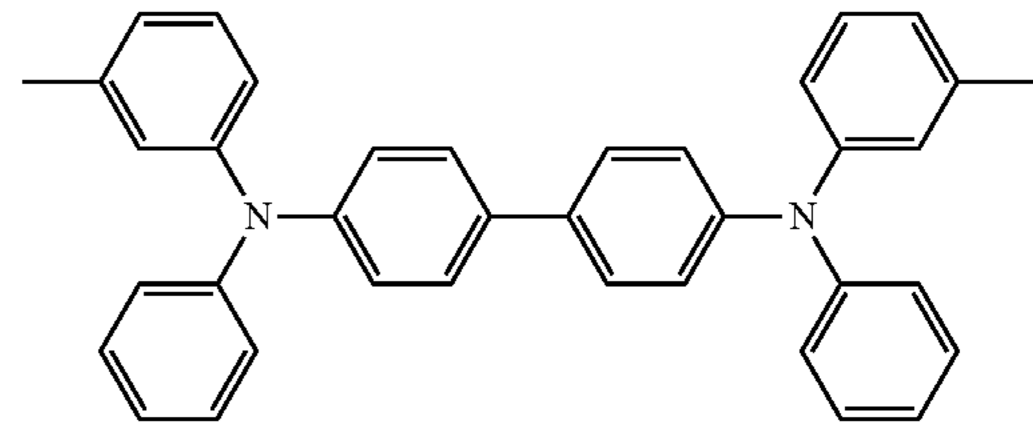
TPD
