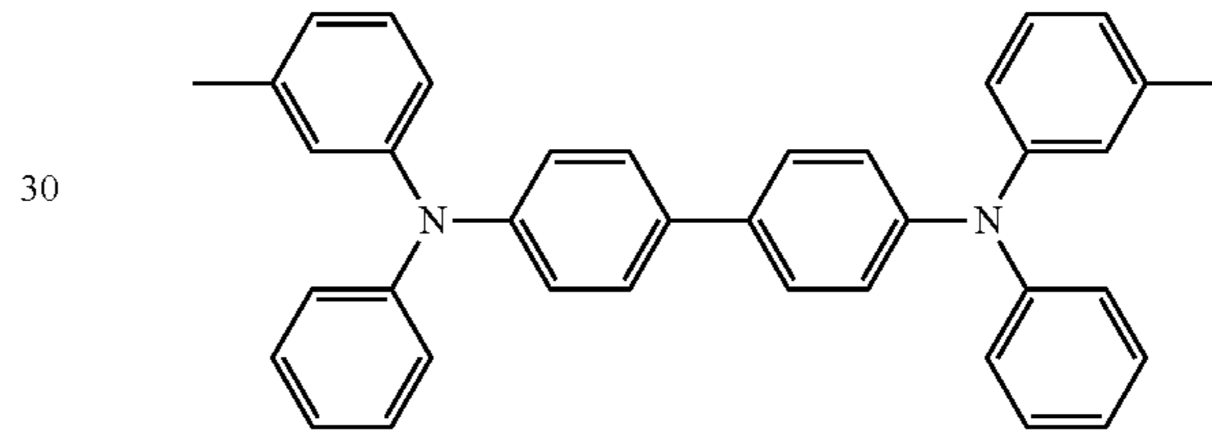
TPD
