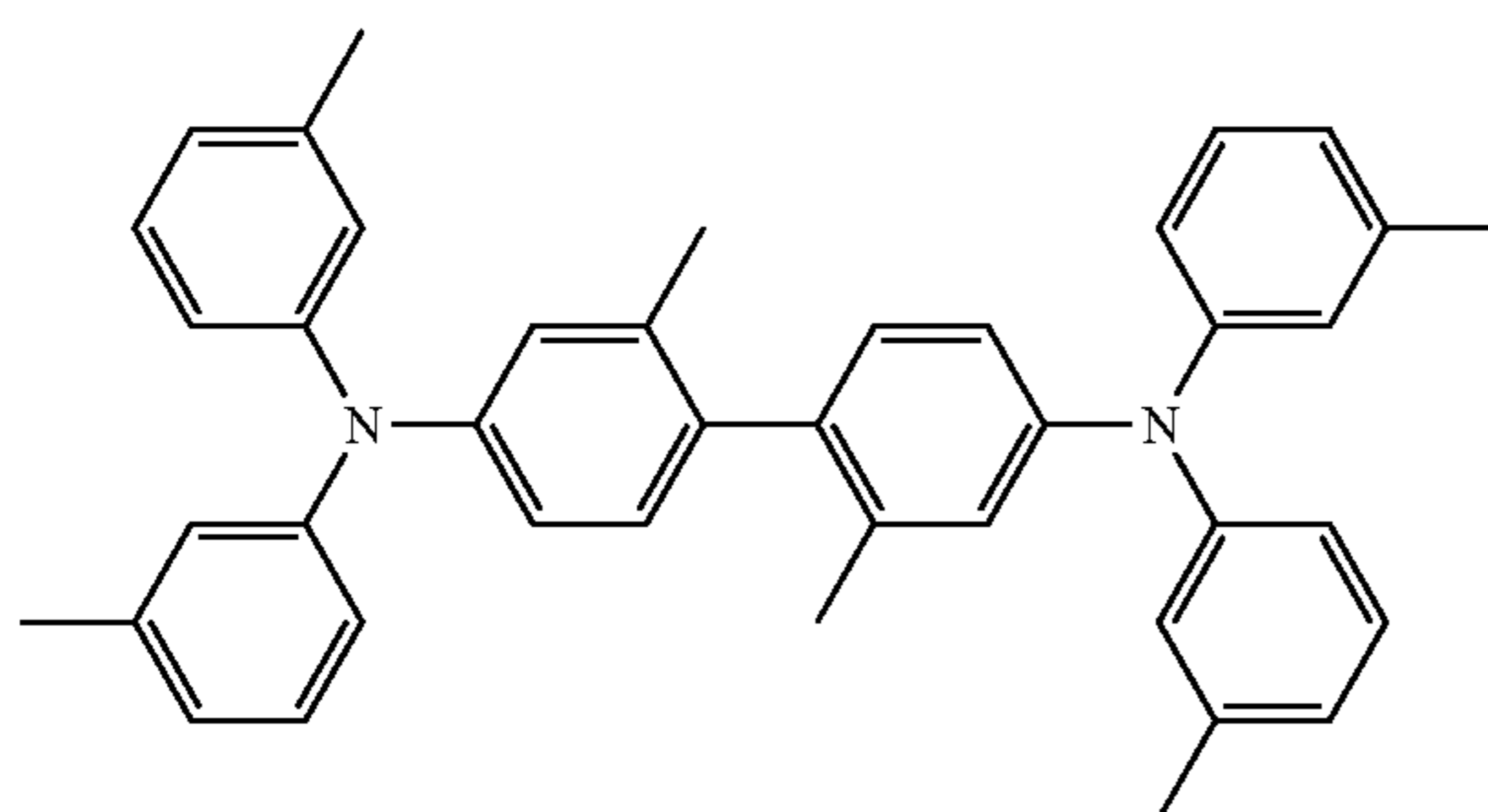
HMTPD
