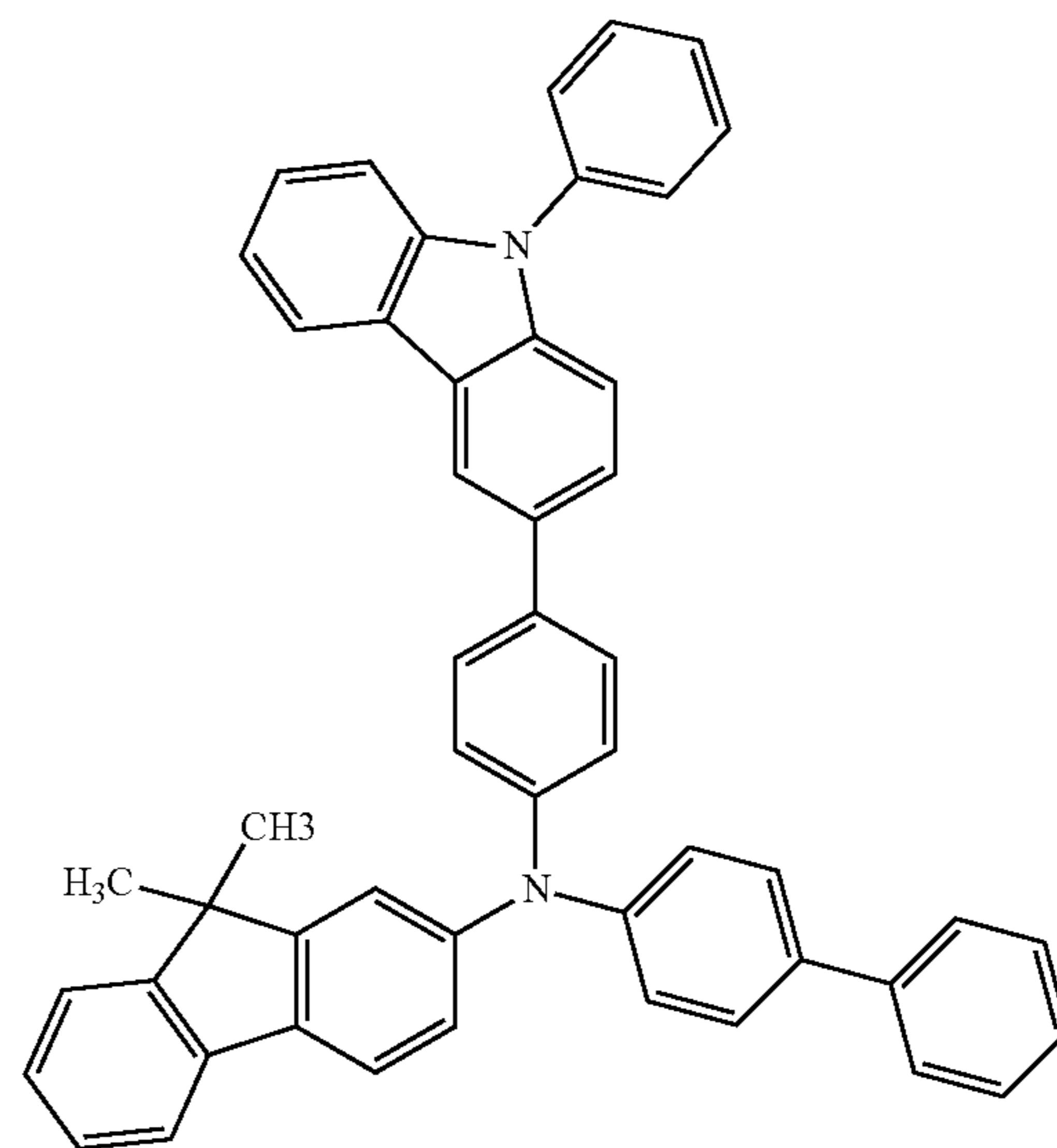
PCBBiF
