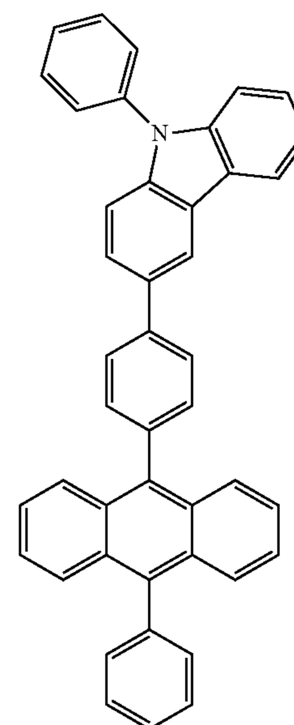
PCzPA
