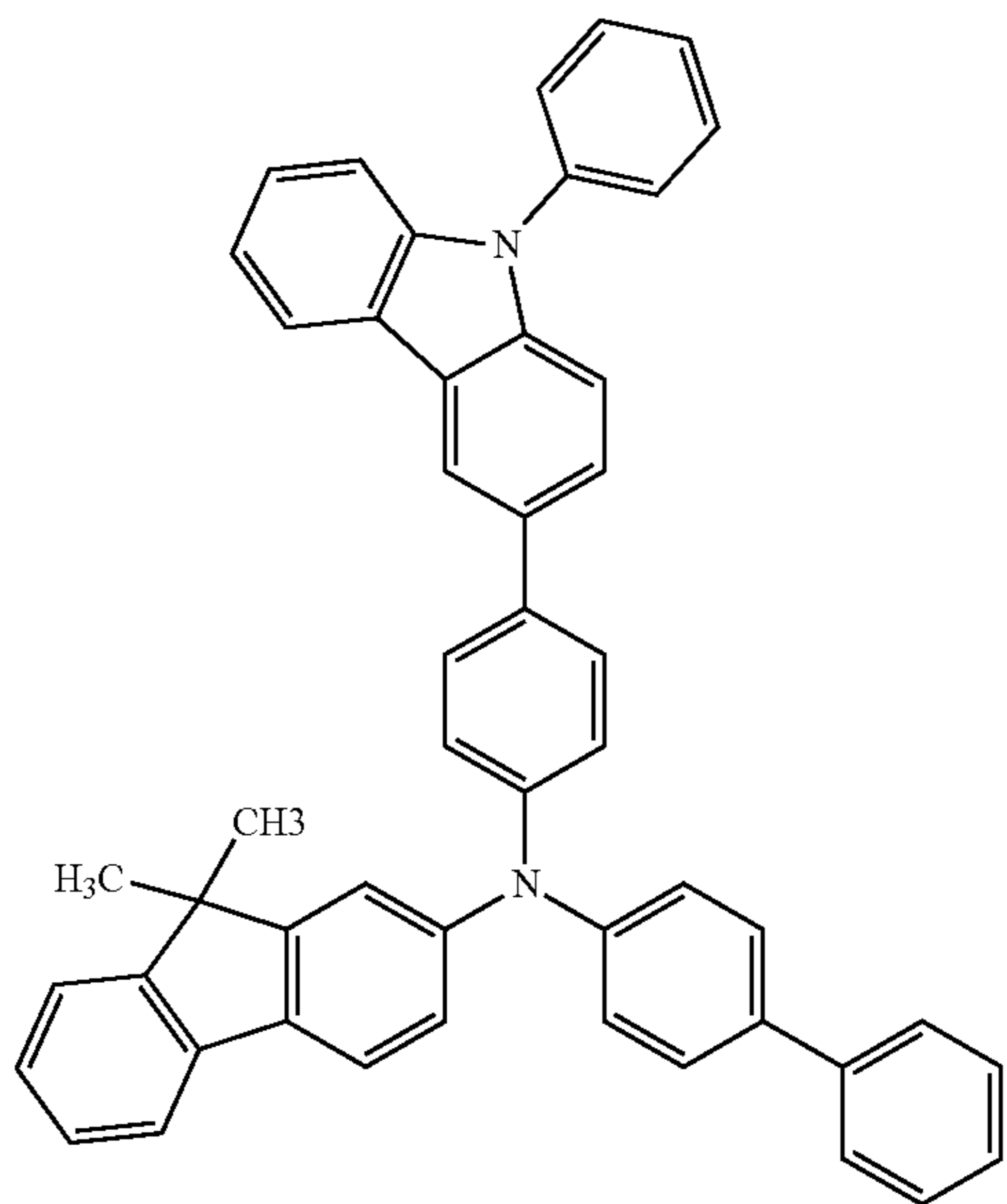
PCBBiF
