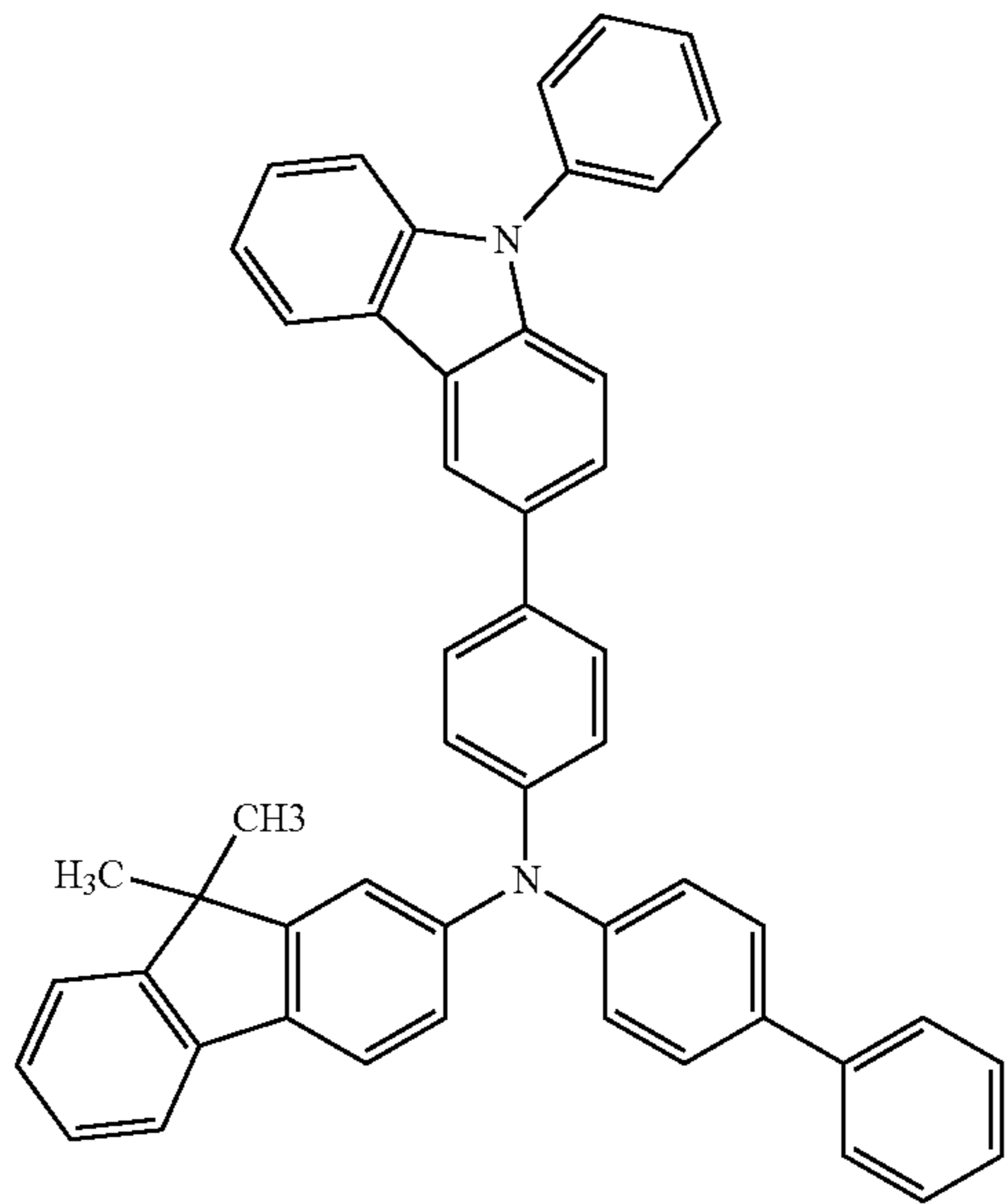
PCBBiF
