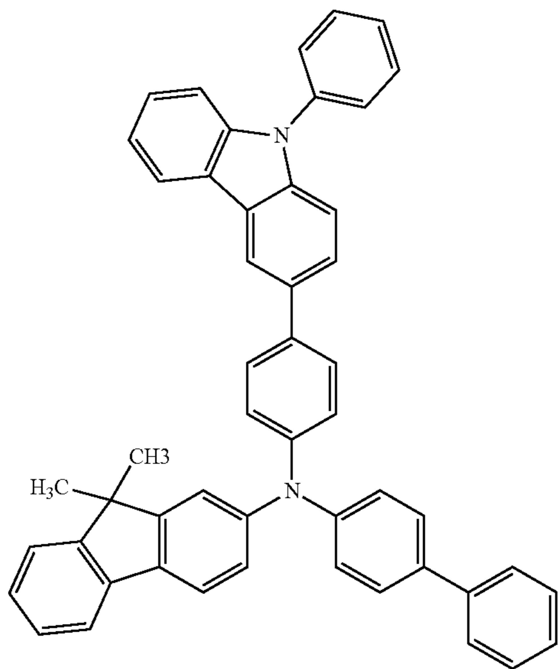
PCBBiF
