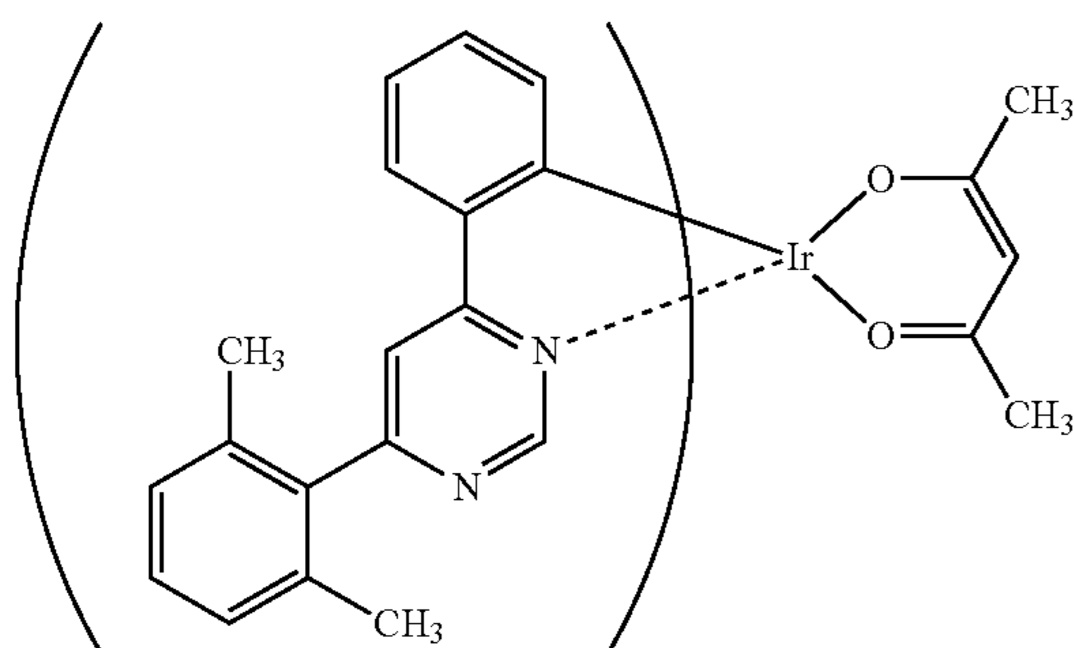
Ir(ppm-dmp) 2 (acac)
