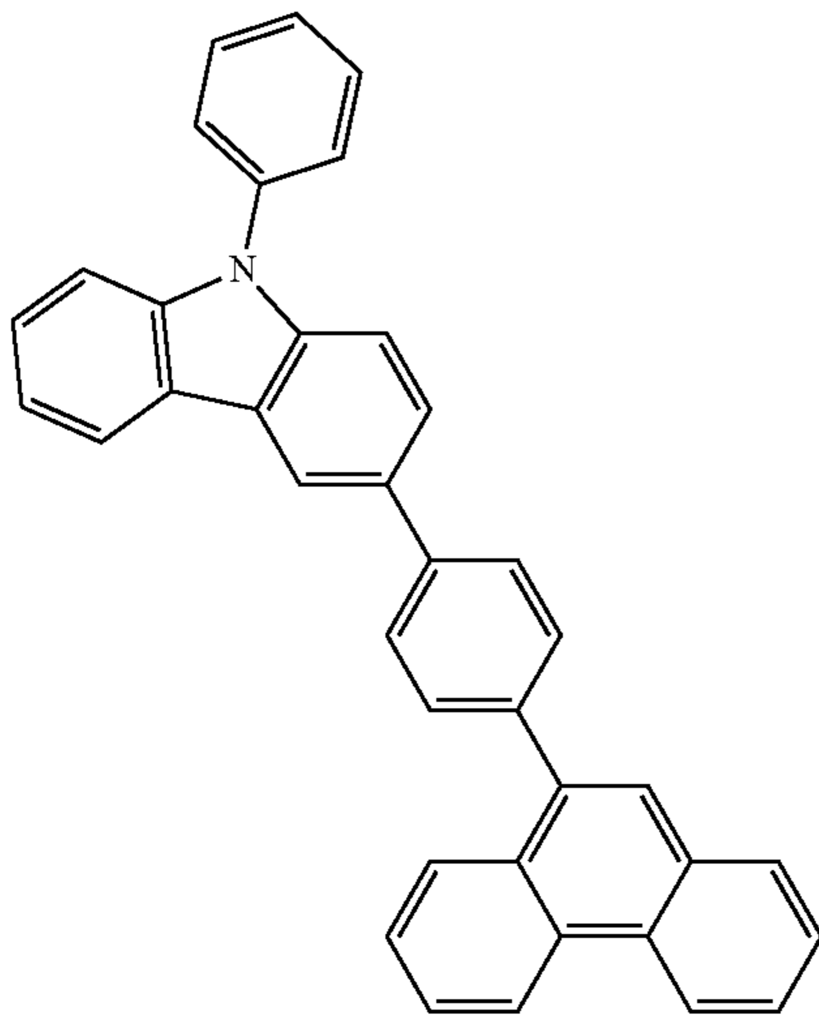
PCPPn
