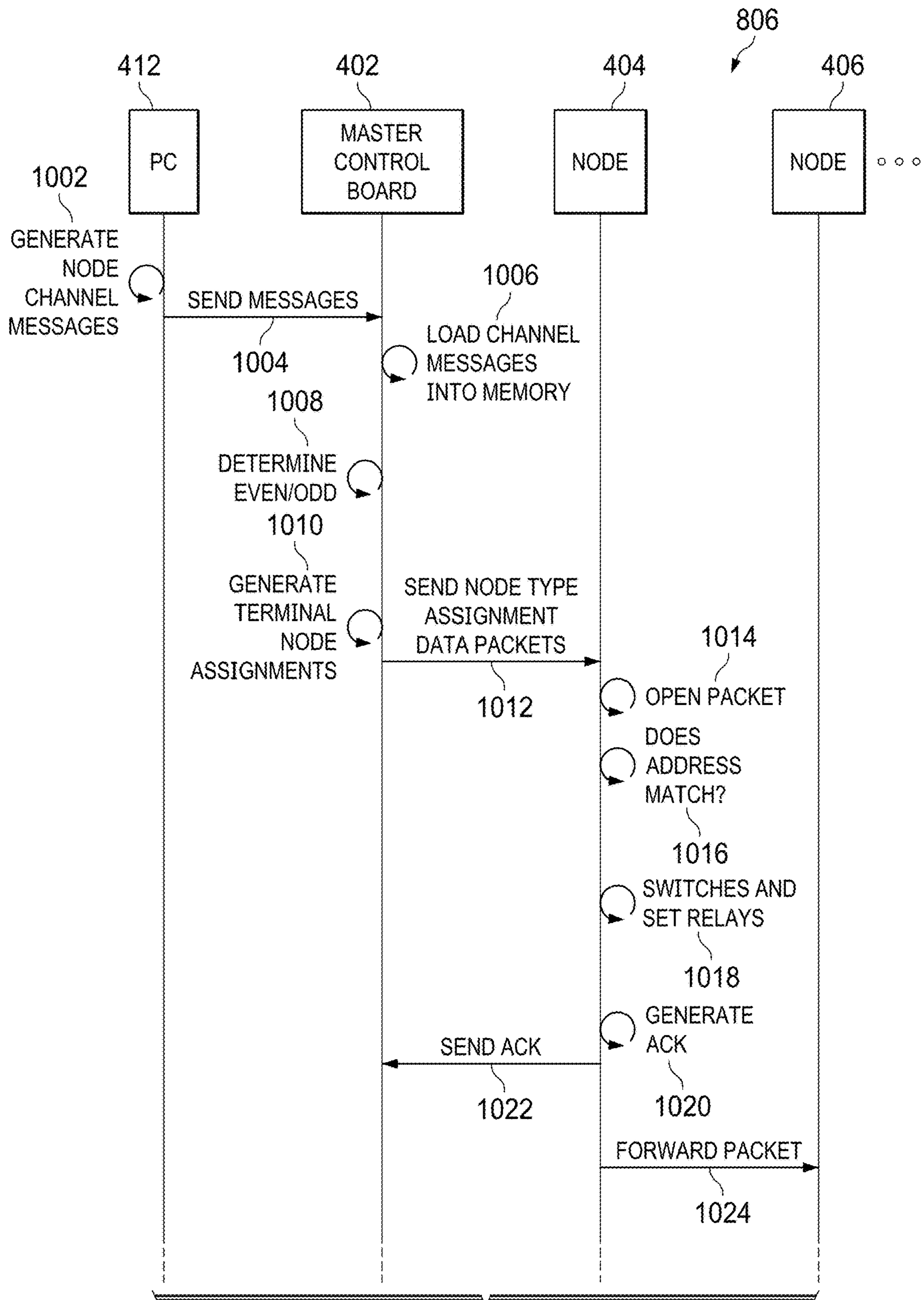
FIG. 10A
