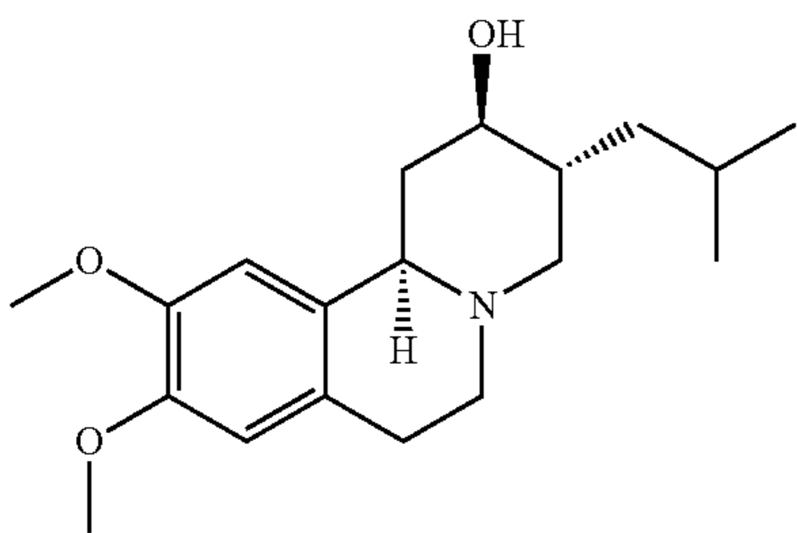
(+)-α-HTBZ
