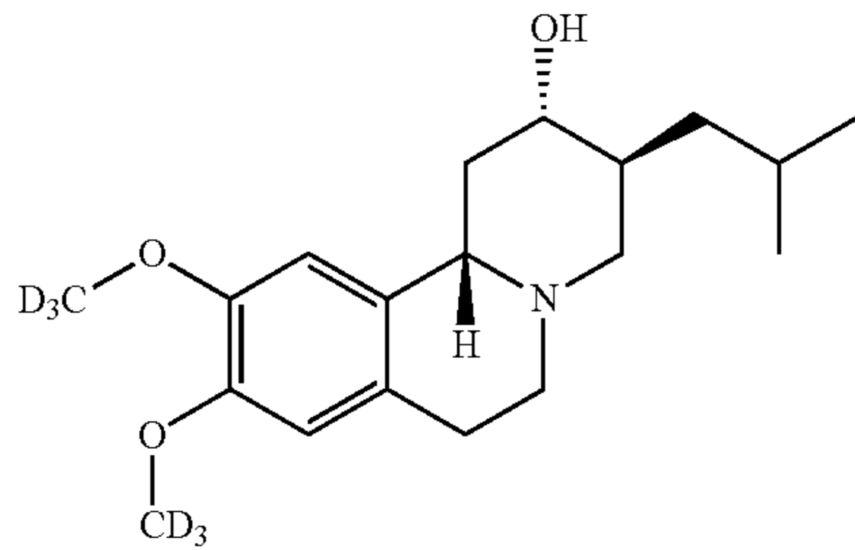
(-)-d 6 -α-HTBZ
