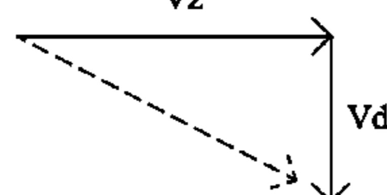
T=0
