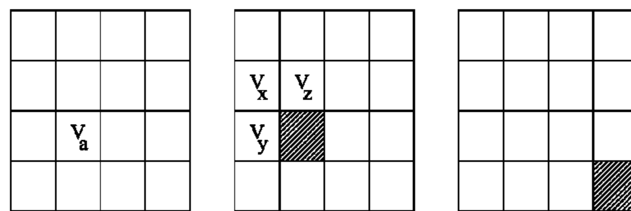
T=-1
