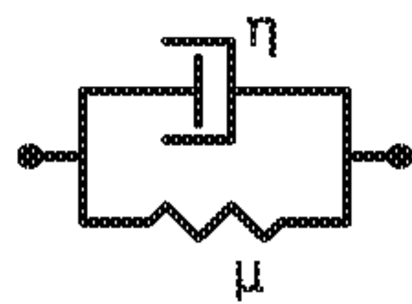
Kelvin-Voigt Model
