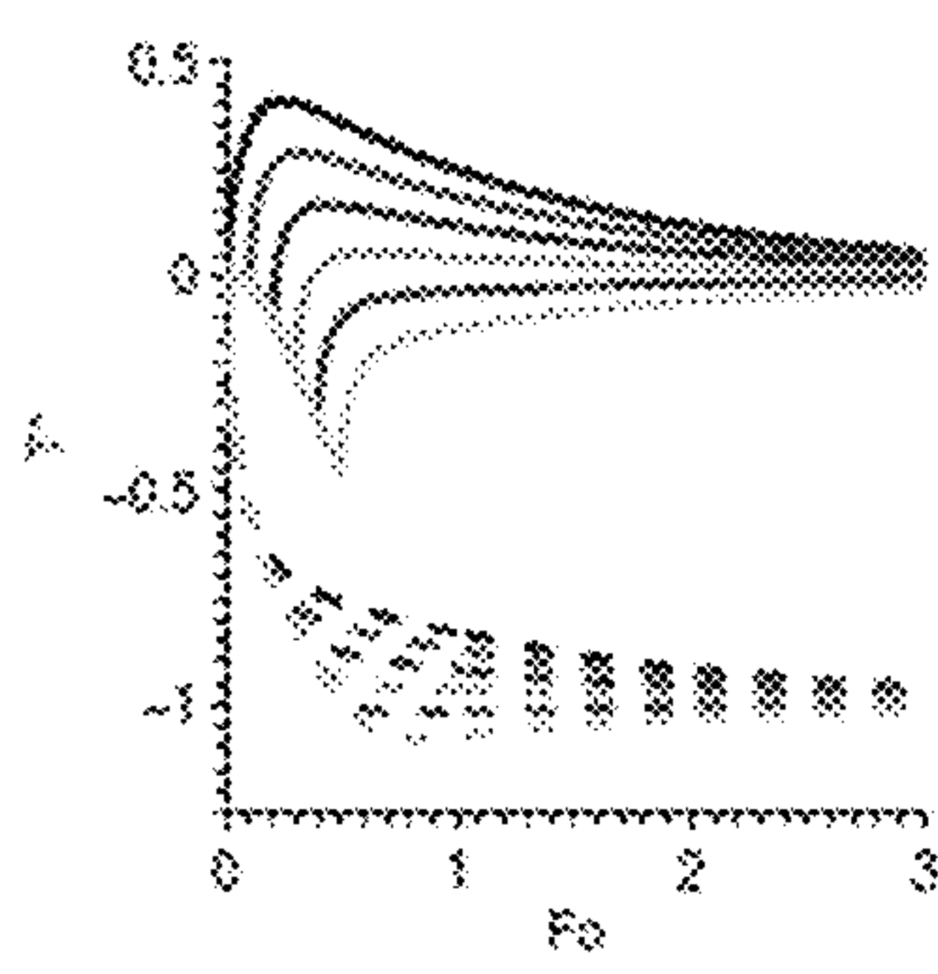
(b) Bi=1 FIG. 20B
