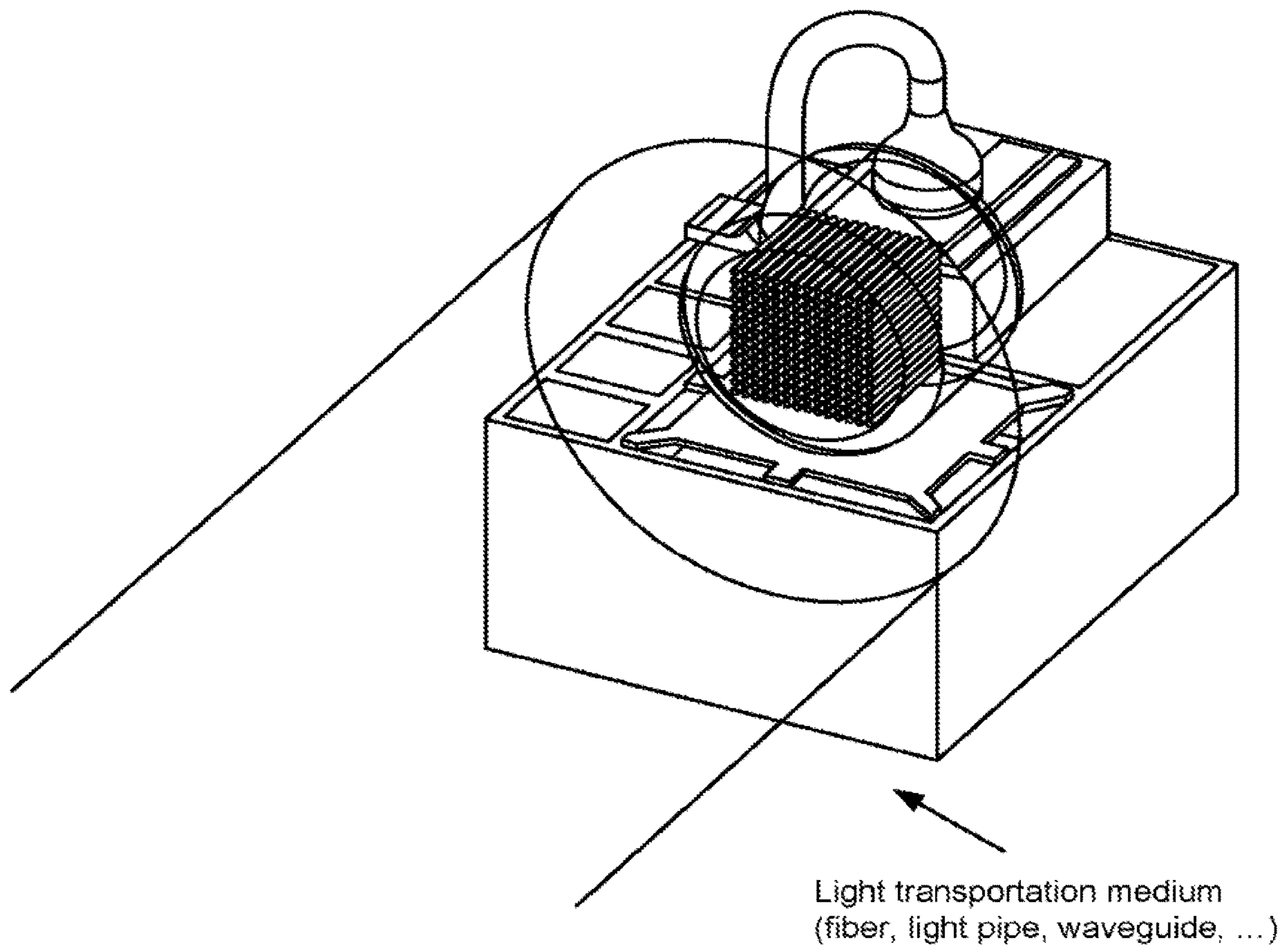
FIG. 22: Array or Module Configuration
