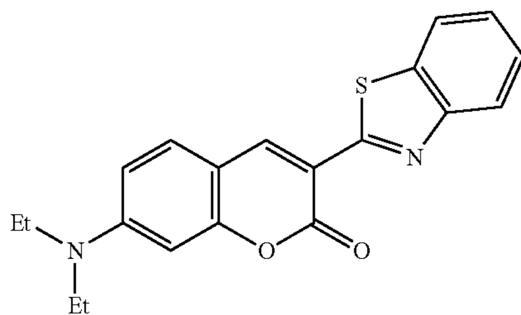
Coumarin 6
