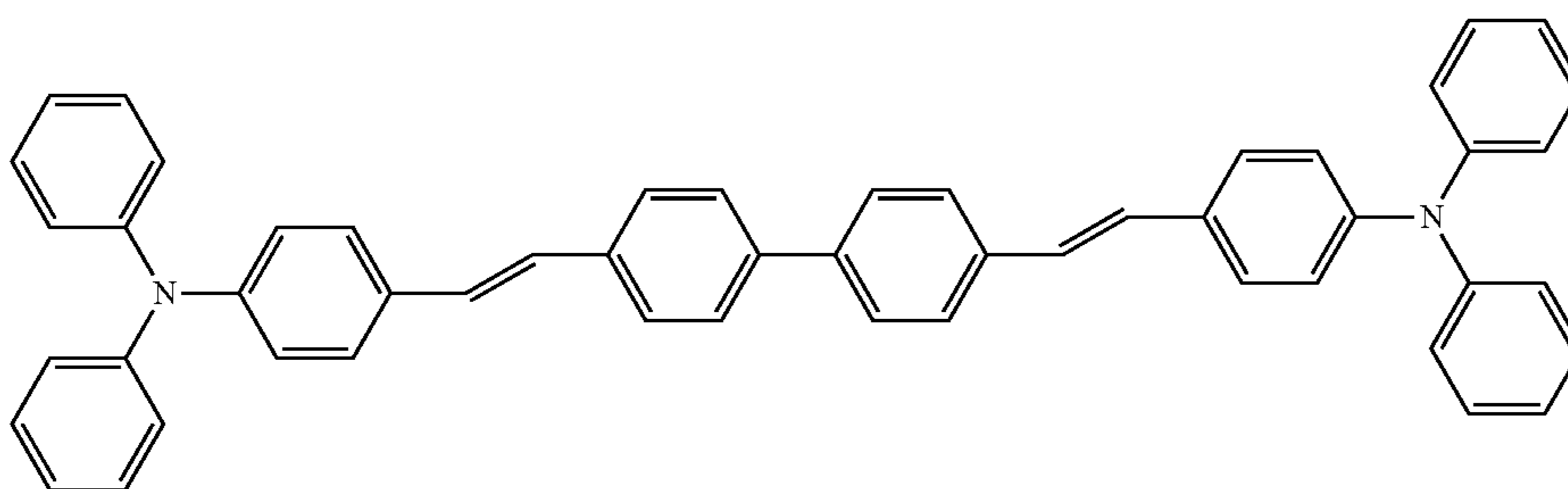
DPAVBi
