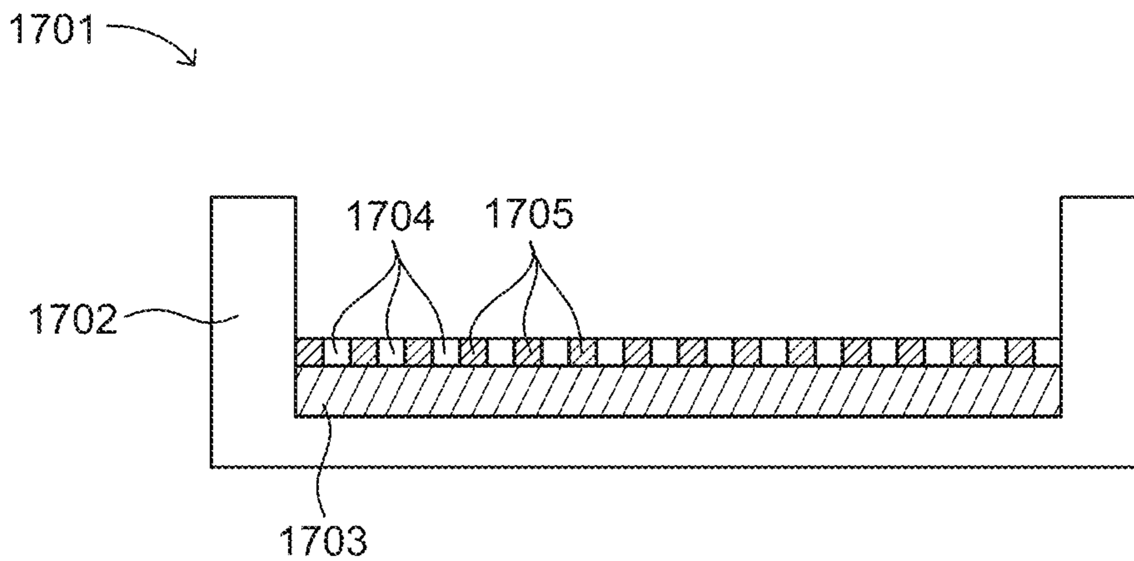
FIG. 17A
