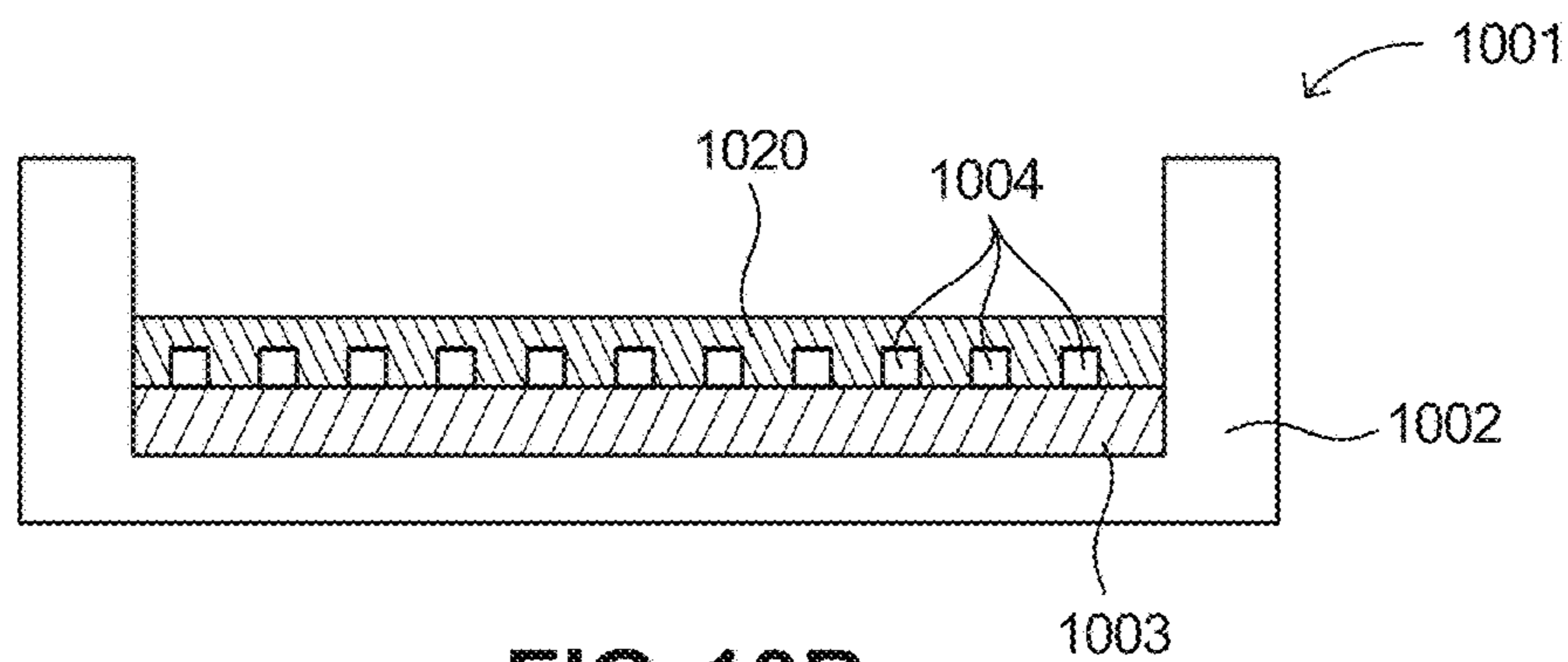
FIG. 10B
