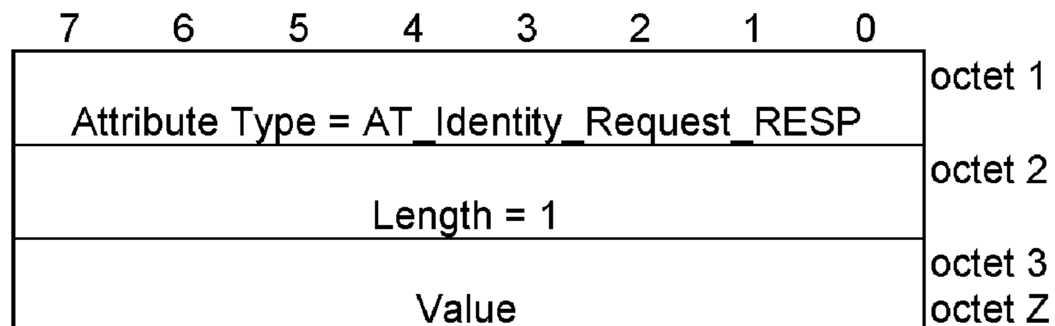
Figure 8.2.X.1-1: AT_Identity_Request attribute_RESP
