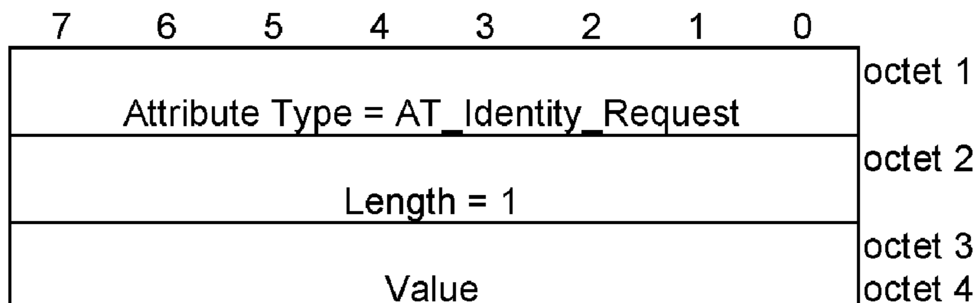
Figure 8.2.X.1-1: AT_Identity_Request attribute
