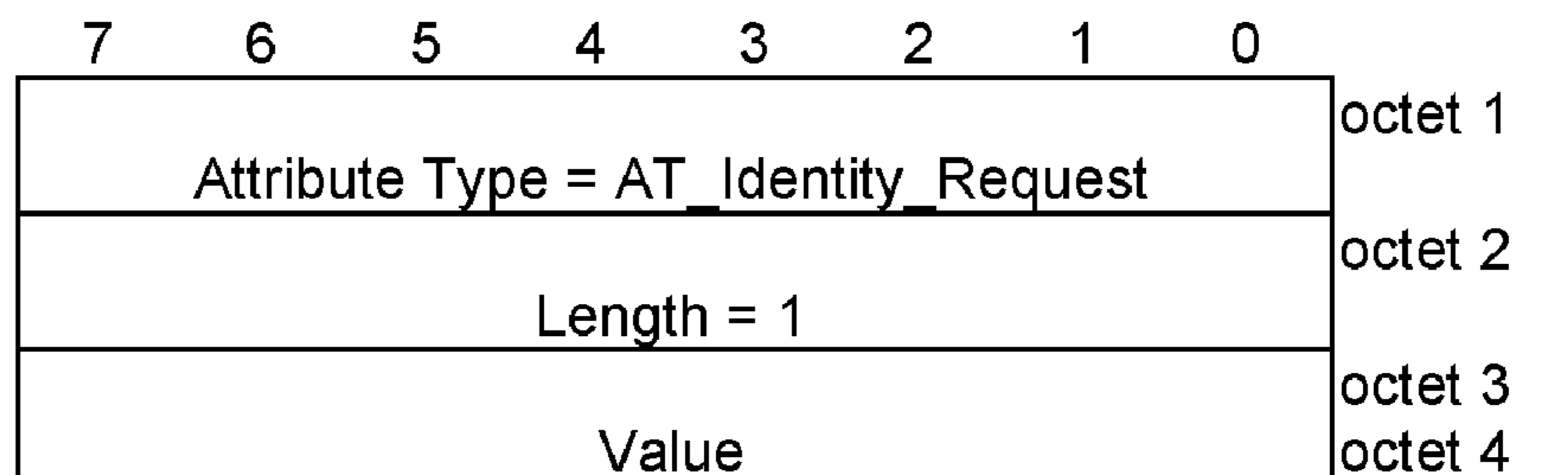
Figure 8.2.X.1-1: AT_Identity_Request attribute
