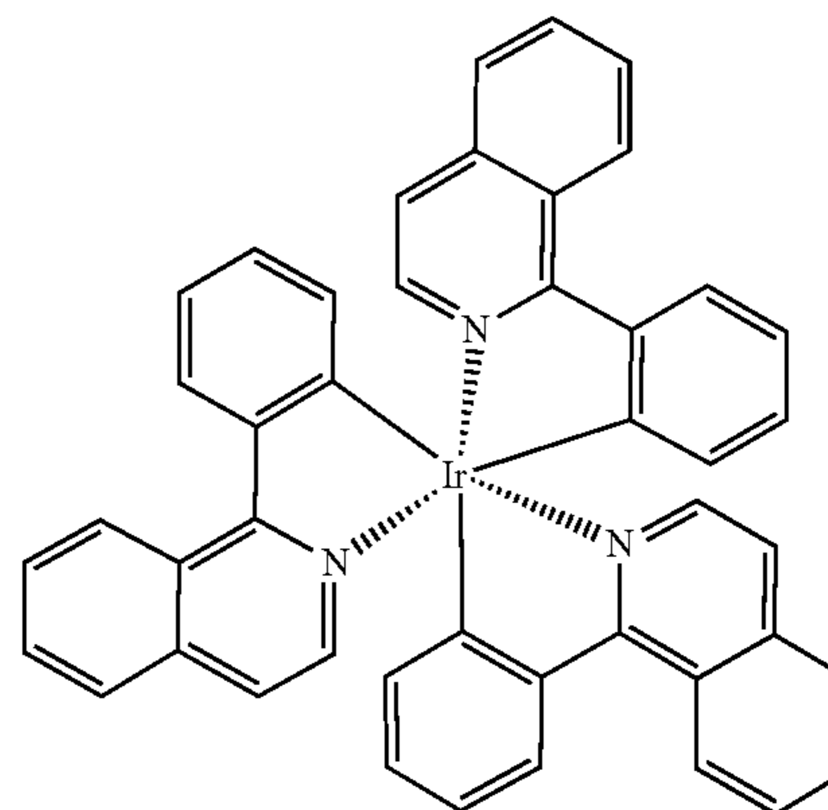
Ir(piq) 3
