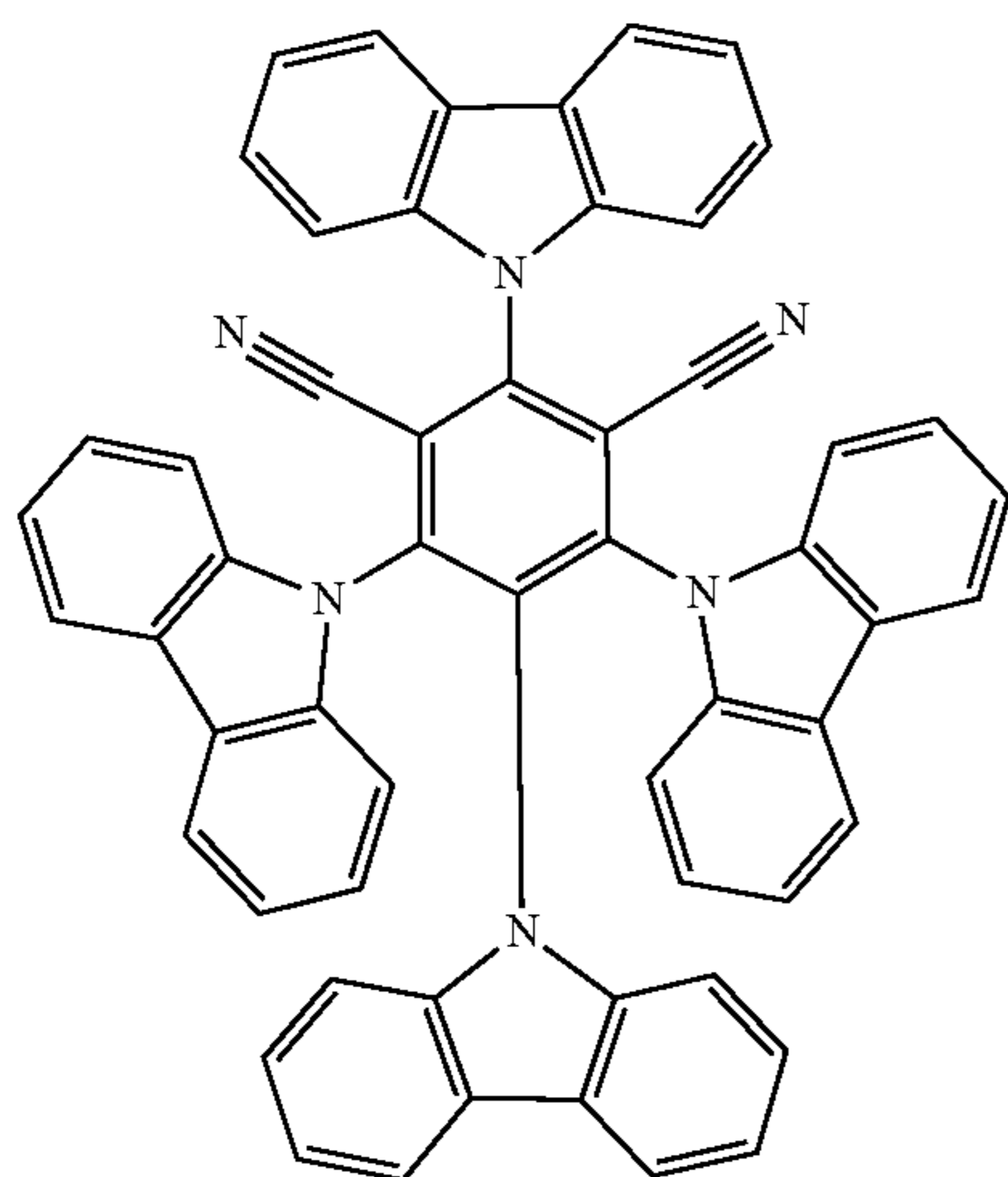
4CzIPN
