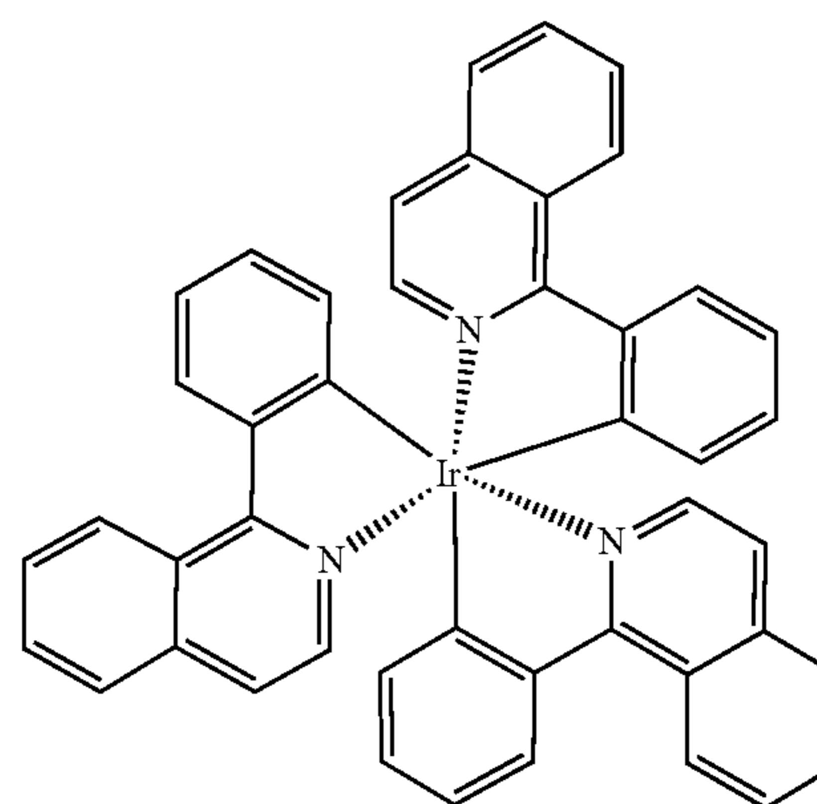
Ir(piq) 3
