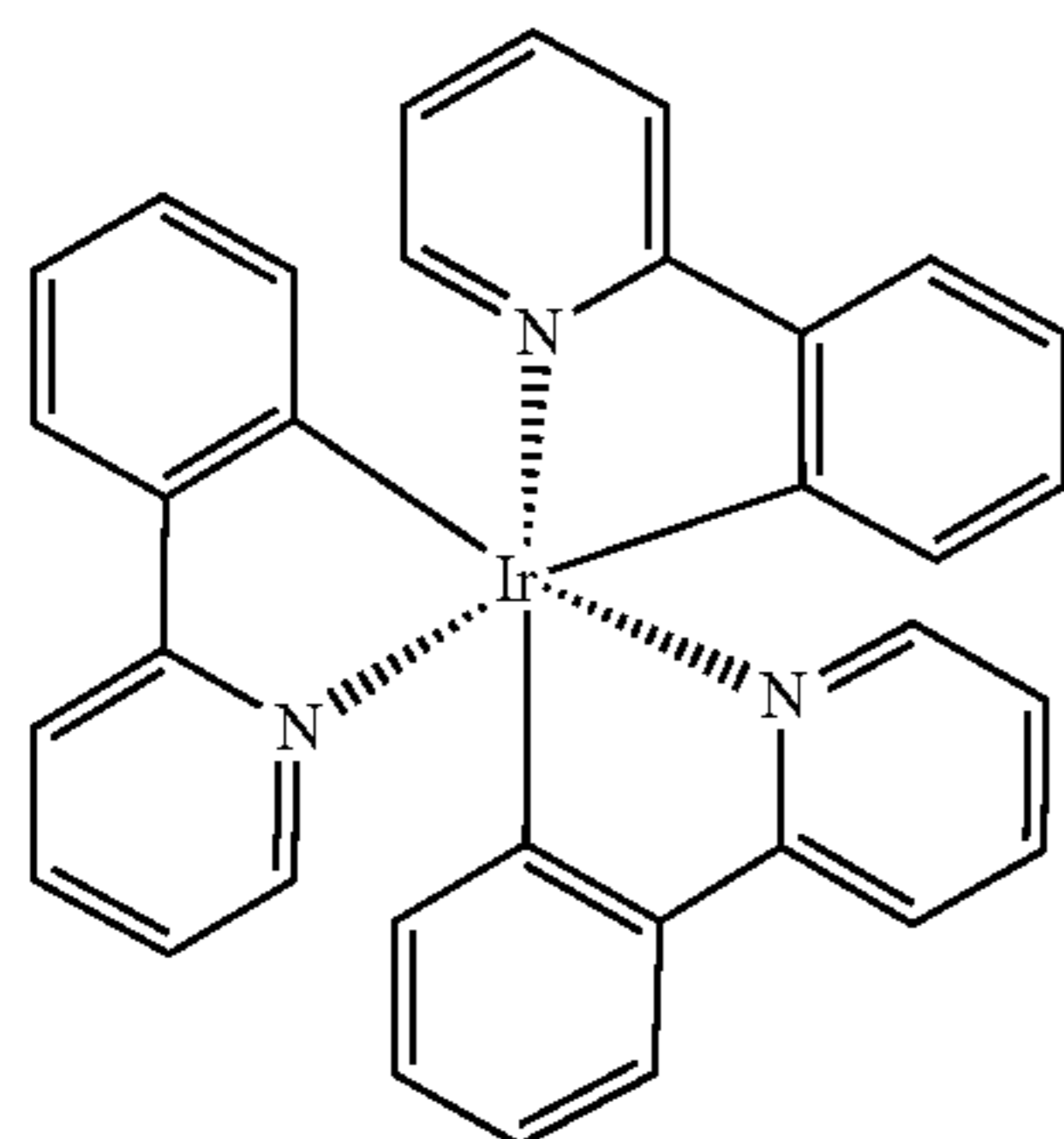
Ir(ppy) 3
