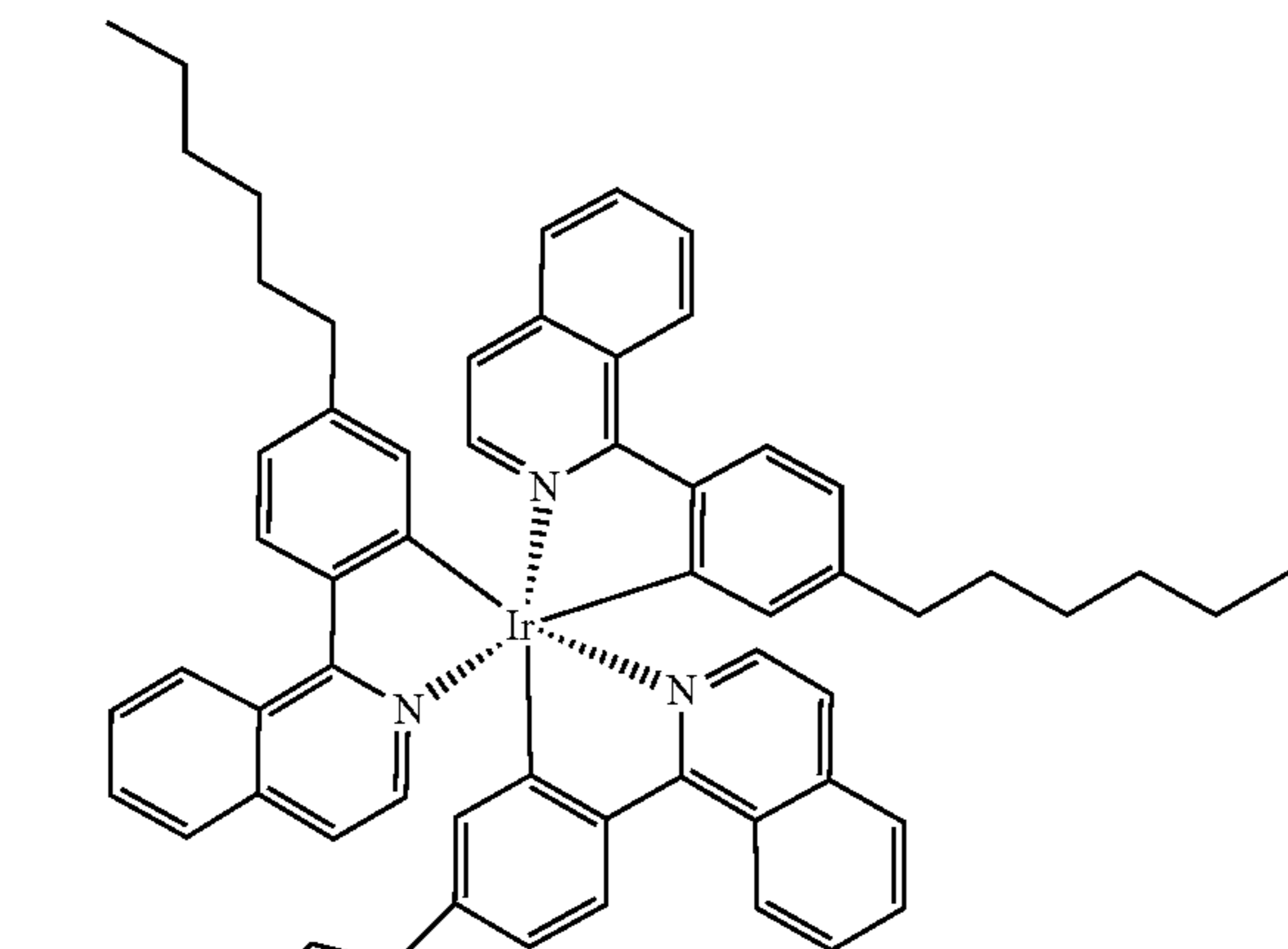
Hex-Ir(piq) 3
