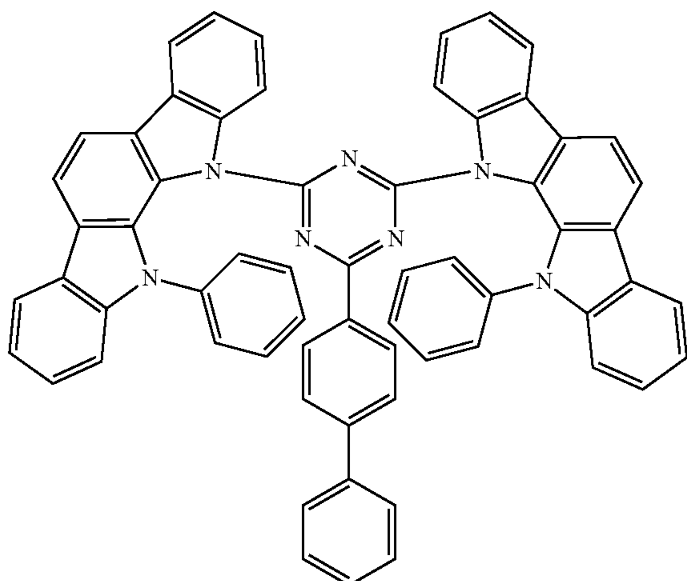
PIC-TRZ
