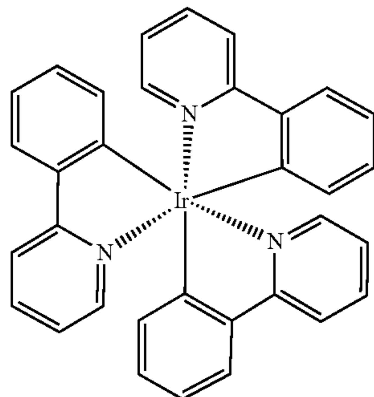
Ir(ppy) 3
