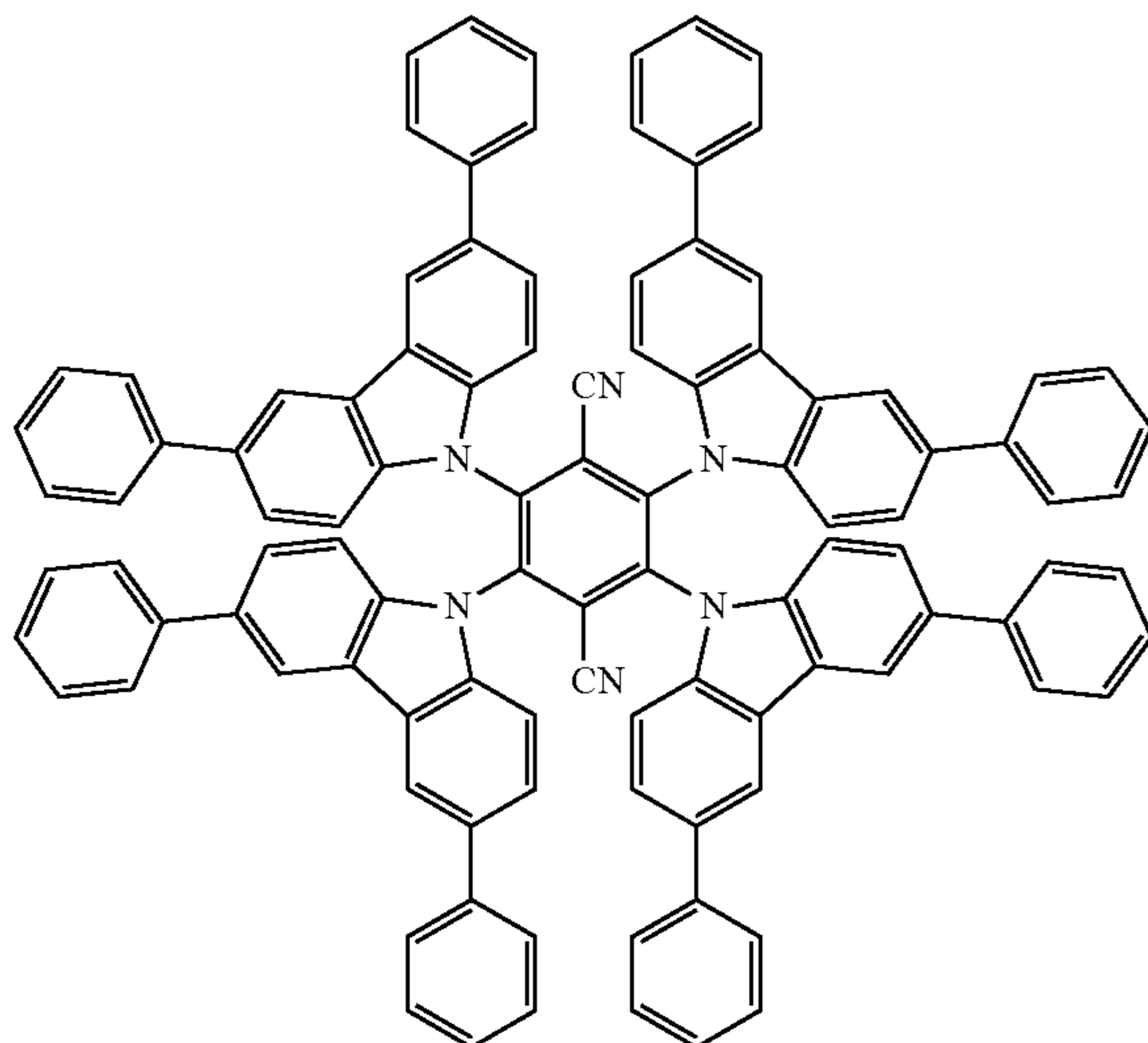
4Cz-TPN-Ph
