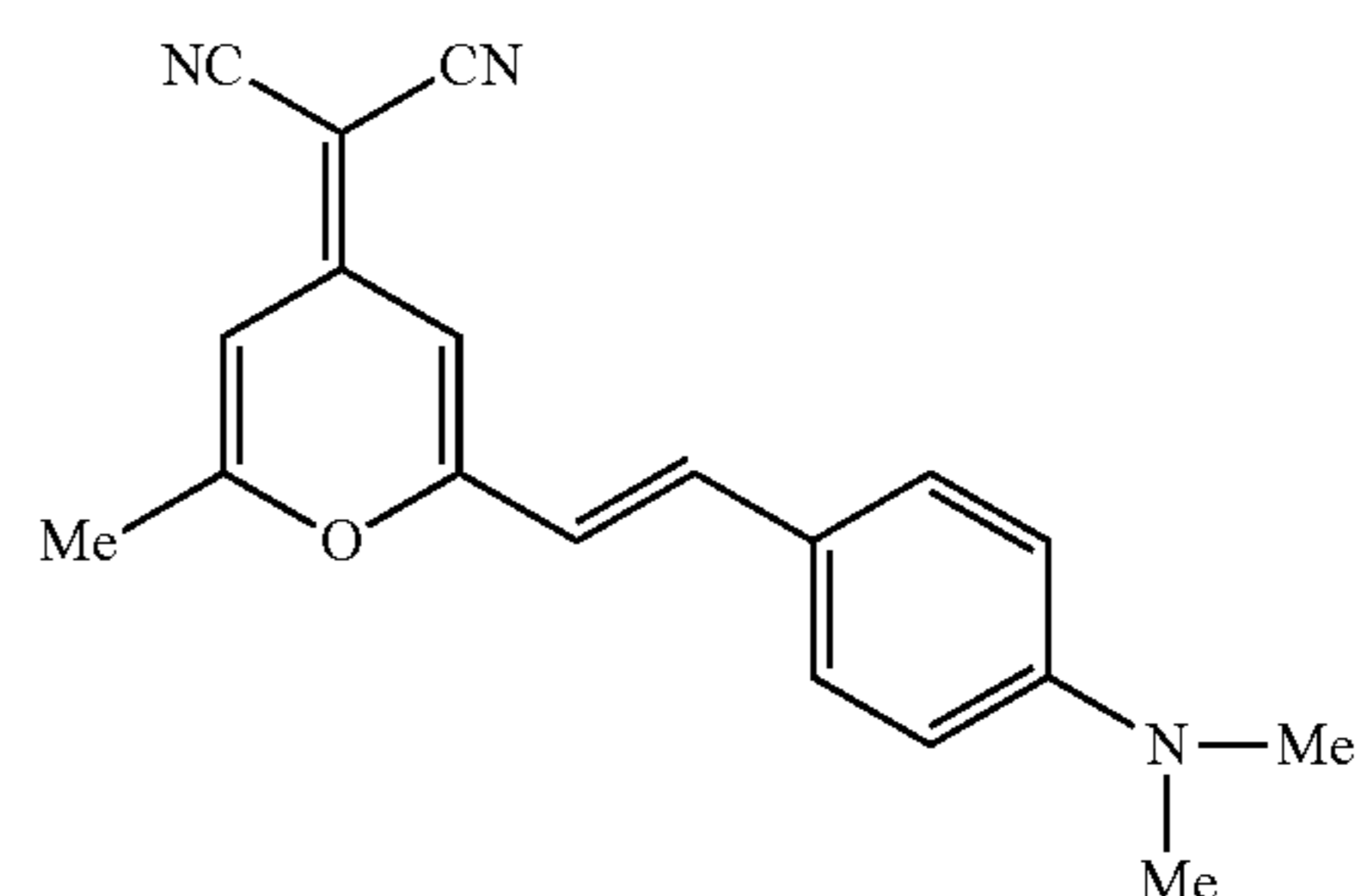
DCM
