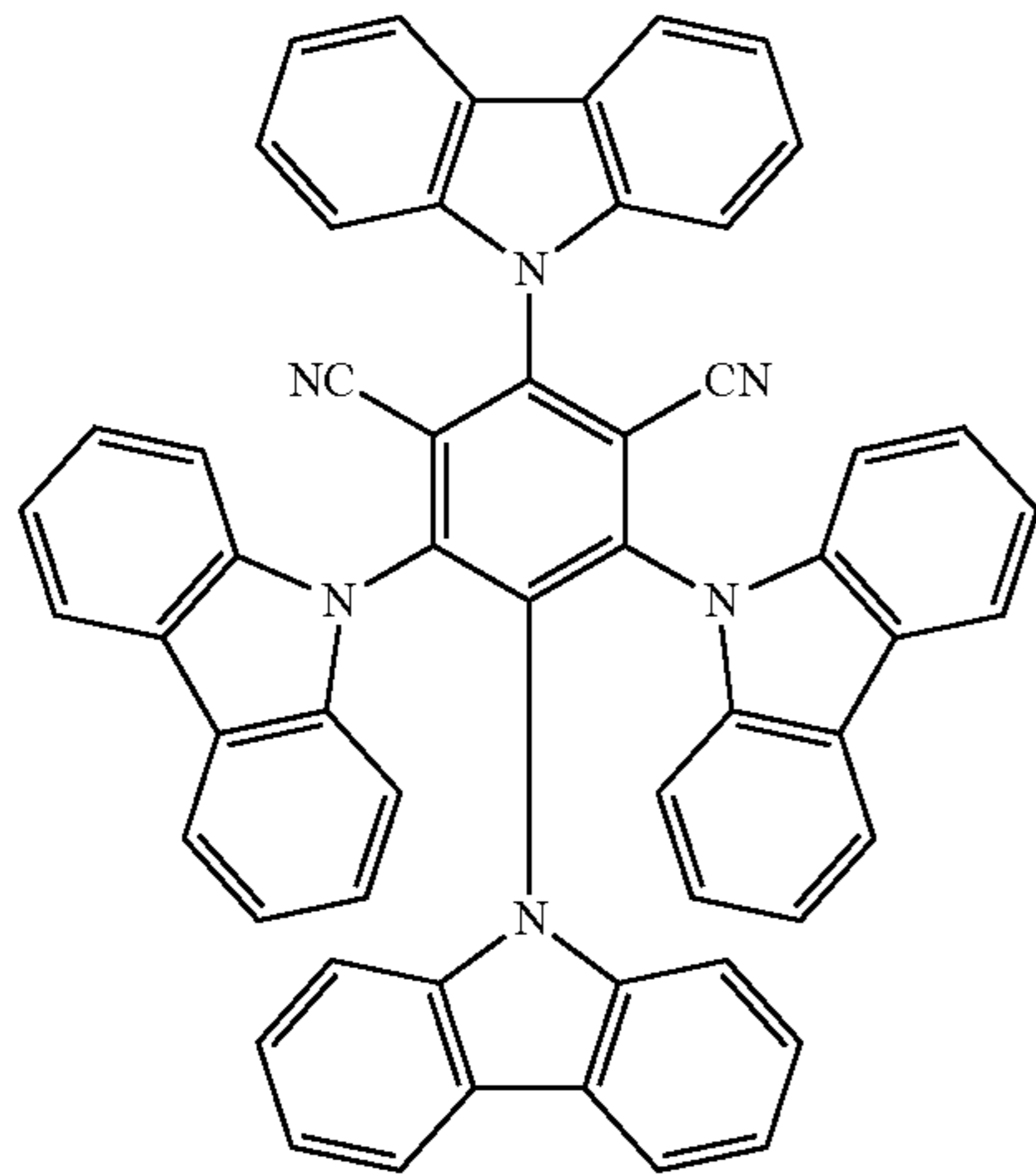
4CzIPN
