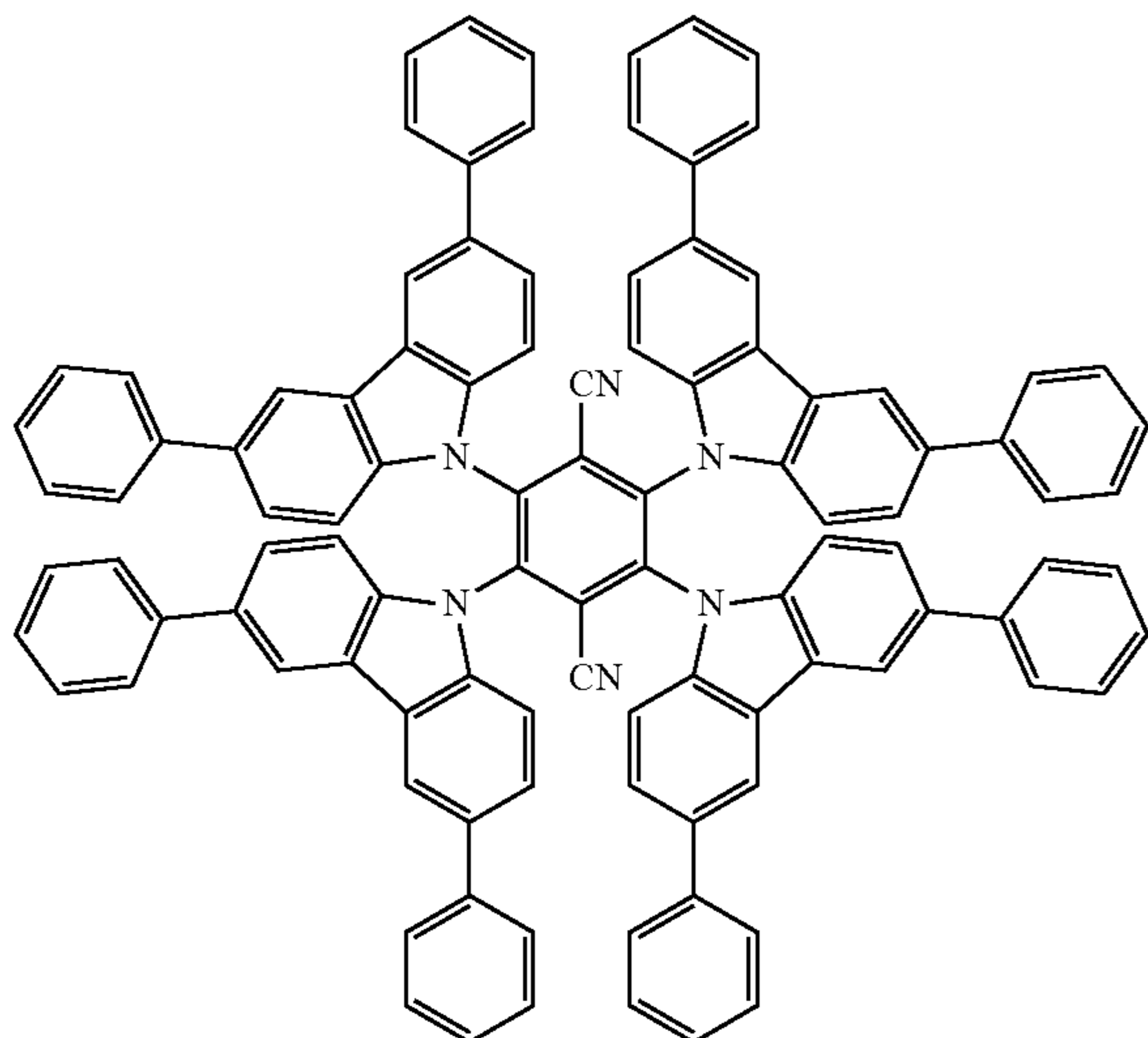
4Cz-TPN-Ph
