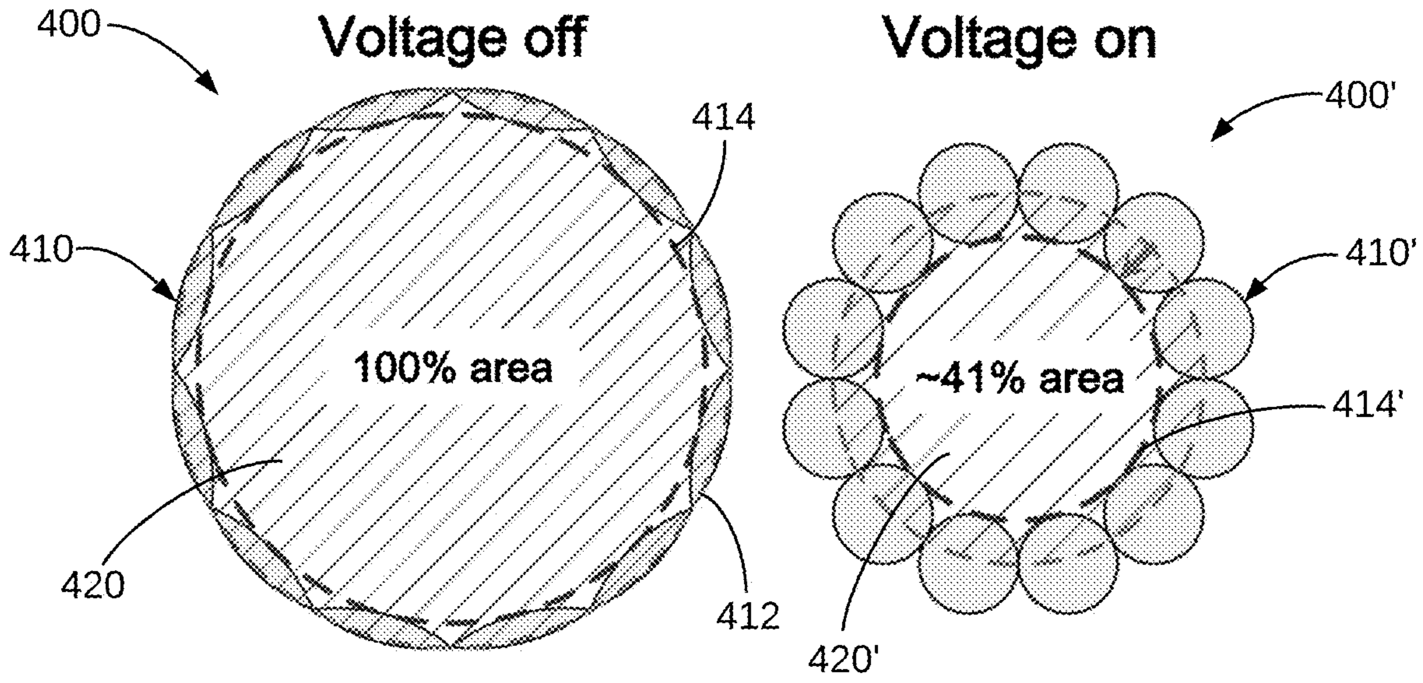
FIG. 4A
