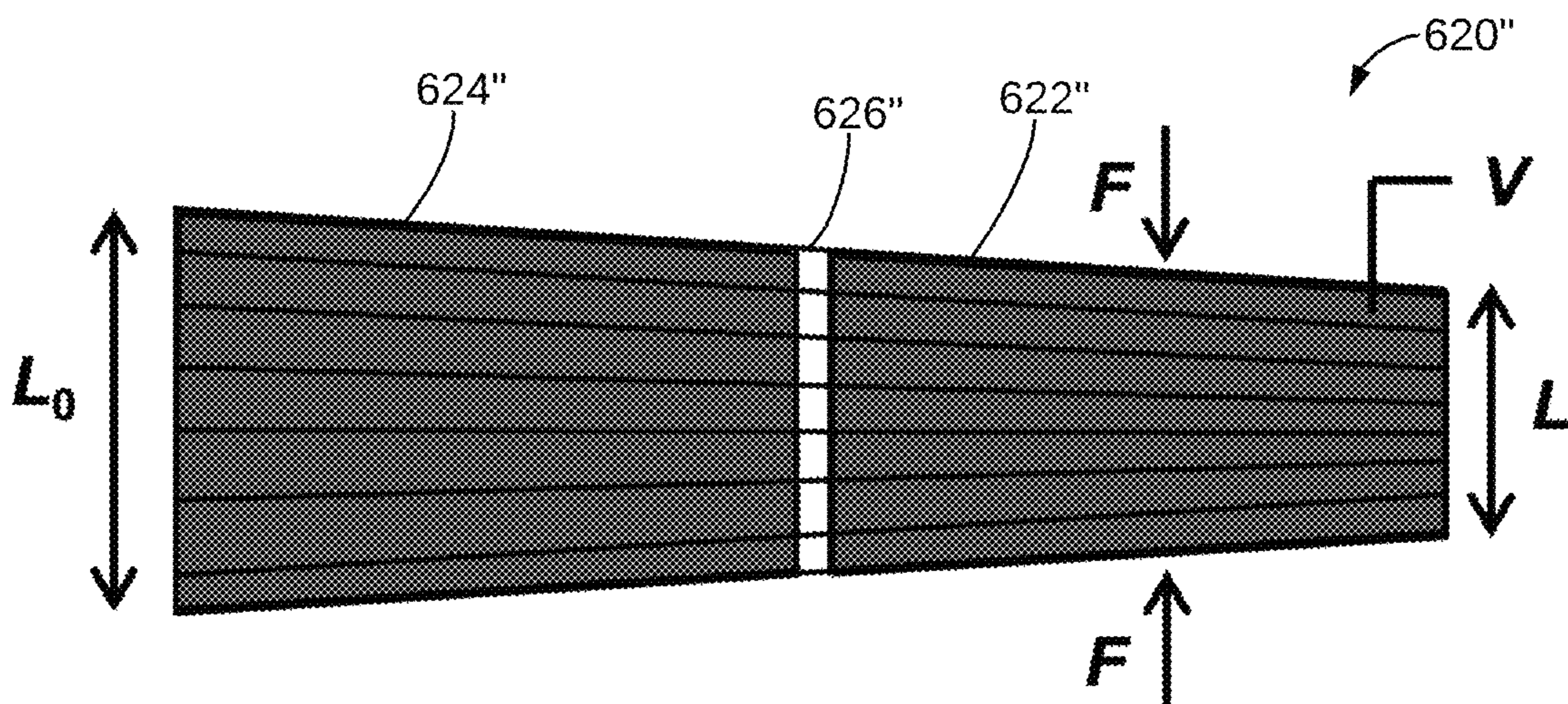
FIG. 6G
