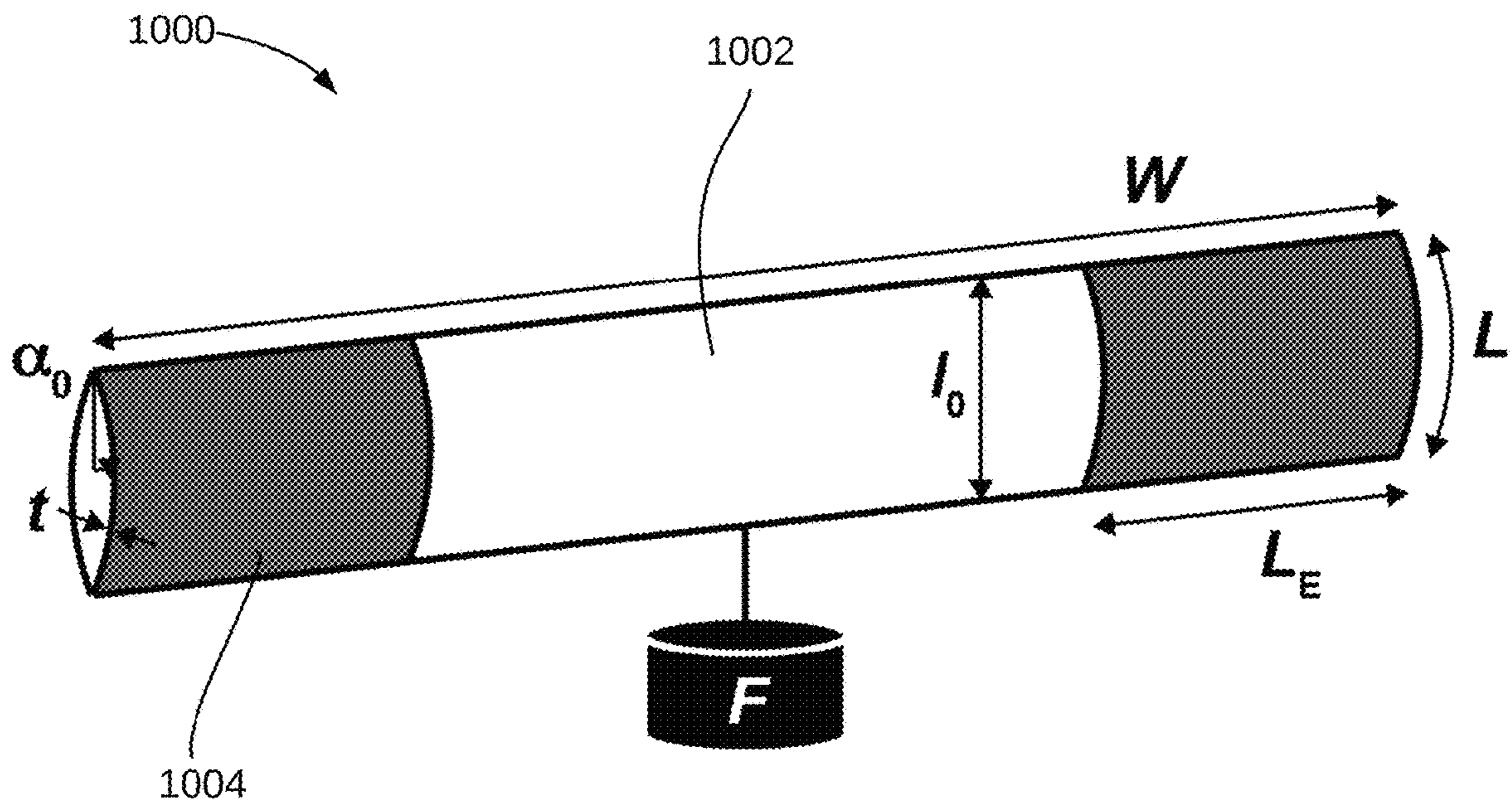
FIG. 10A
