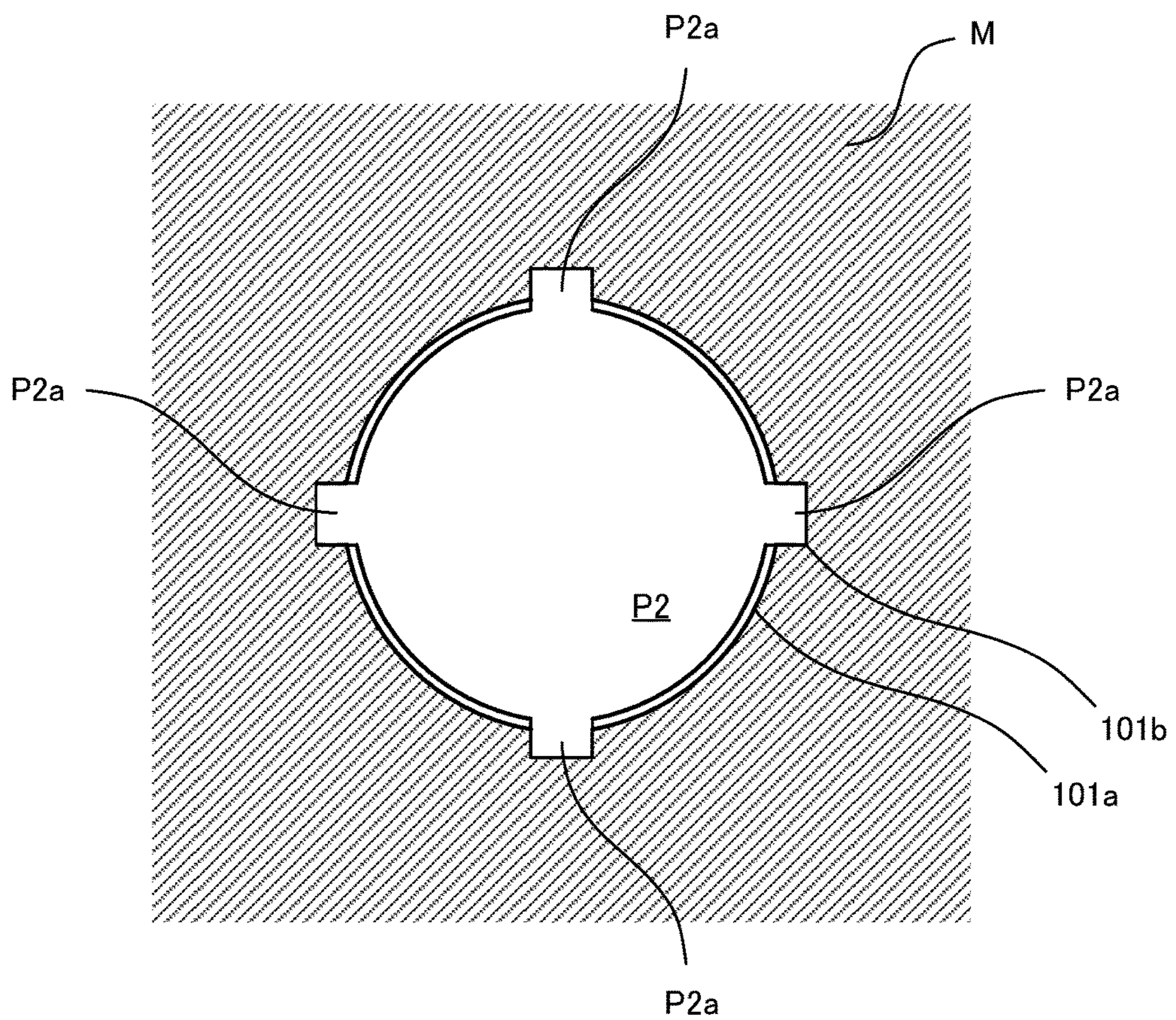
FIG.10B
