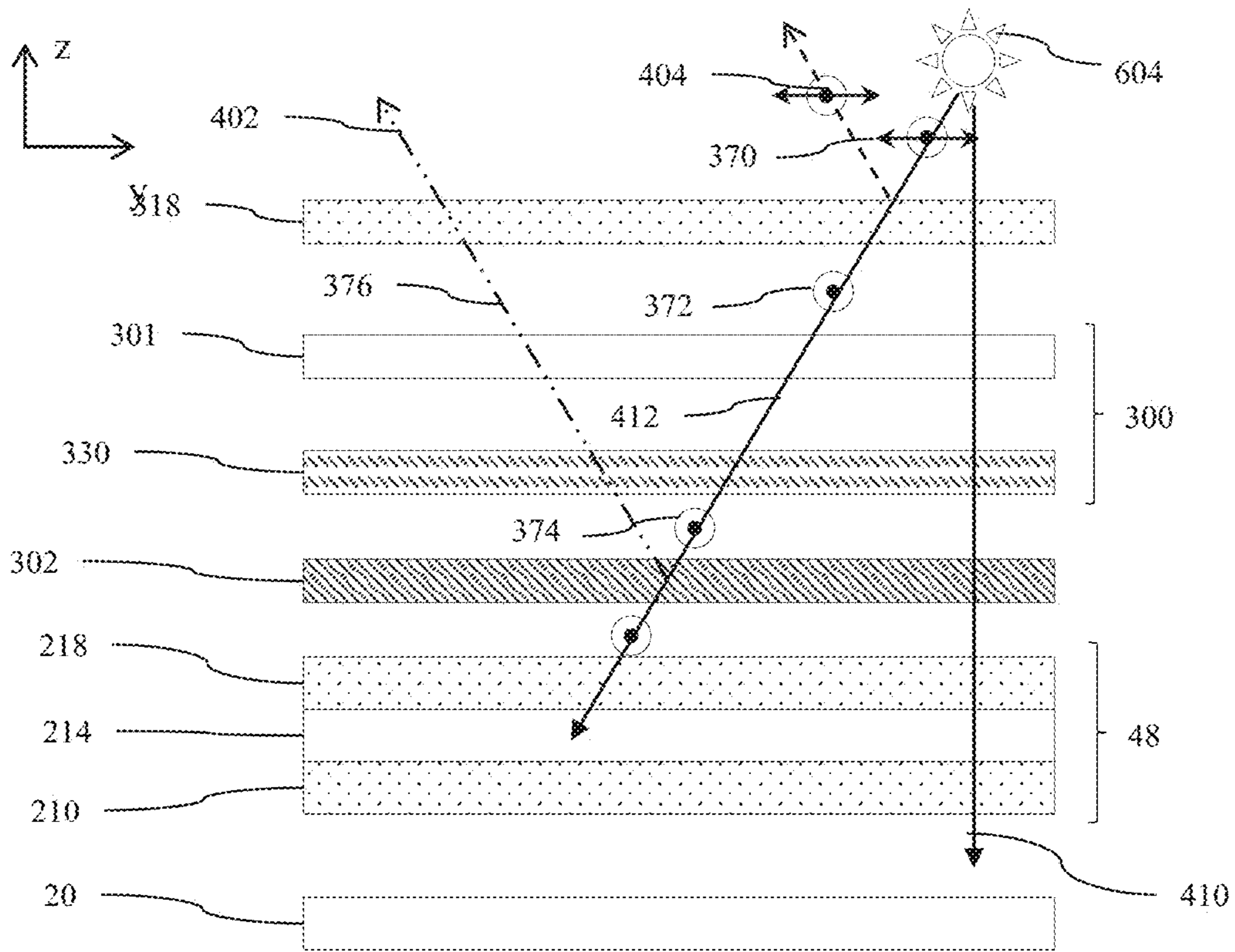
FIG. 9D Reflectivity
