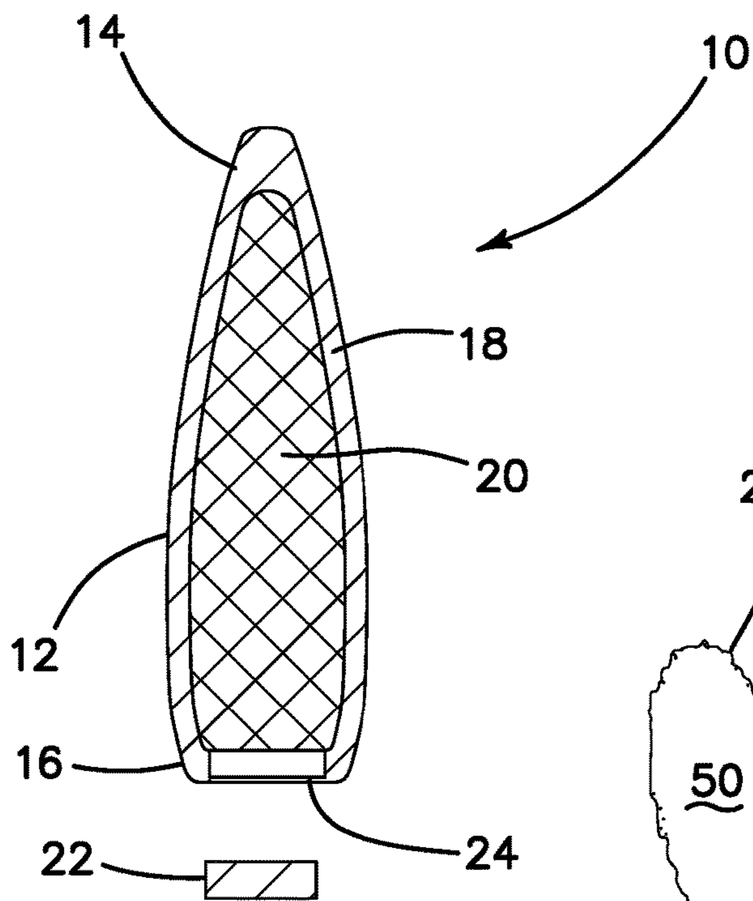
FIG. 1A
