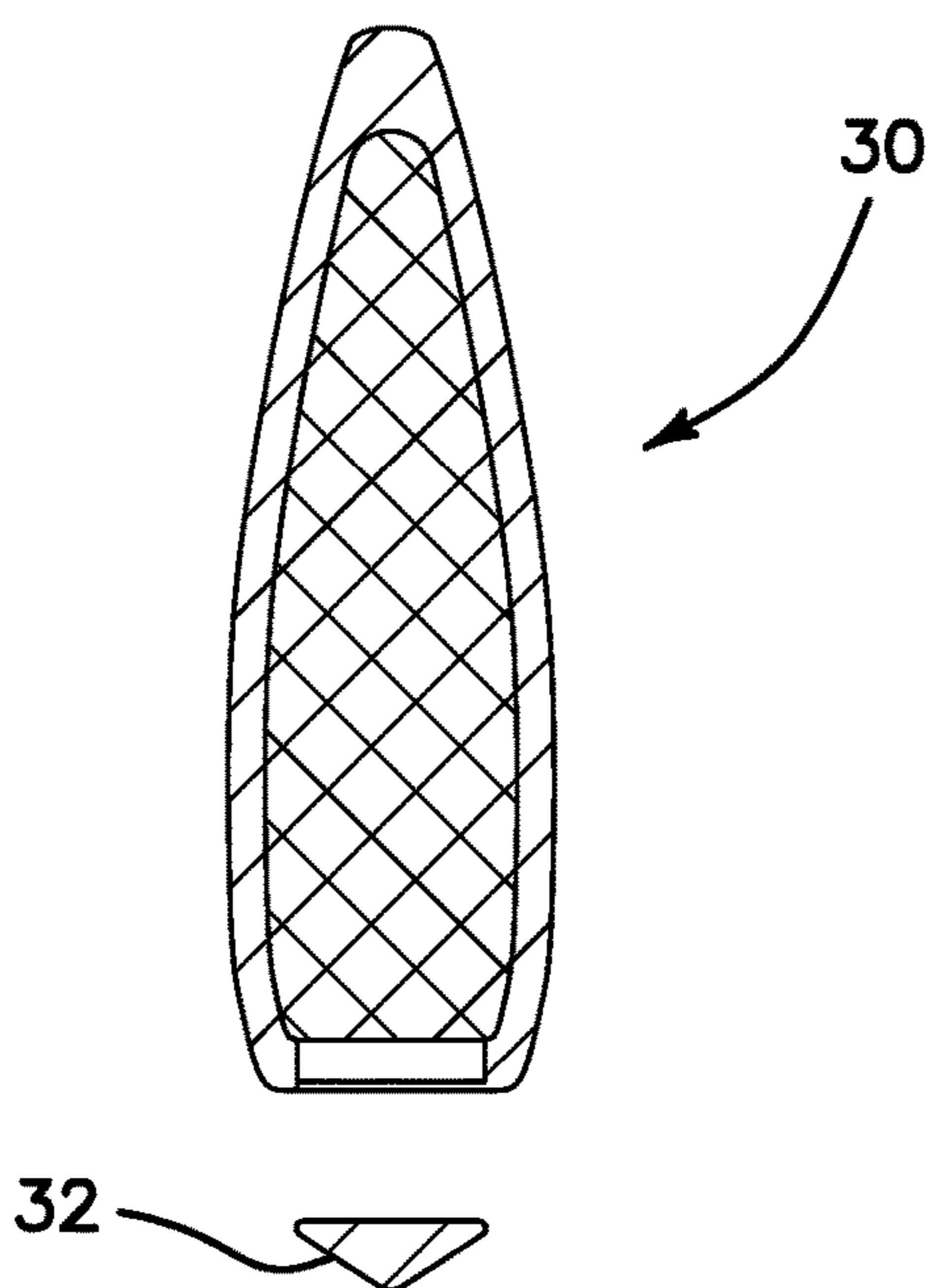
FIG. 2A
