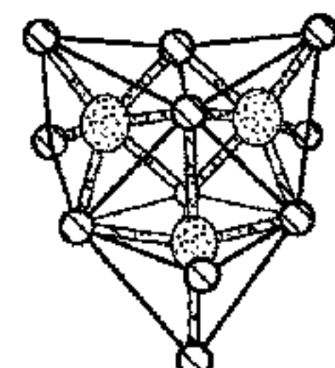
Trimer
