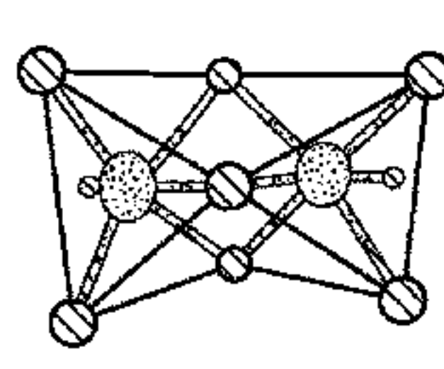
Dimer
