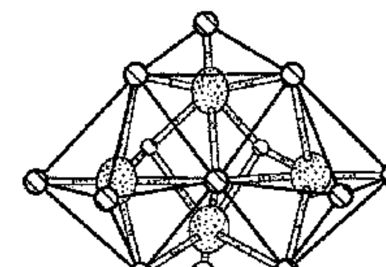
Tetramer
