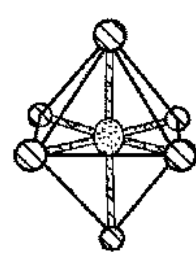
Monomer
